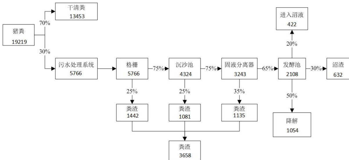
图 3.2-2 猪粪、粪渣、沼渣平衡图 (单位: t/a)
