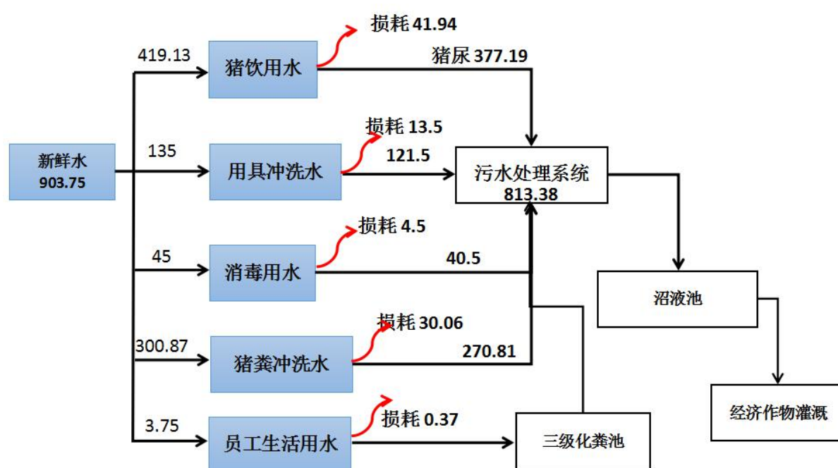
图 3.2-1 项目日水平衡图 (单位 t/d)
