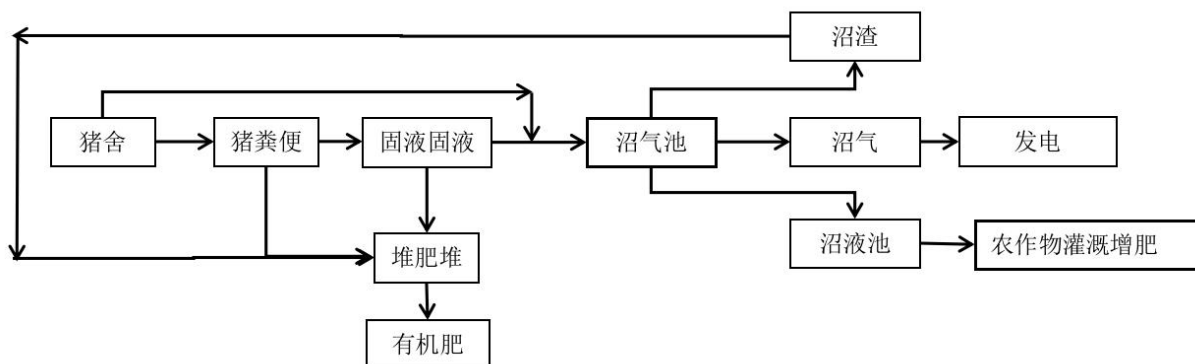
图 3.2-4 污水处理系统工艺流程示意图
