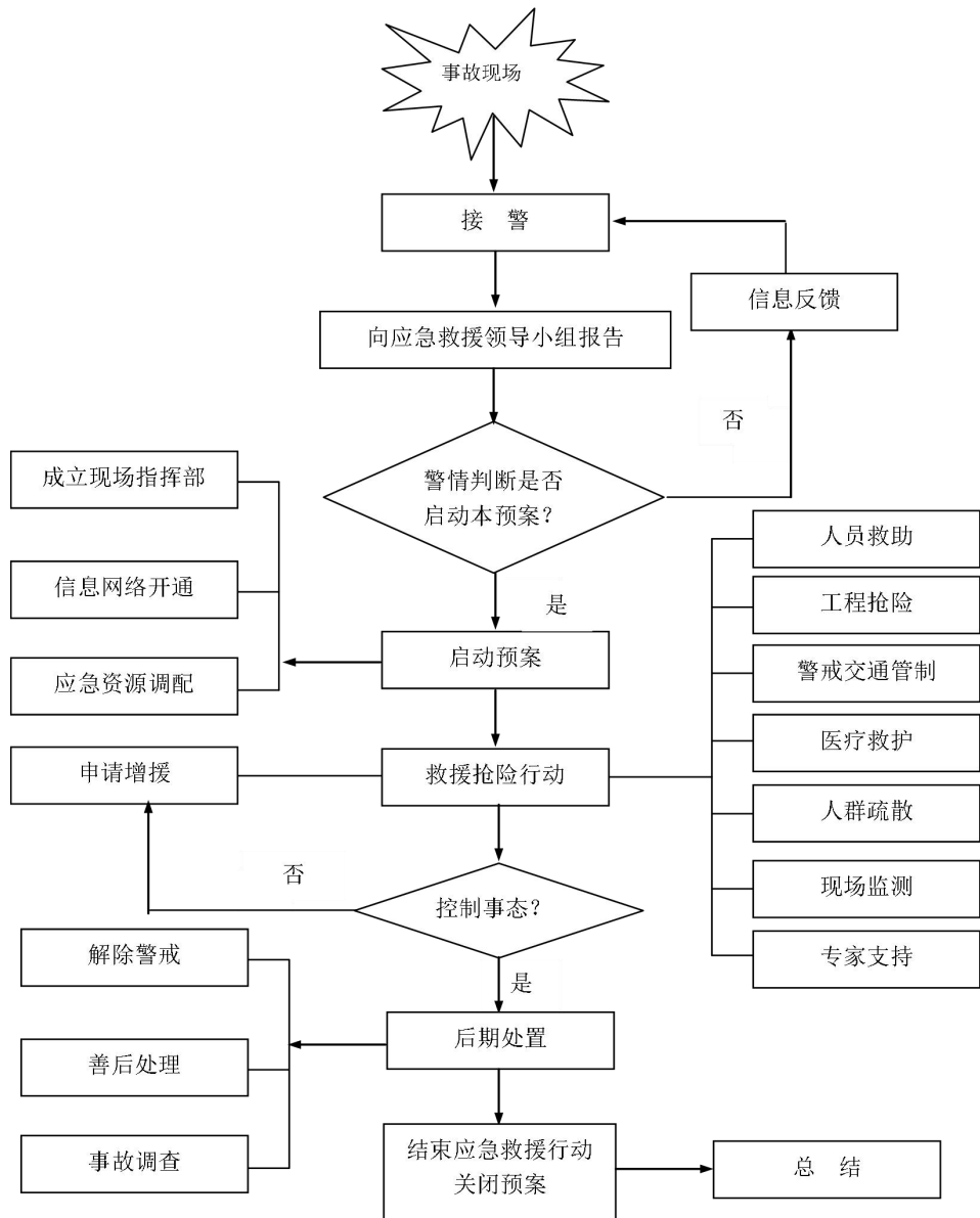
图 8.5-1 报警与响应流程图
