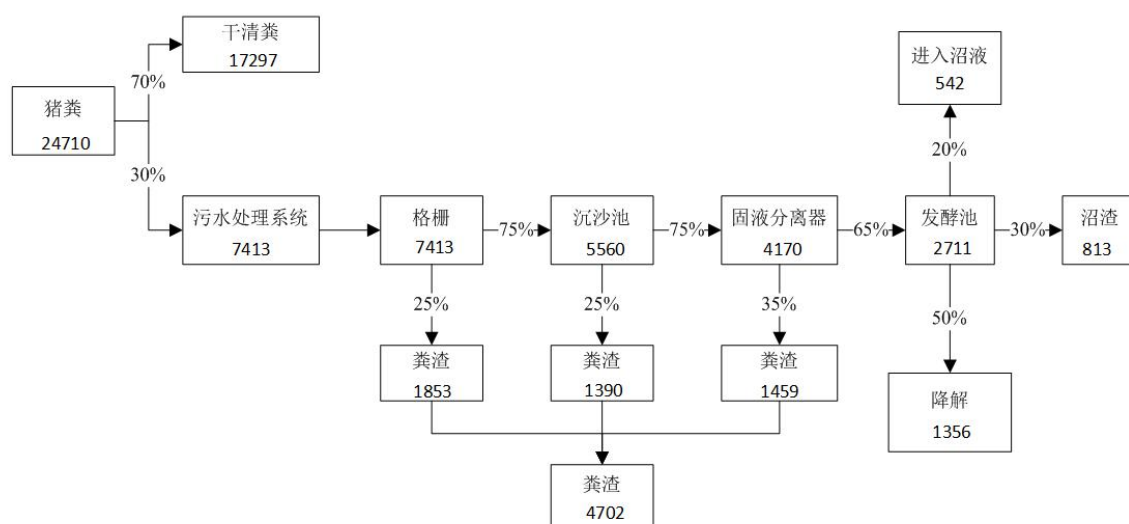
图 3.2-2 猪粪、粪渣、沼渣平衡图 (单位: t/a)
