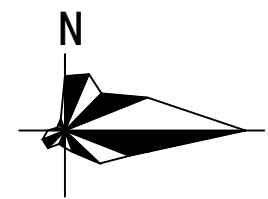
风玫瑰图
