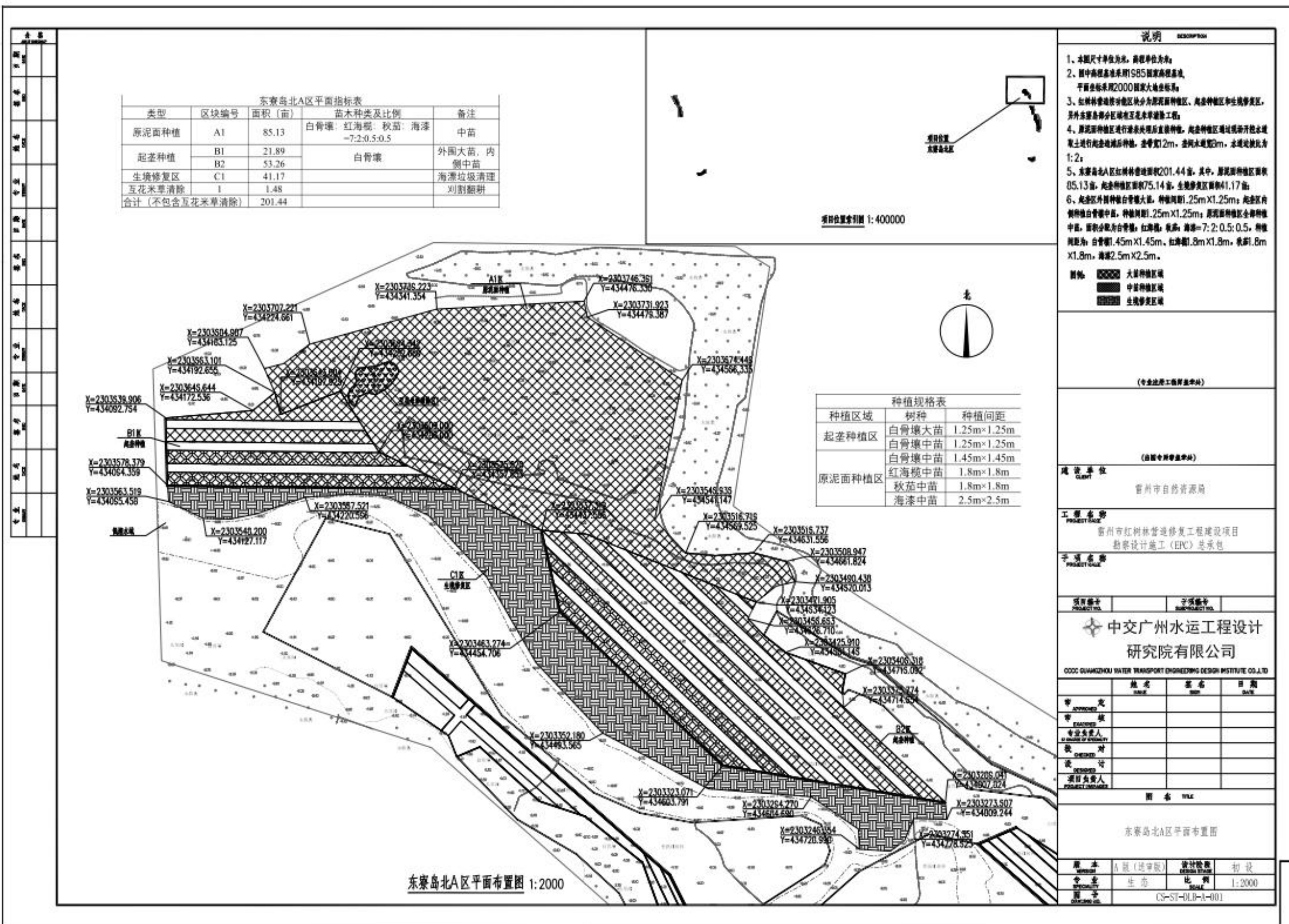
附图 2 (1) 东里镇北 A 区平面布置图
