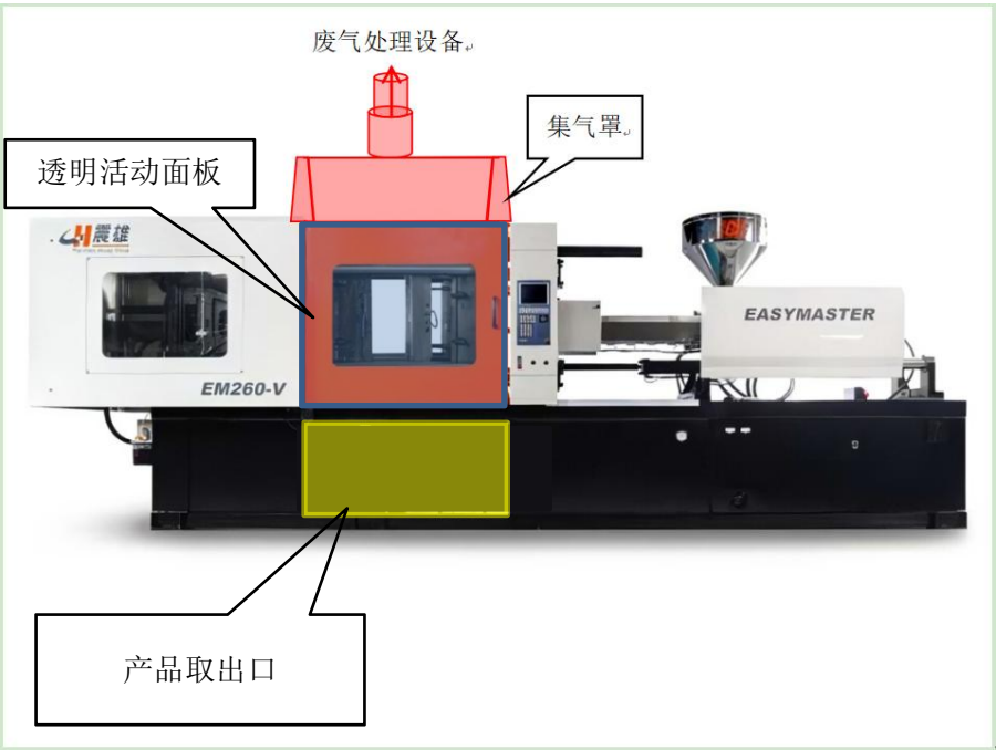
图4-3 注塑废气集气罩设置情况
