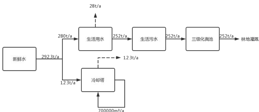
图 2-8 项目用水平衡表
