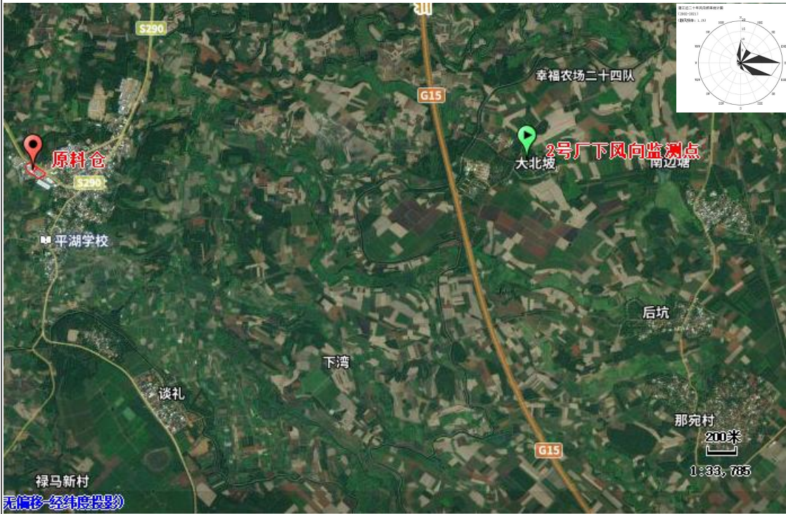
图 3-1 项目大气特征污染物现状监测示意图
