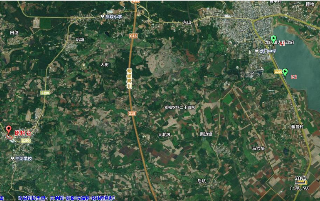
图 3-2 项目引用水环境现状监测示意图
