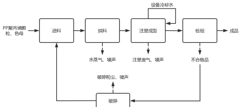
图2-9 项目生产工艺流程图
