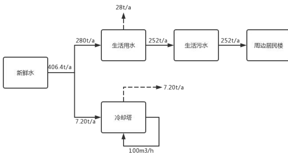
图 2-8 项目用水平衡表
