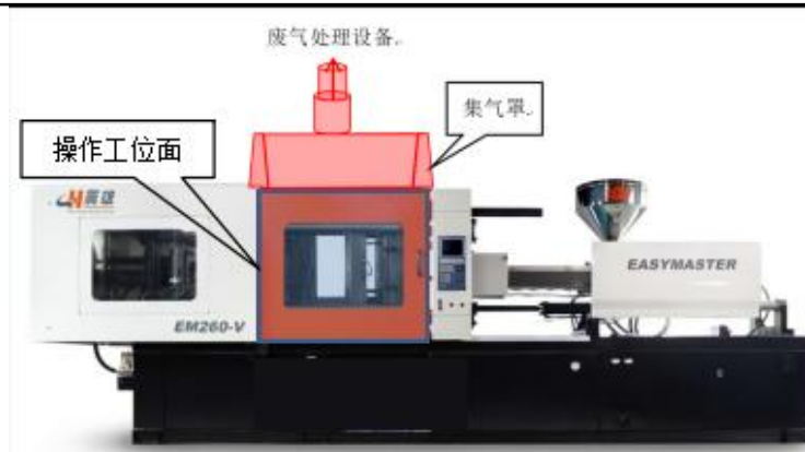
图 4-4 注塑废气集气罩设置情况
