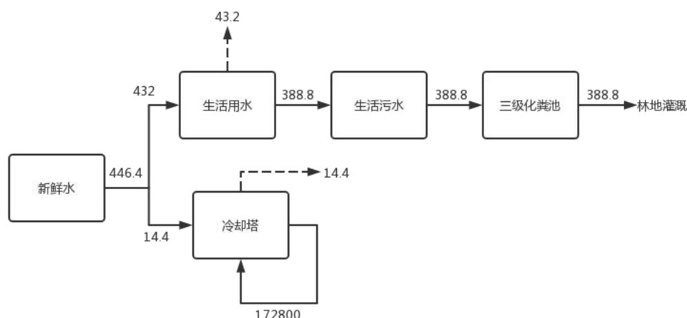
图 2-5 项目用水平衡表
