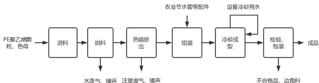
图 2-7 项目农业节水管生产工艺流程及产污环节图
