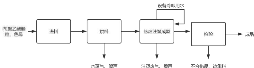
图2-6 项目农业节水管配件生产工艺流程及产污环节图
