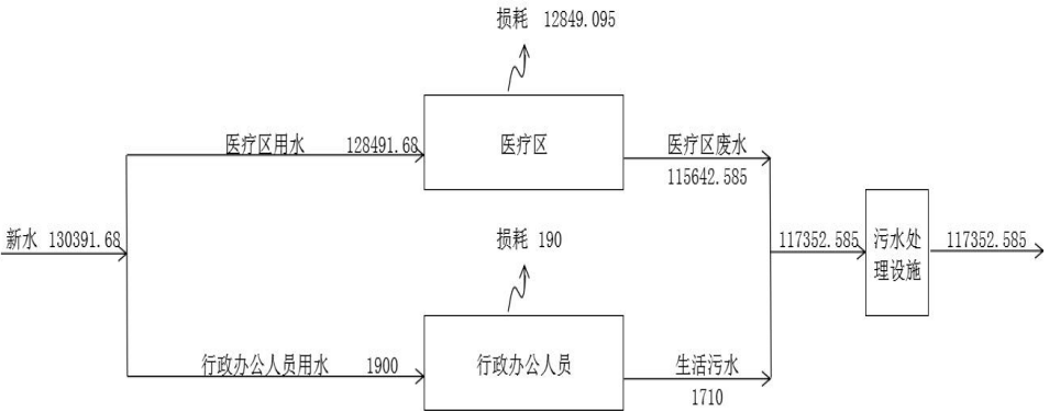
图 4-1 项目水平衡图（单位：m³/a）
