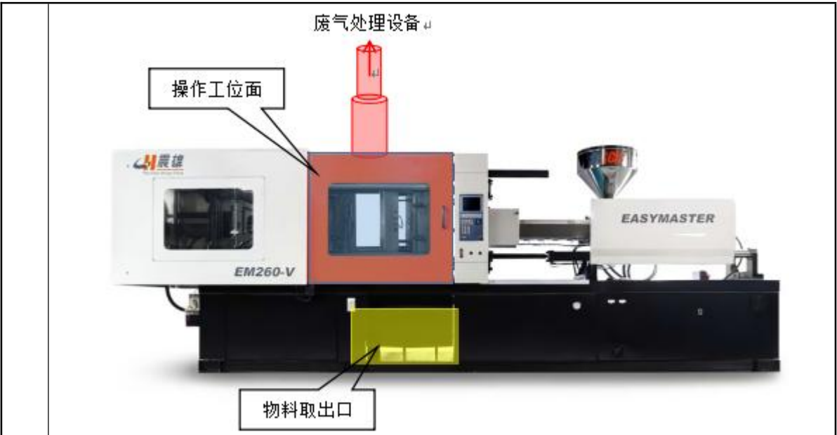
图 4-2.2 热熔机废气集气罩设置情况
