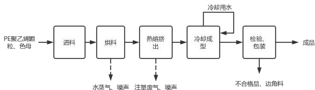
图 2-7 主管带生产工艺流程及产污环节图
