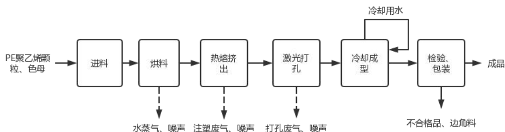
图 2-7 喷灌管带生产工艺流程及产污环节图
