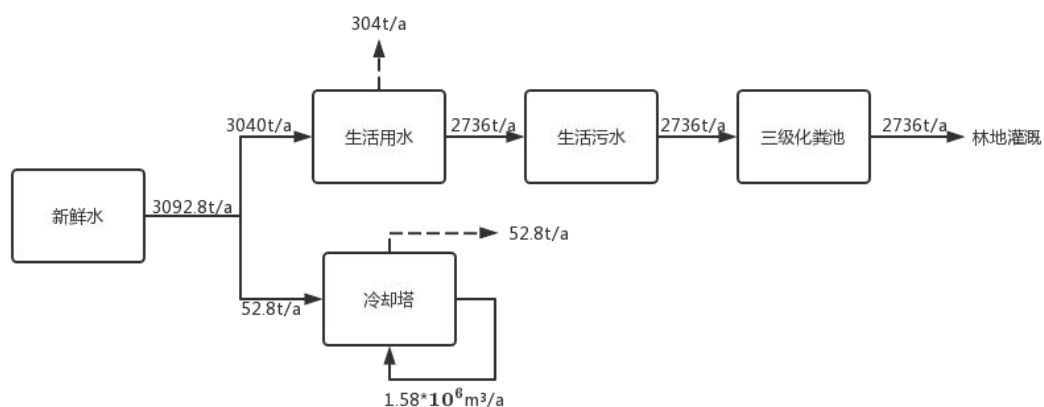
图 2-6 项目用水平衡表
