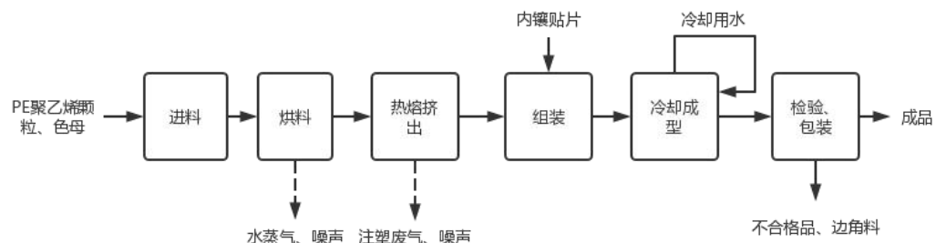
图 2-7 内镶贴片滴灌管生产工艺流程及产污环节图
