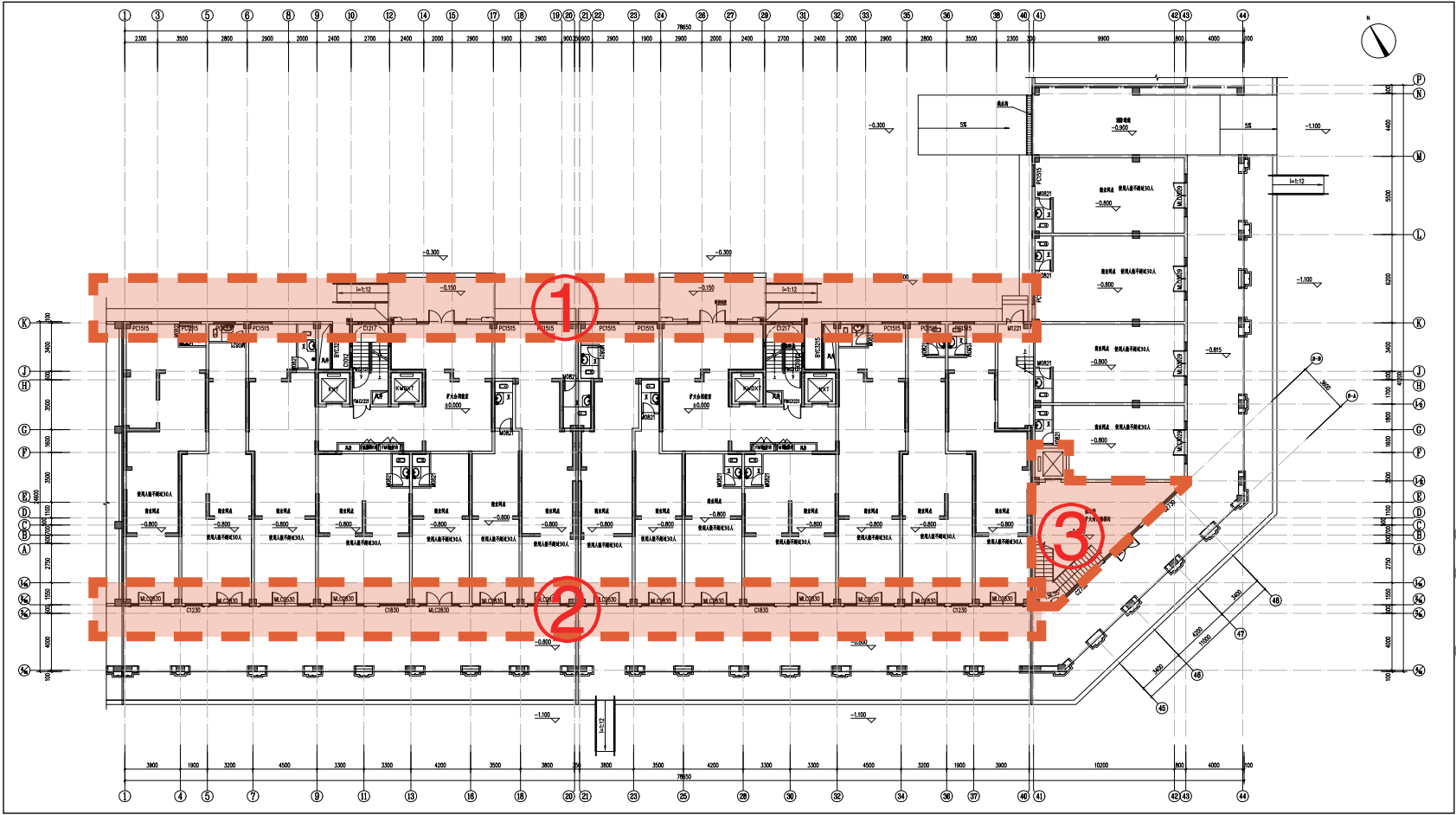
13# 调整后方案首层
