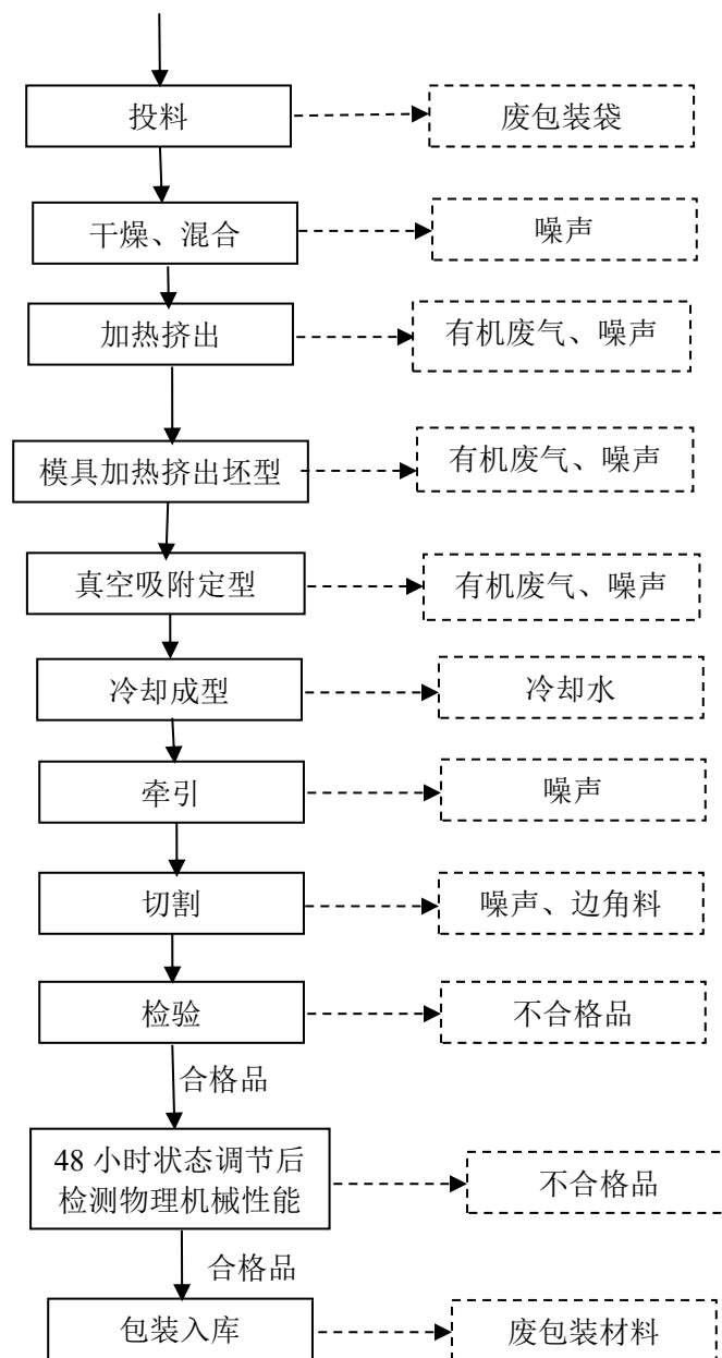
图 2-4 HDPE 给水管生产工艺流程图
