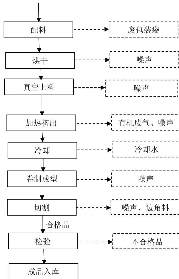
图 2-7 HDPE 内肋波纹管生产工艺流程图
