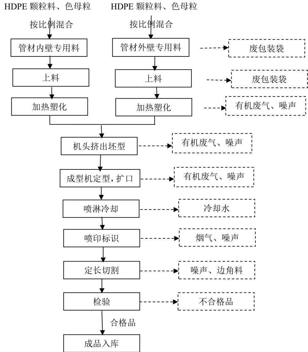
图 2-3 HDPE 双壁波纹管生产工艺流程图
