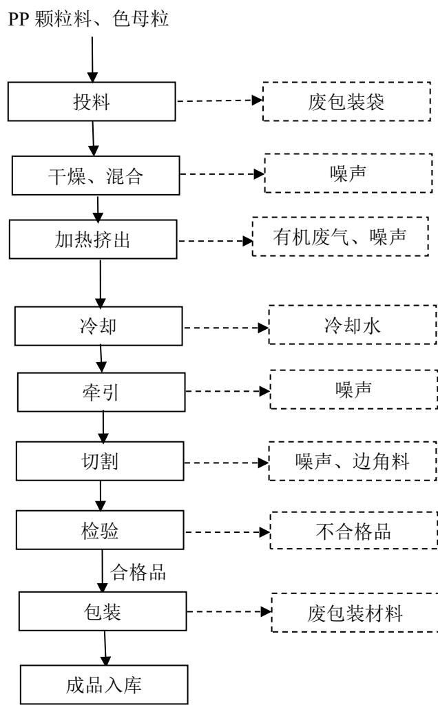
图 2-5 MPP 牵引管生产工艺流程图
