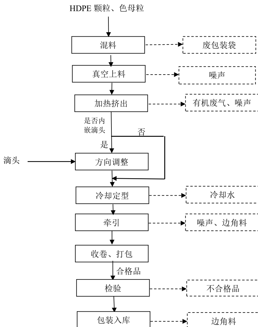
图2-8 贴片/贴条式滴灌管生产工艺流程图
