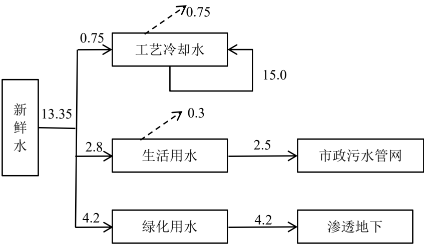
图 2-2 项目水平衡图（单位：t/d）
