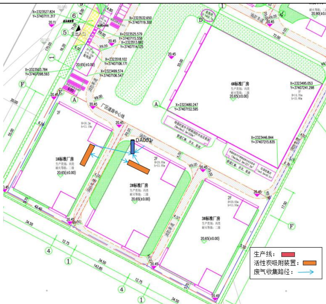
图4-3 楼顶有机废气收集图
