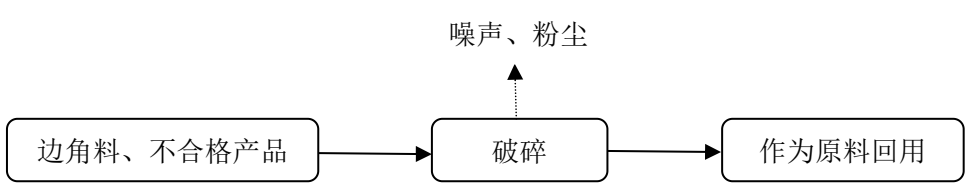
图2-10 废品回收利用工艺流程图
