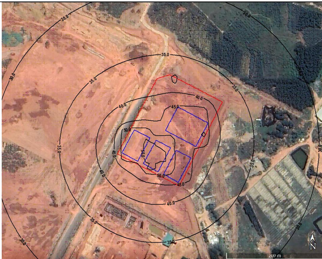
图 4-11 项目噪声贡献值等声值线图
