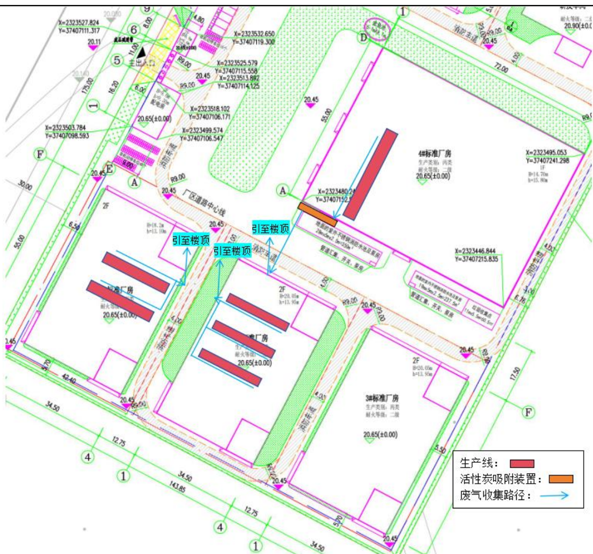
图4-1 1F有机废气收集图
