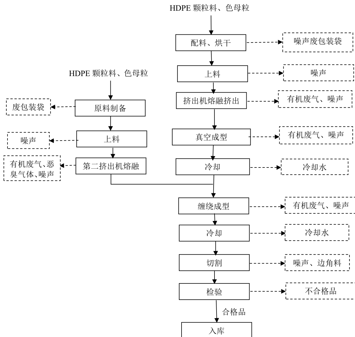
图 2-6 HDPE 中空壁缠绕管生产工艺流程图
