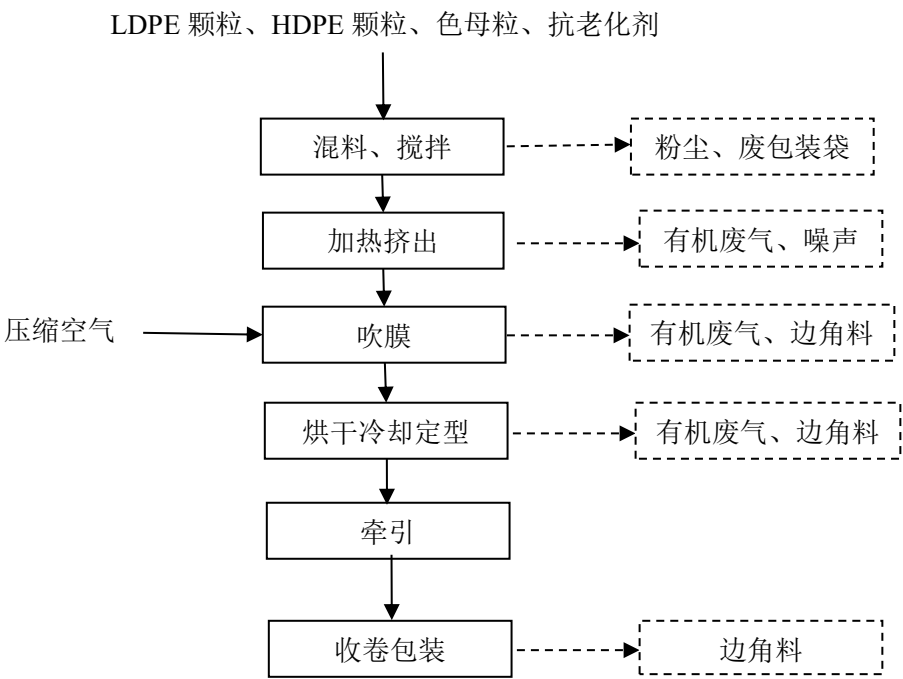
图2-9 农膜生产工艺流程图
