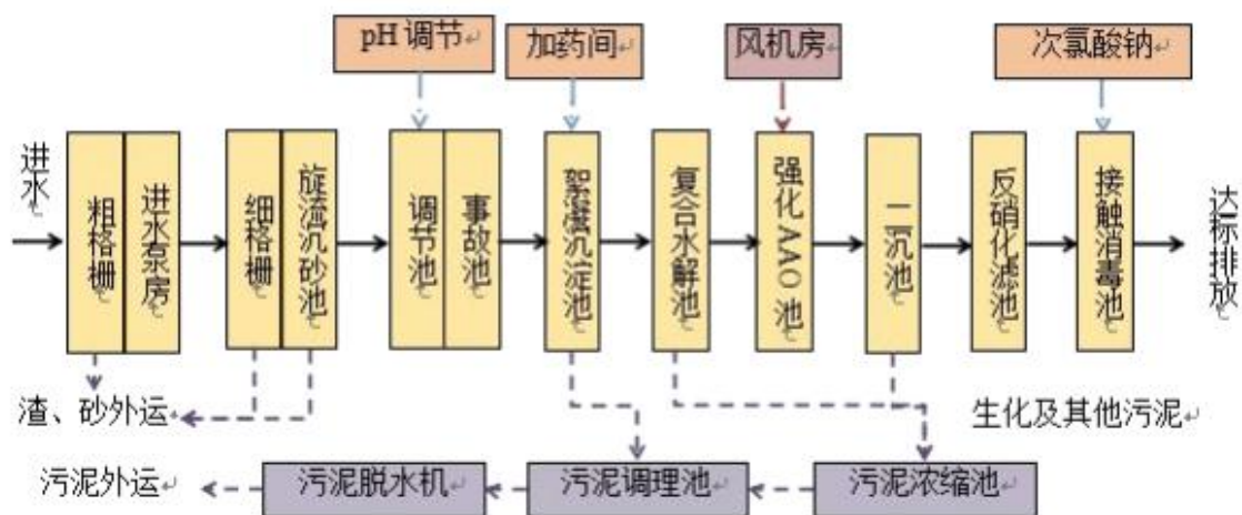
图 4-4 园区污水处理工艺流程图
