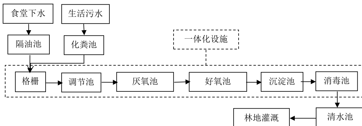
图 4-9 地埋式一体化生活污水处理工艺流程图
