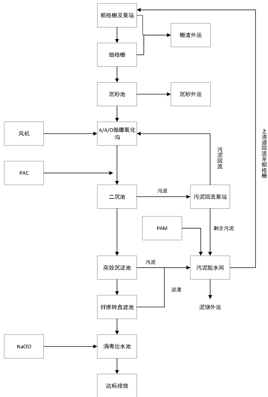
图 4-6 雷州市污水厂污水处理工艺流程图
