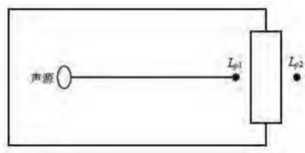
图 4-10 室内声源等效为室外声源图例
