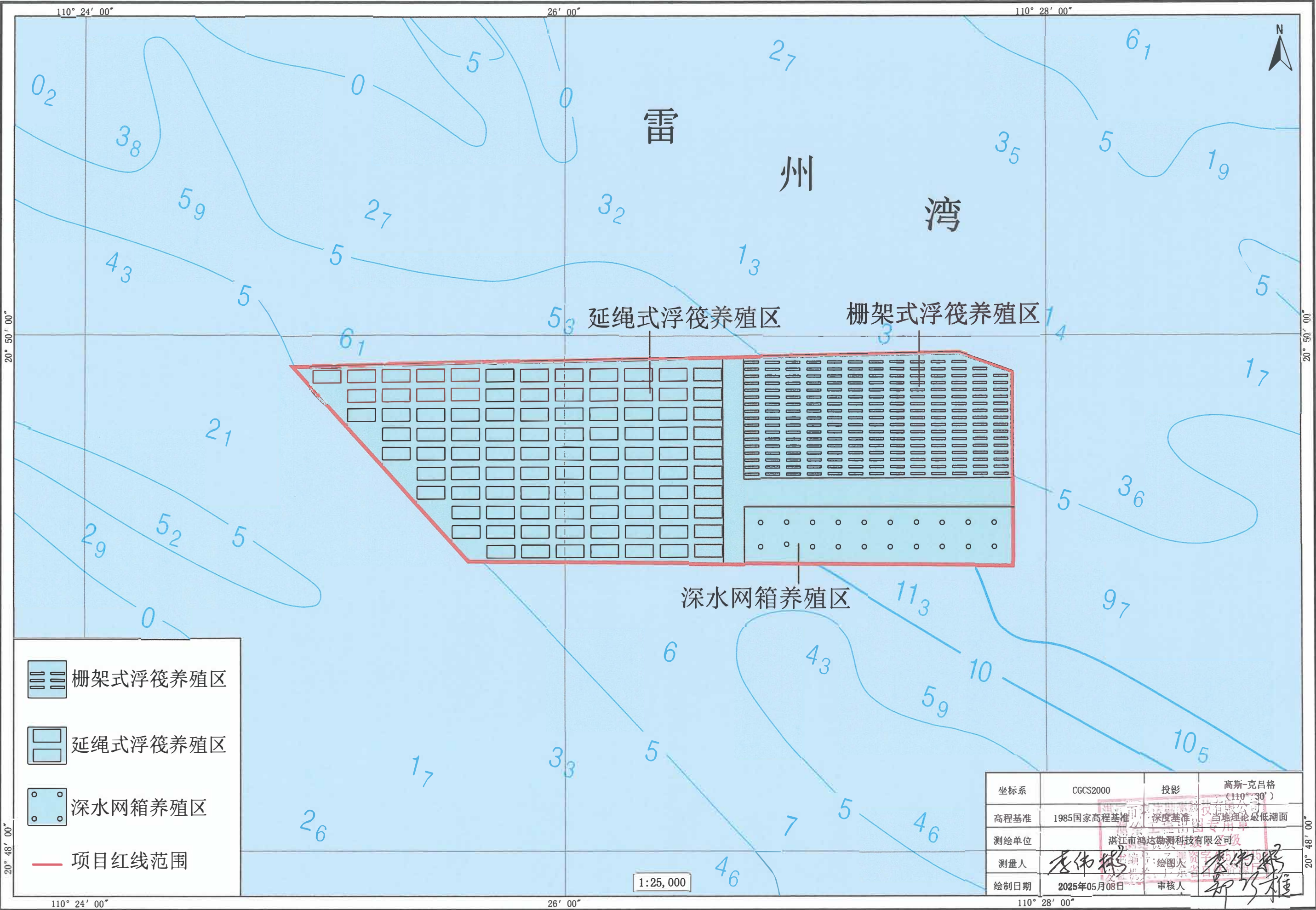
湛江市雷州湾4号海域现代化海洋牧场建设项目宗海平面布置图
