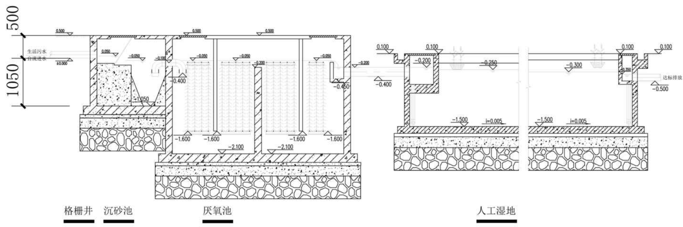
厌氧+人工湿地污水处理池流程图
