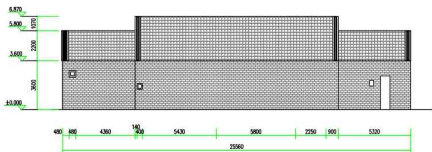
⑥—①立面图
