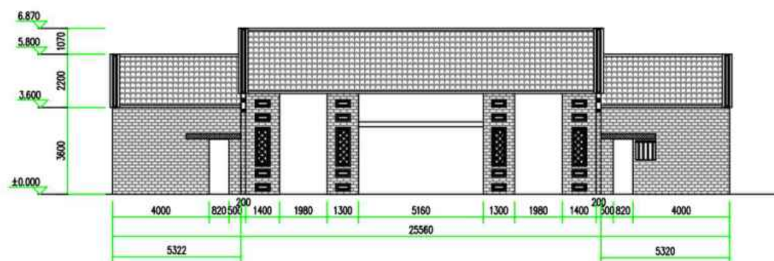
①—⑥立面图
