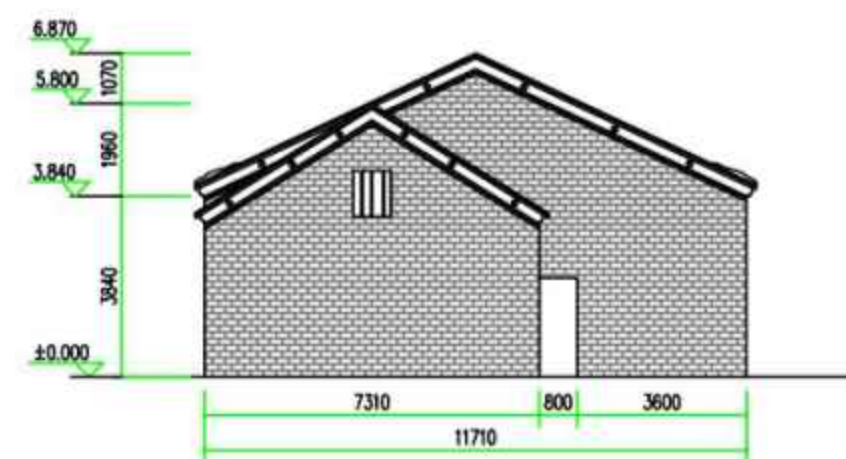
①—⑥立面图
