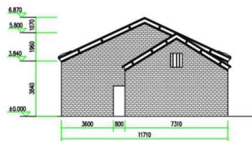
⑥—①立面图
