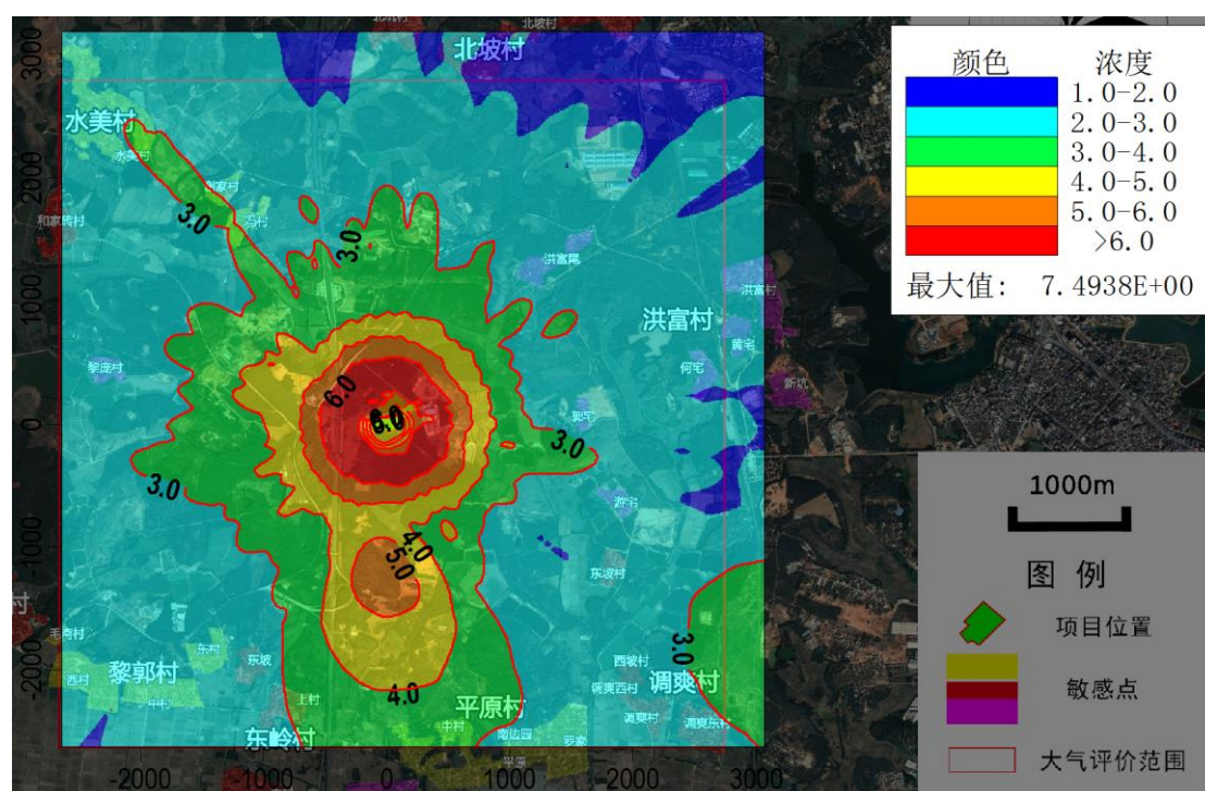
图 6-1-10 HCl 贡献浓度小时值分布图 ( \mu\text{g}/\text{m}^3 )
