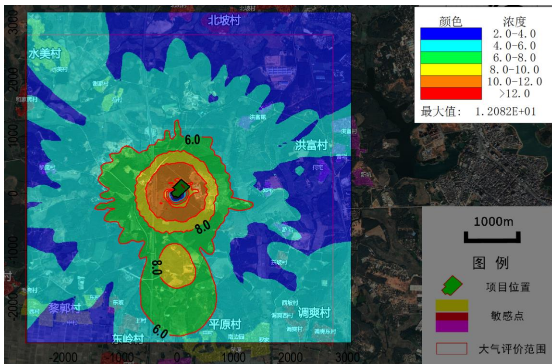
图 6-1-7 SO 2 贡献浓度小时值分布图 (μg/m 3 )
