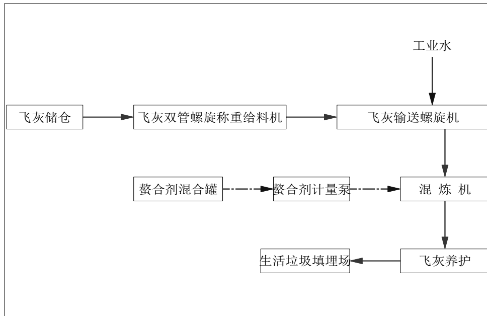
图 4-7-2 飞灰固化工艺流程图
