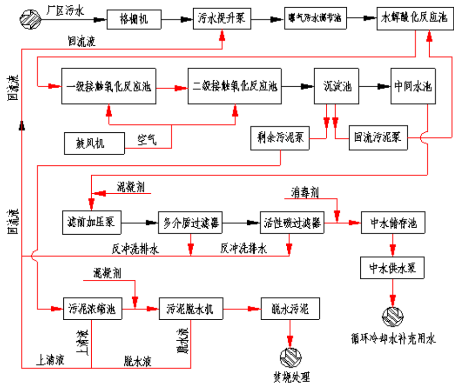
图 9-2-2 低浓度污水处理工艺流程示意图
