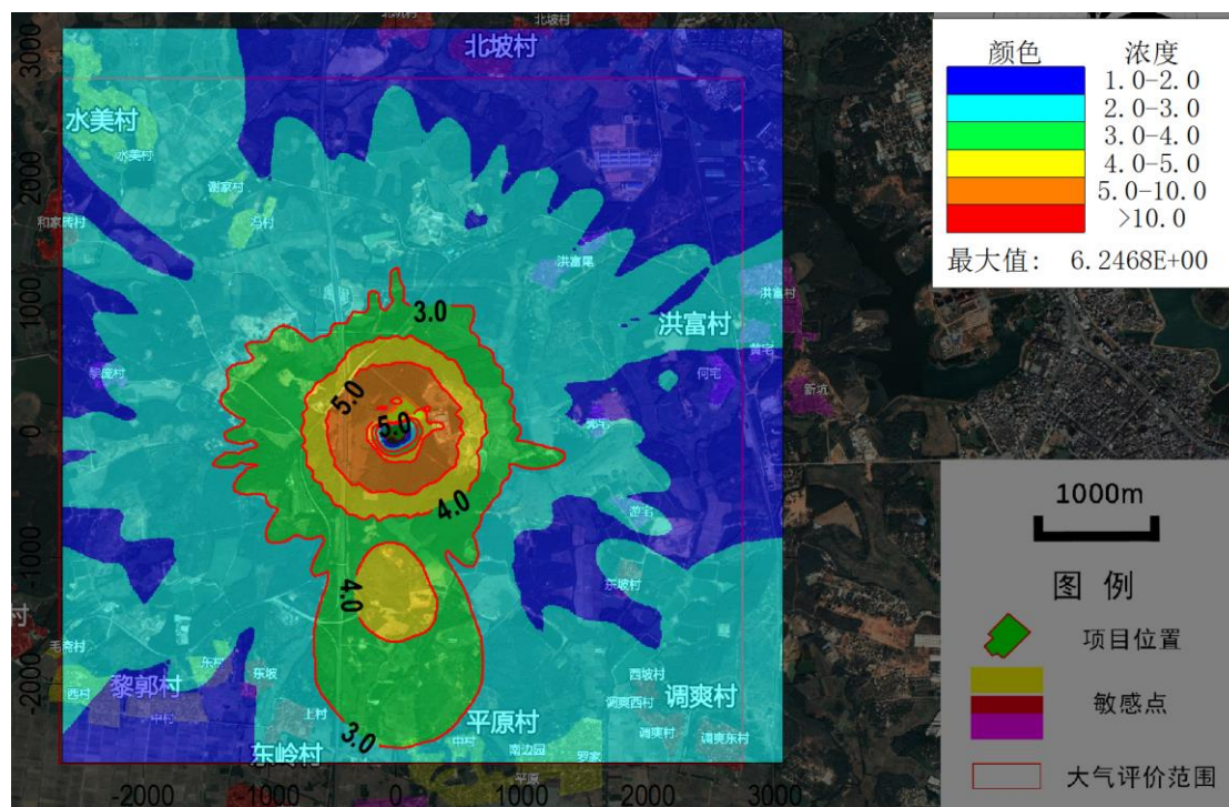
图 6-1-11 CO 贡献浓度小时值分布图 ( \mu\text{g}/\text{m}^3 )
