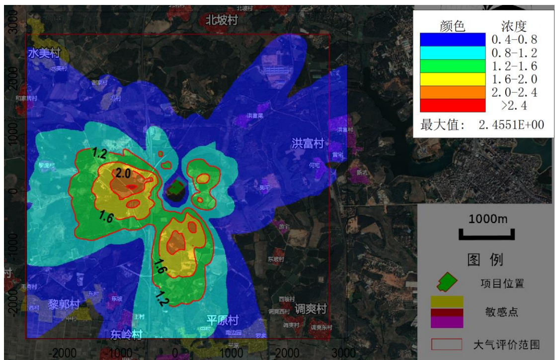
图 6-1-19 CO 贡献浓度日均值分布图 ( \mu\text{g}/\text{m}^3 )
