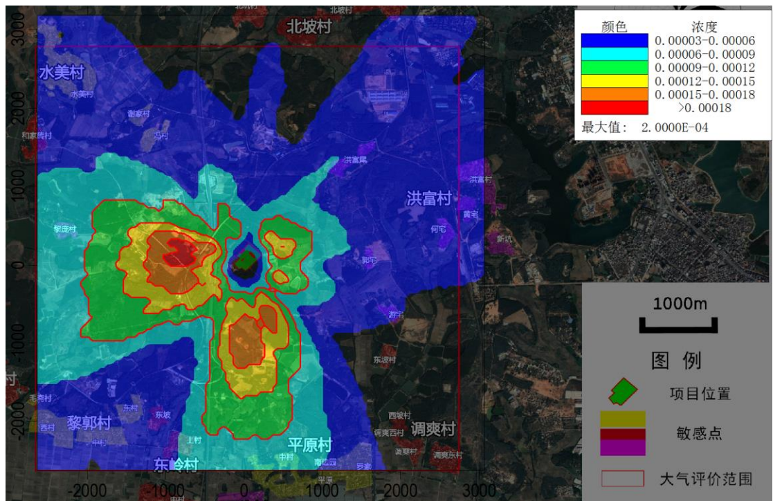
图 6-1-22 Hg 贡献浓度日均值分布图 ( \mu\text{g}/\text{m}^3 )
