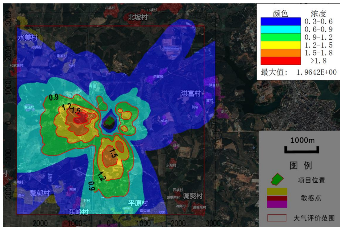
图 6-1-23 HCl 贡献浓度日均值分布图 ( \mu\text{g}/\text{m}^3 )
