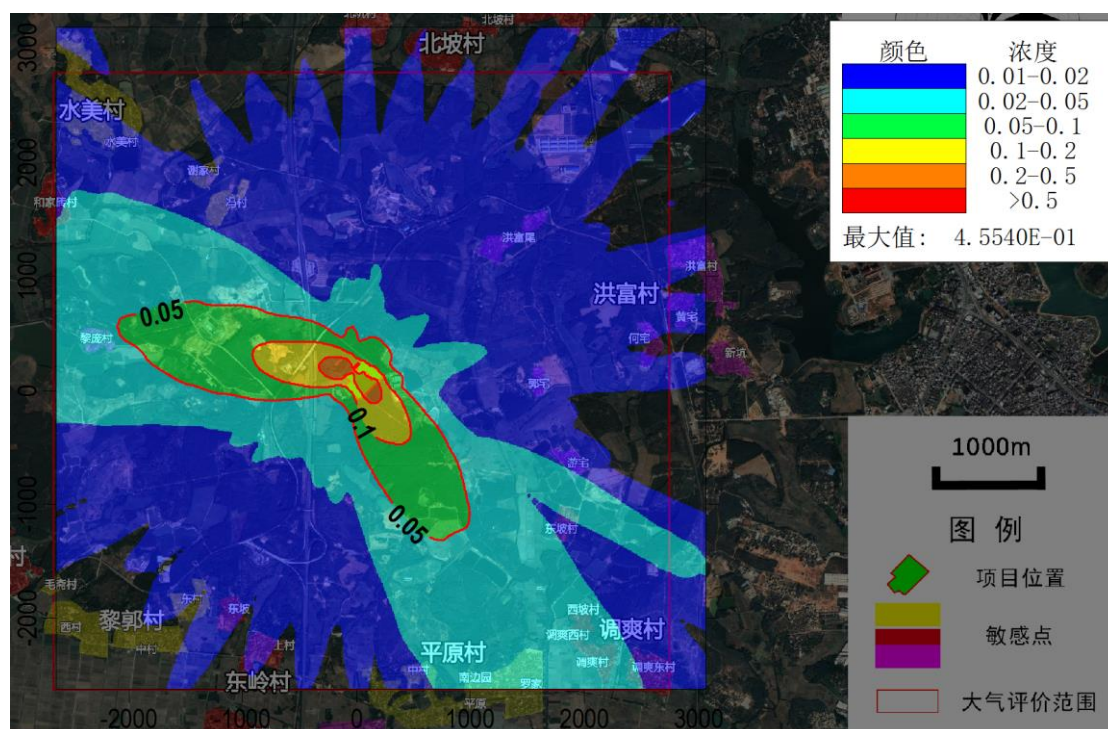
图 6-1-13 H 2 S 贡献浓度小时值分布图 (µg/m 3 )
