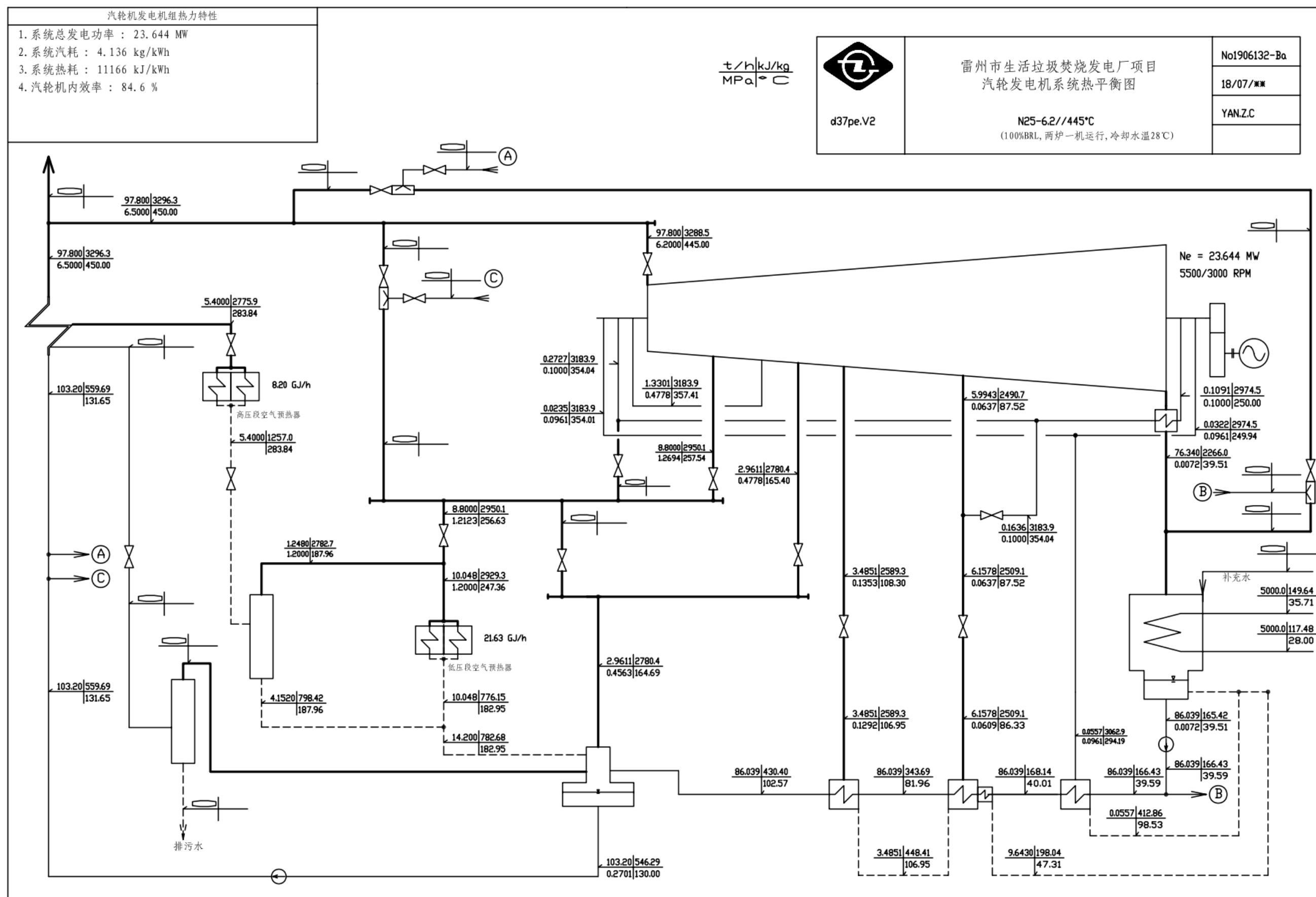
图 4-5-1 项目热平衡图
