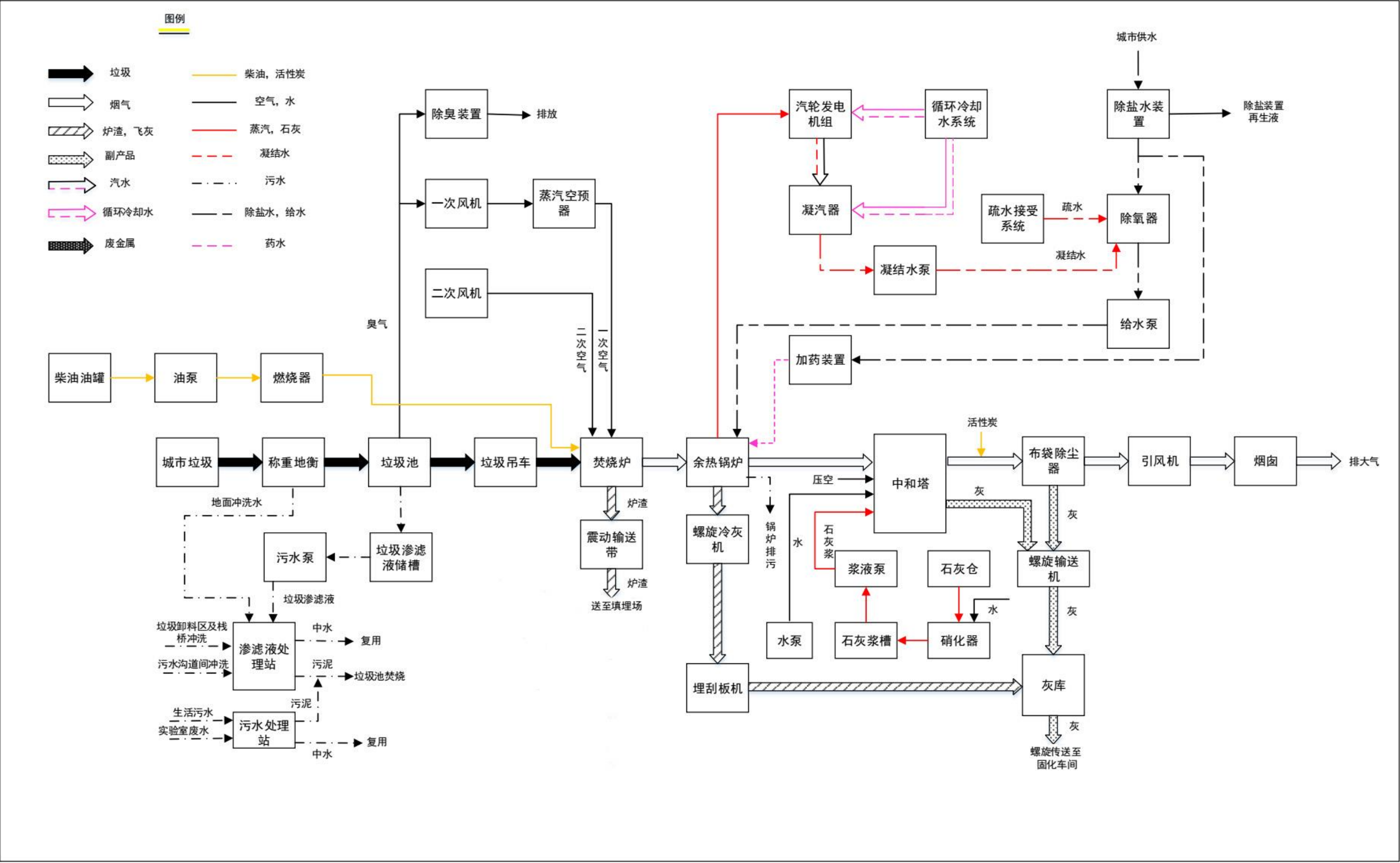
图 4-7-1 本项目工艺流程图
