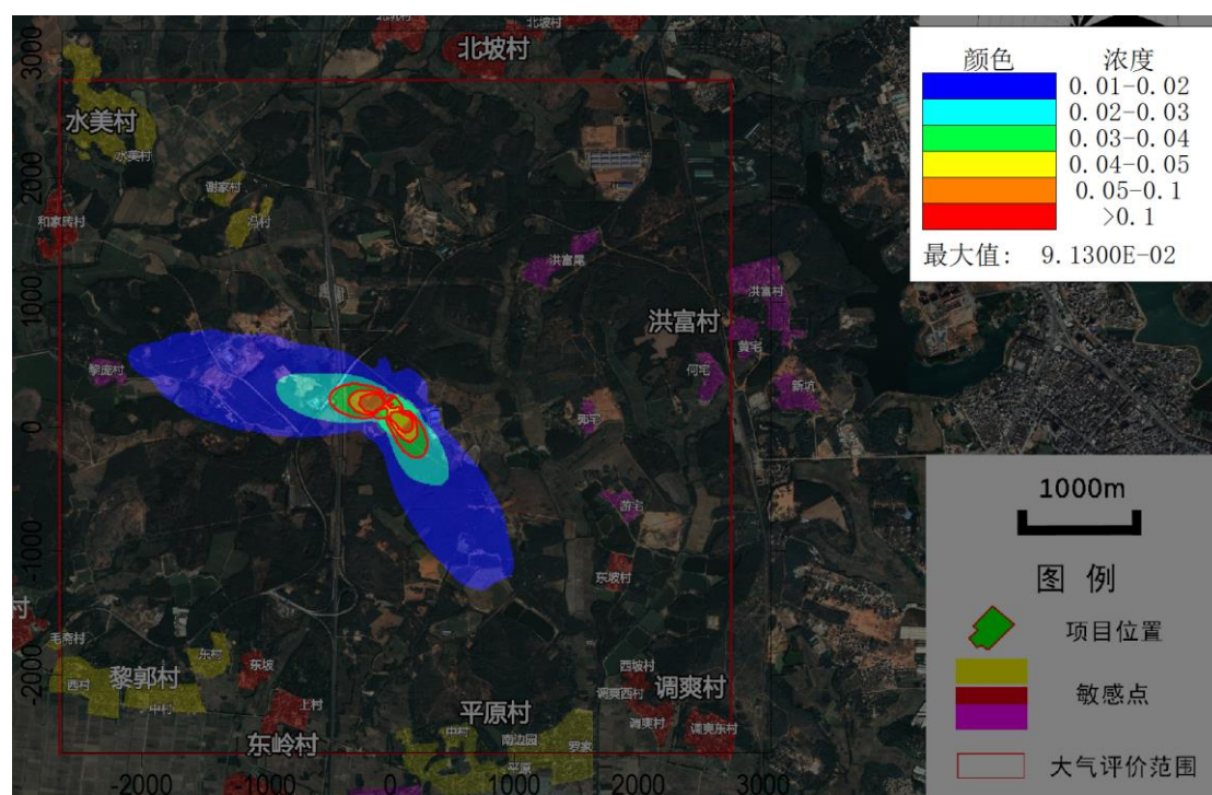
图 6-1-12 \text{CH}_3\text{SH} 贡献浓度小时值分布图 ( \mu\text{g}/\text{m}^3 )
