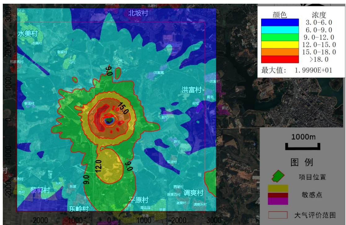
图 6-1-16 NO 2 贡献浓度日均值分布图 (μg/m 3 )
