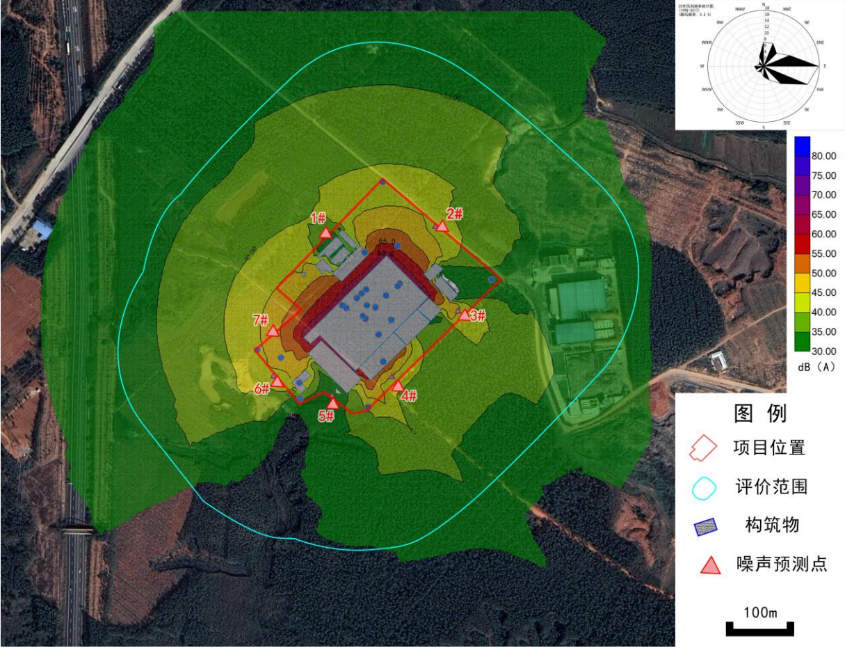
图 6-4-1 噪声贡献值等声值线图
