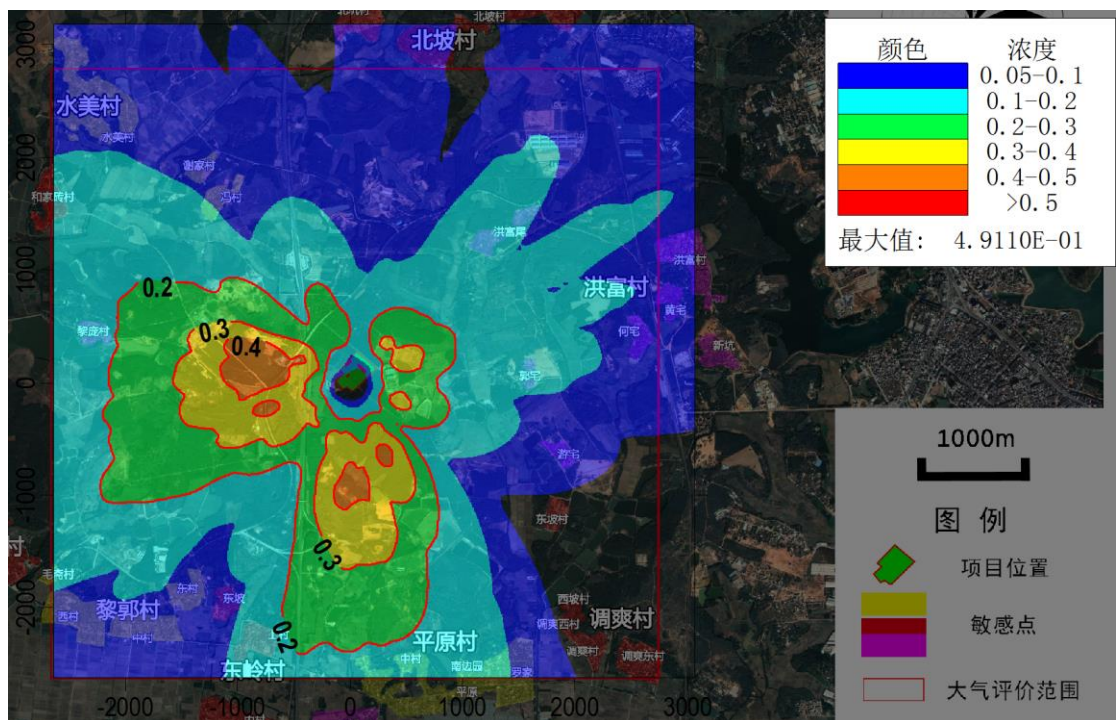
图 6-1-18 PM 10 贡献浓度日均值分布图 (μg/m 3 )
