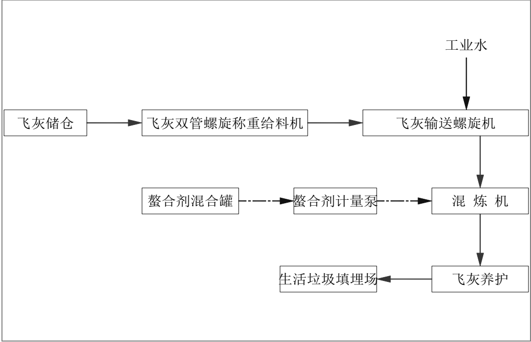
图 3-2-3 螯合剂固化工艺流程
