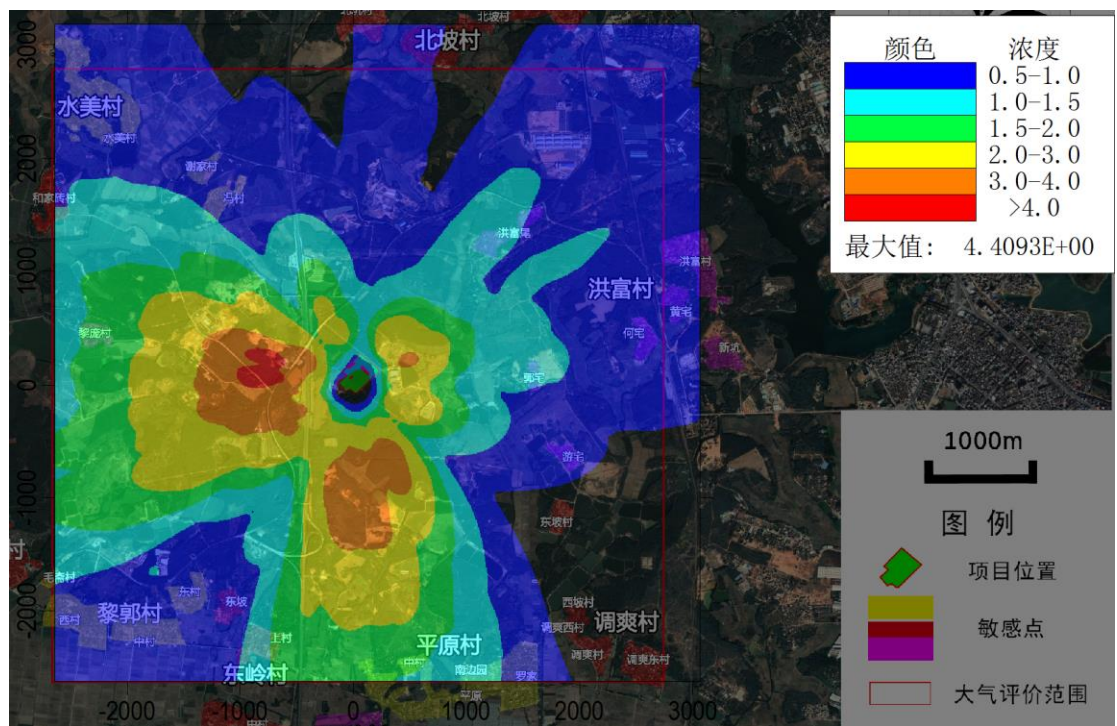
图 6-1-20 \text{PM}_{2.5} 贡献浓度日均值分布图 ( \mu\text{g}/\text{m}^3 )
