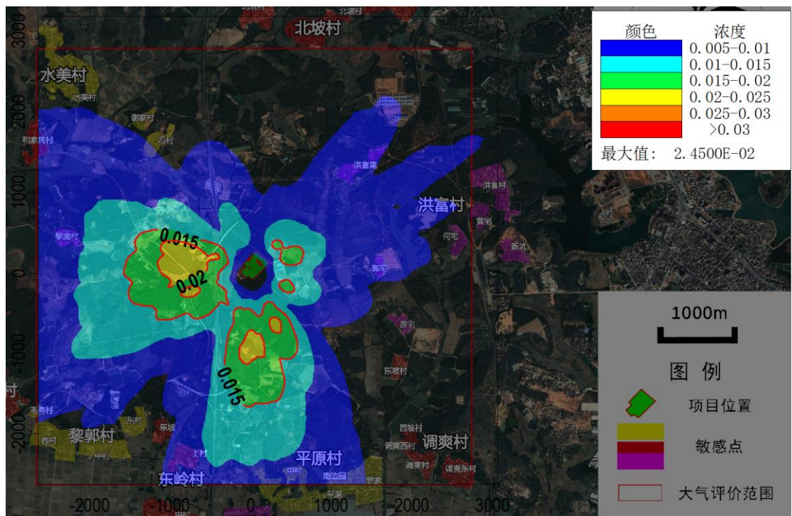
图 6-1-21 Pb 贡献浓度日均值分布图 ( \mu\text{g}/\text{m}^3 )
