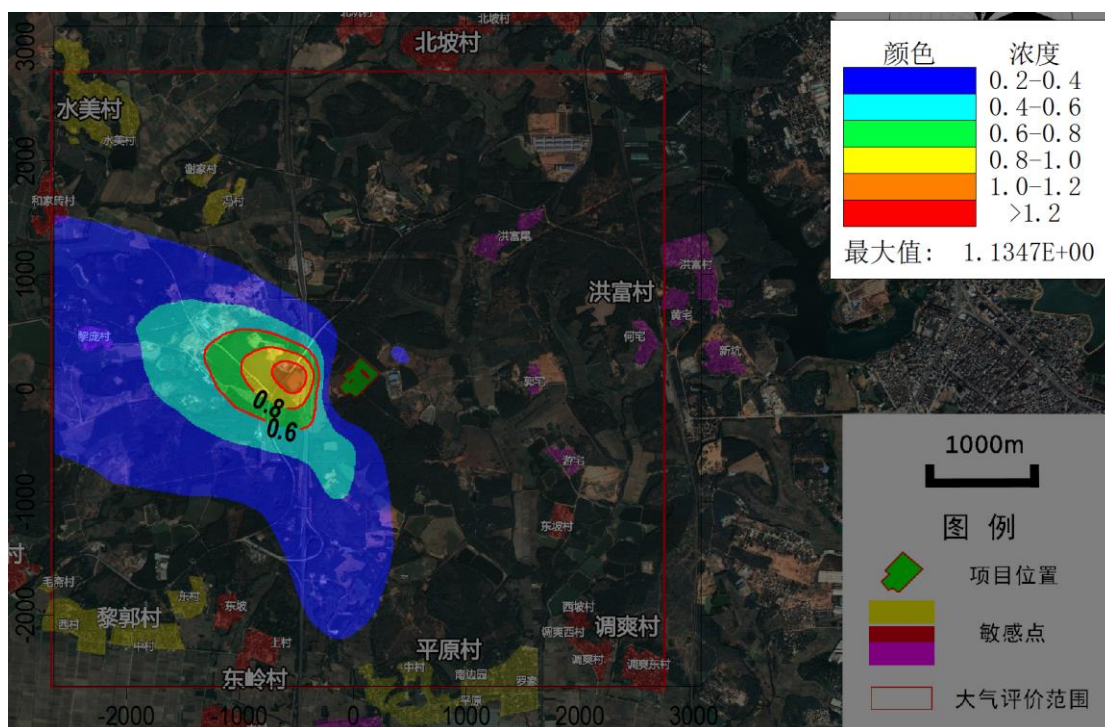
图 6-1-24 \text{SO}_2 贡献浓度年均值分布图 ( \mu\text{g}/\text{m}^3 )
