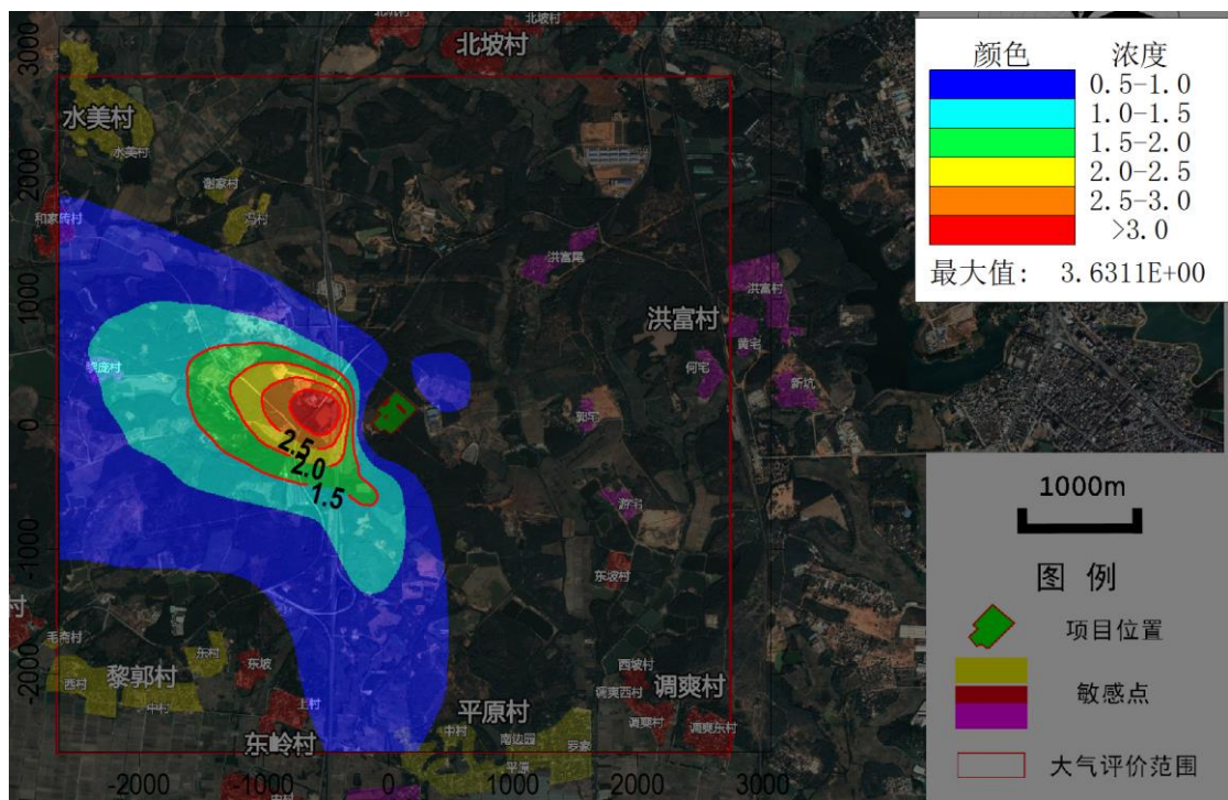
图 6-1-25 NO 2 贡献浓度年均值分布图 (μg/m 3 )
