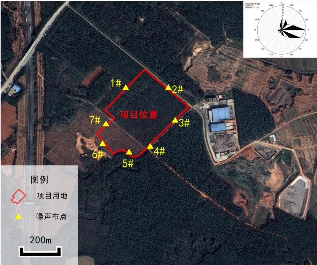
图 5-3-3 声环境环境监测点位布设示意图
