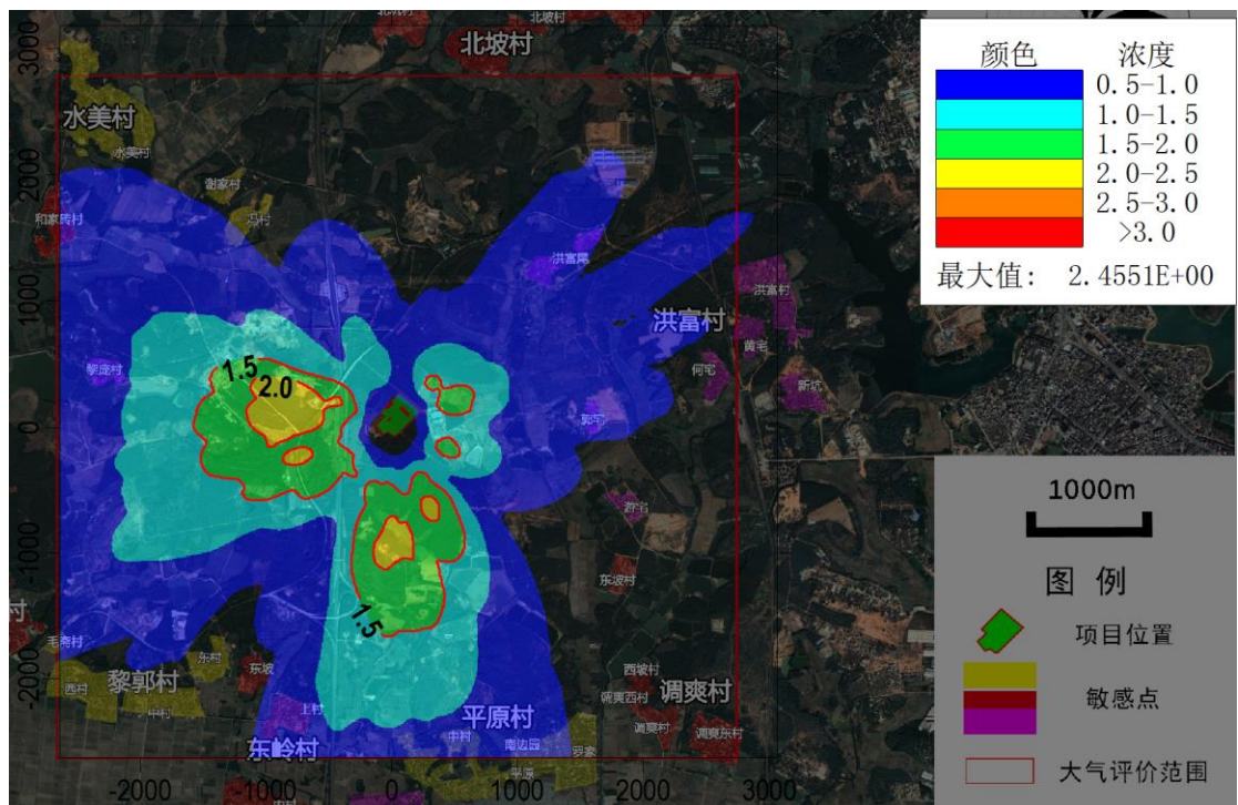
图 6-1-15 SO 2 贡献浓度日均值分布图 (μg/m 3 )
