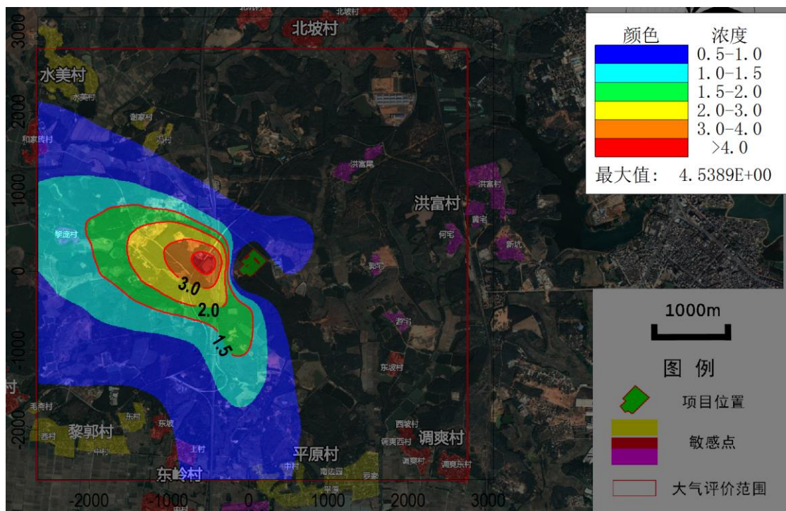
图 6-1-26 NO x 贡献浓度年均值分布图 (μg/m 3 )
