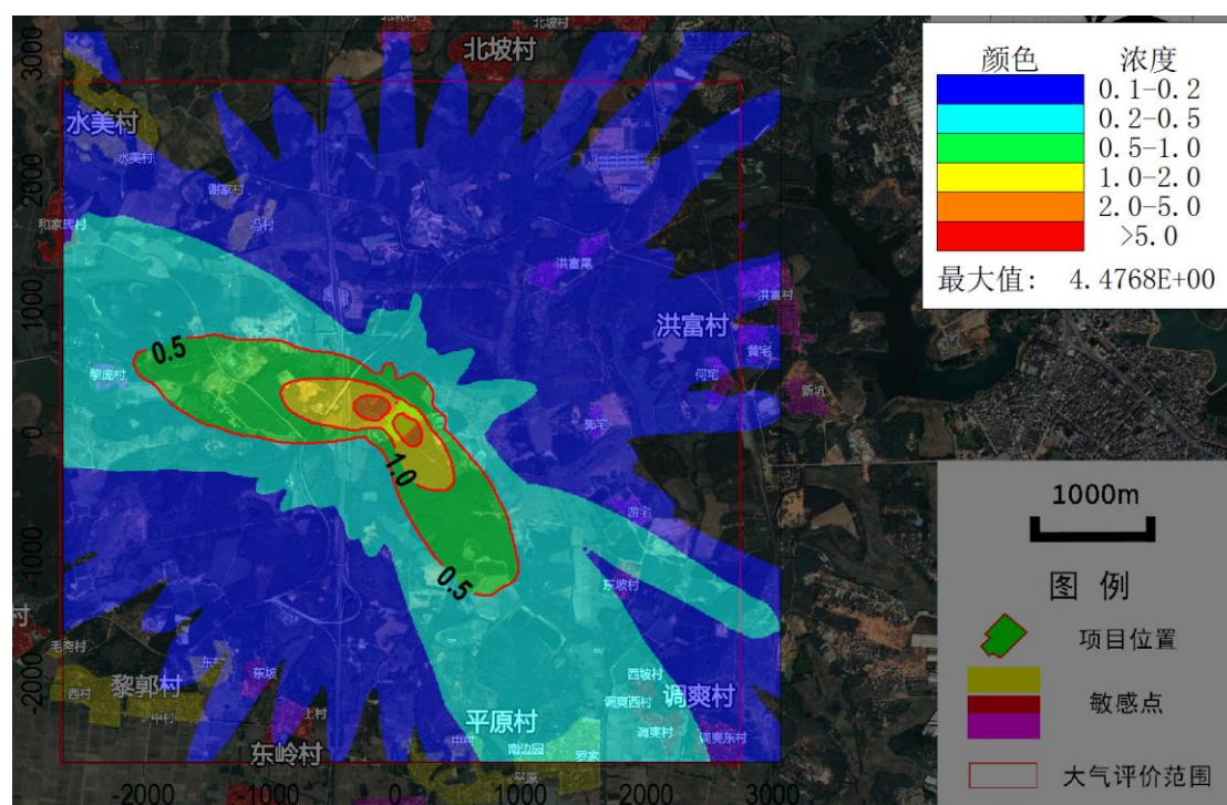
图 6-1-14 NH 3 贡献浓度小时值分布图 (µg/m 3 )
