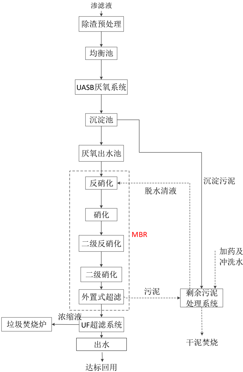
图 9-2-1 高浓度废水处理系统处理工艺
