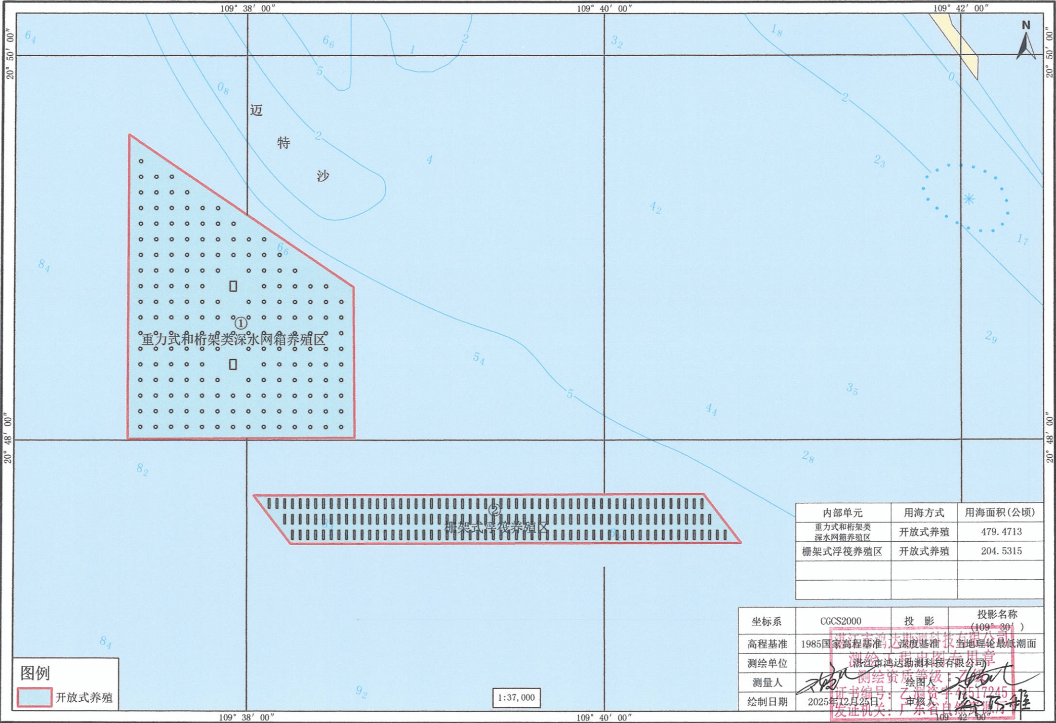
湛江市企水7号海域现代化海洋牧场建设项目宗海平面布置图
