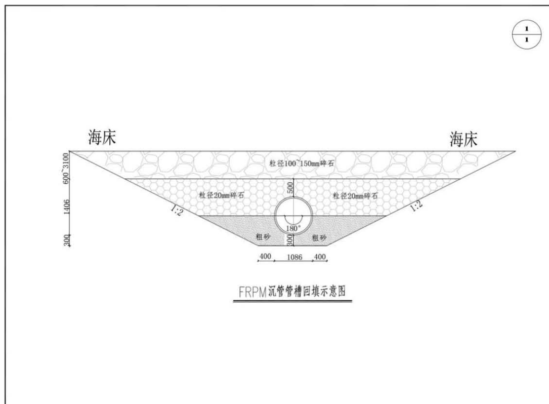
图 3.8.3-2 本项目污水排海管道开挖回填示意图
