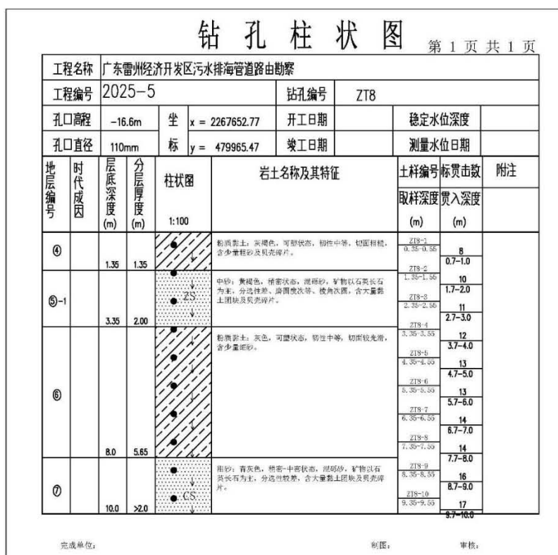
图 5.1.3-7 ZT7 与 ZT8 钻孔柱状图
