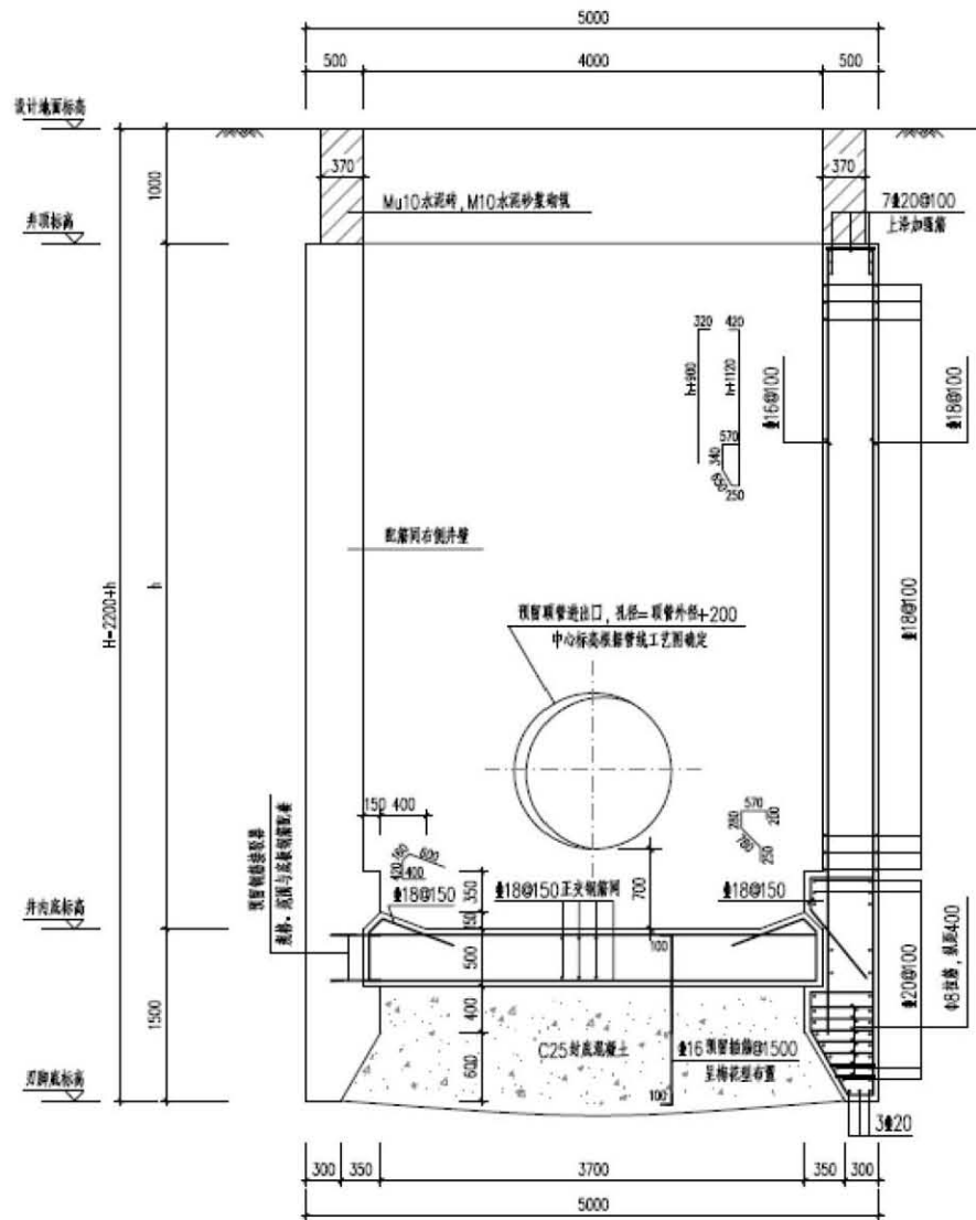
图 3.8.2-4 顶管接收井剖面图
