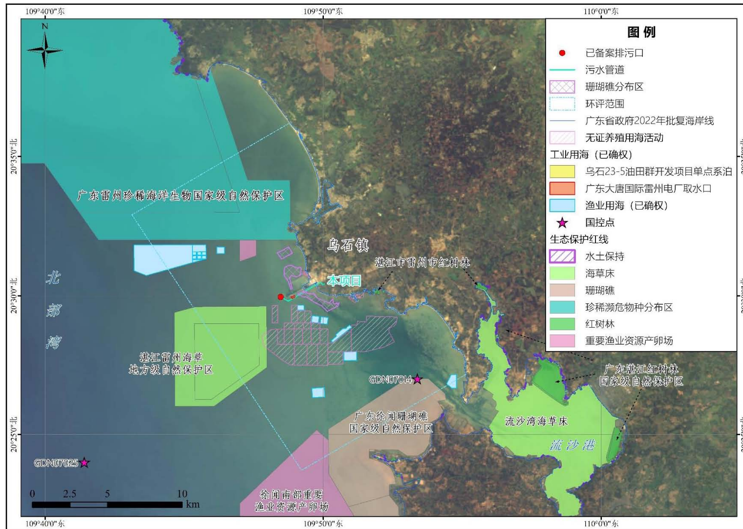
图 7.3.2-1 排污口布置
