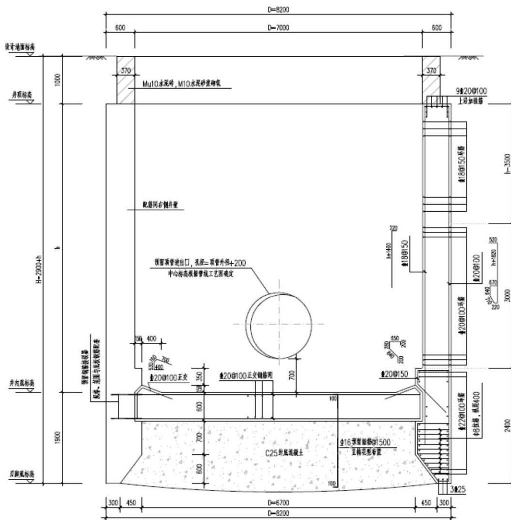
图 3.8.2-3 顶管工作井剖面图
