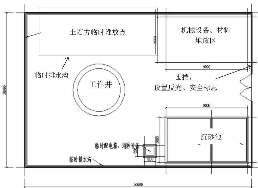
图 3.8.1-3 陆域顶管施工工作井施工场地平面布置图
