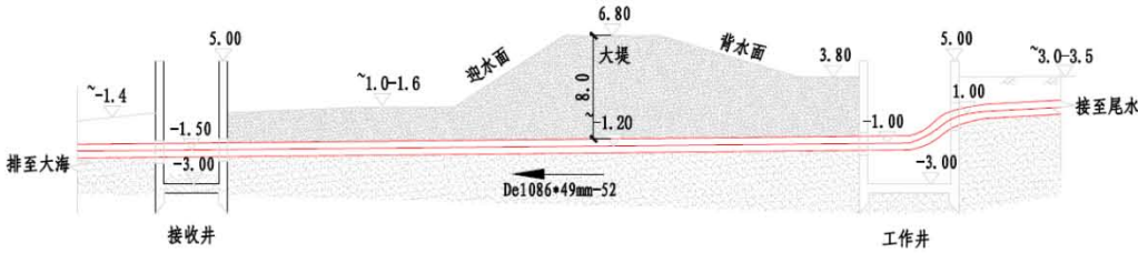
管道穿越大堤剖面示意图
