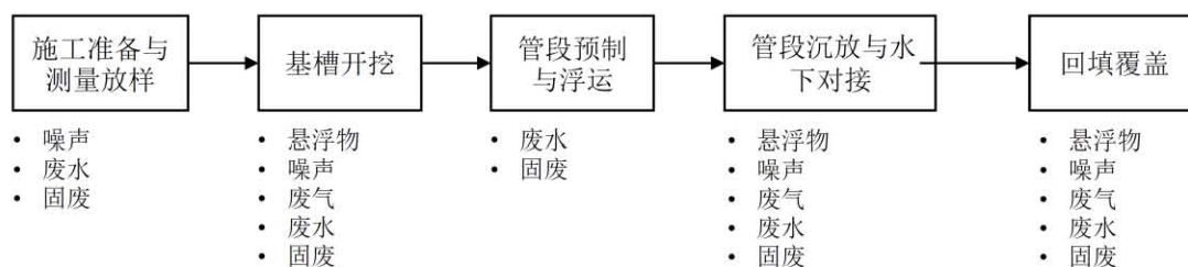
图 4.1.1-1 本项目海上污水管道沉管法主要施工工序及产污环节
