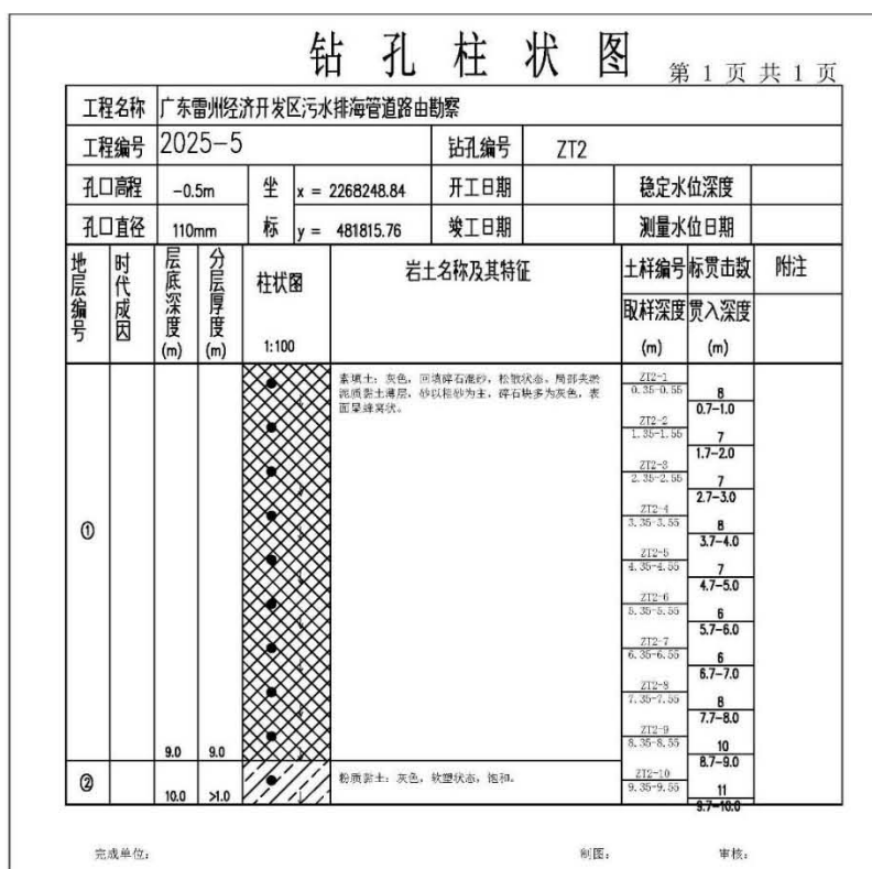
图 5.1.3-4 ZT1 与 ZT2 钻孔柱状图
