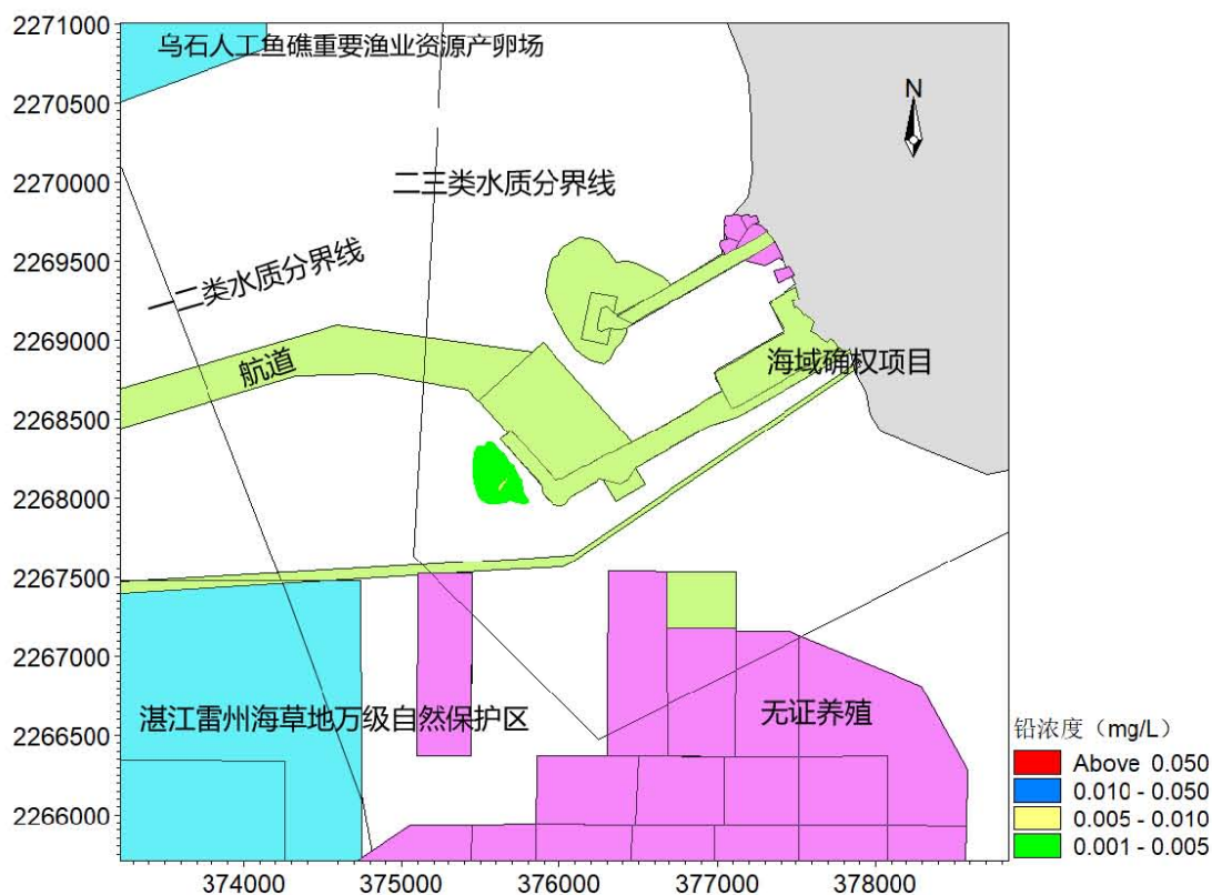
图 7.3.2-13 排污口中层铅扩散范围图
