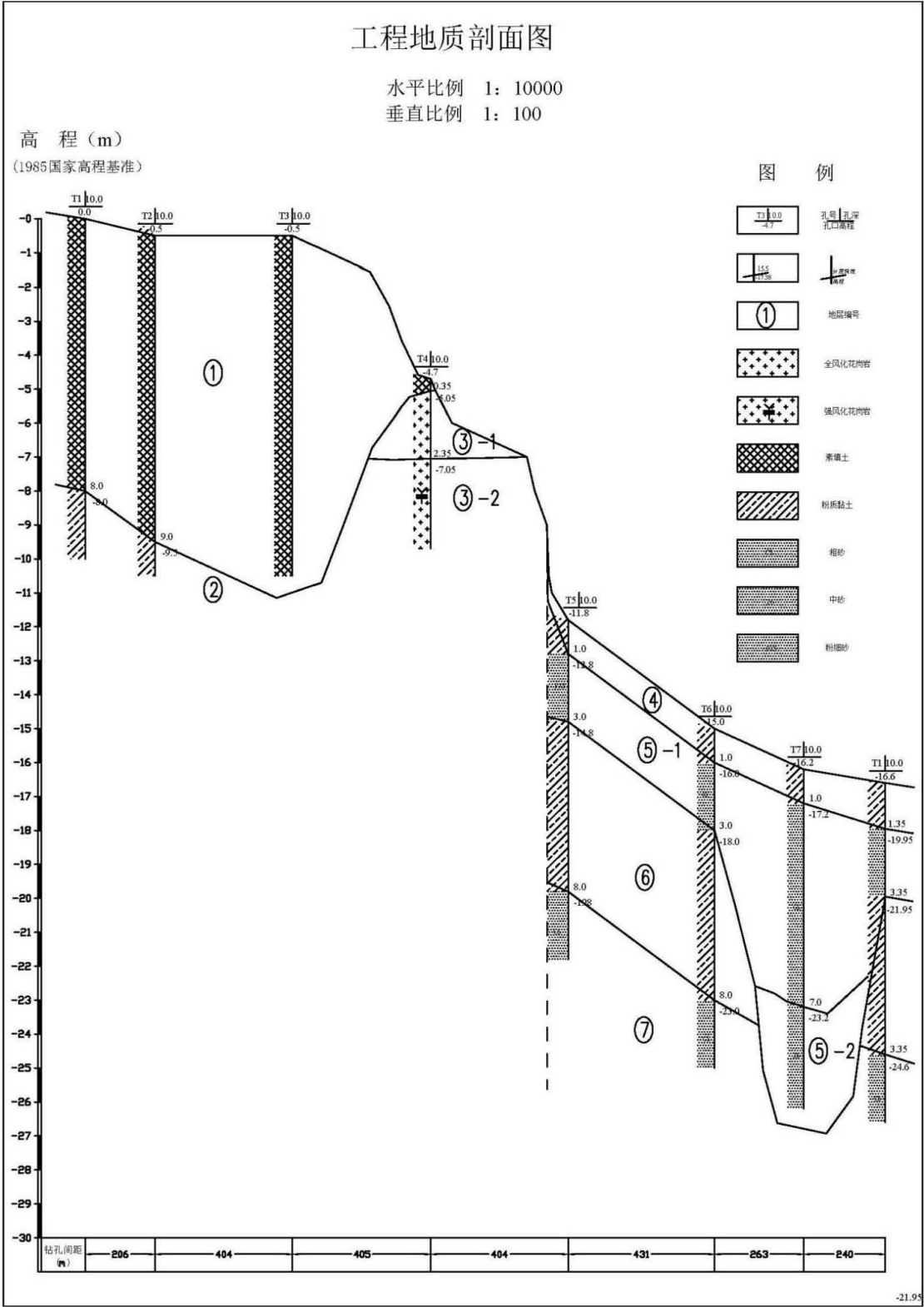
图 5.1.3-3 工程地质剖面图
