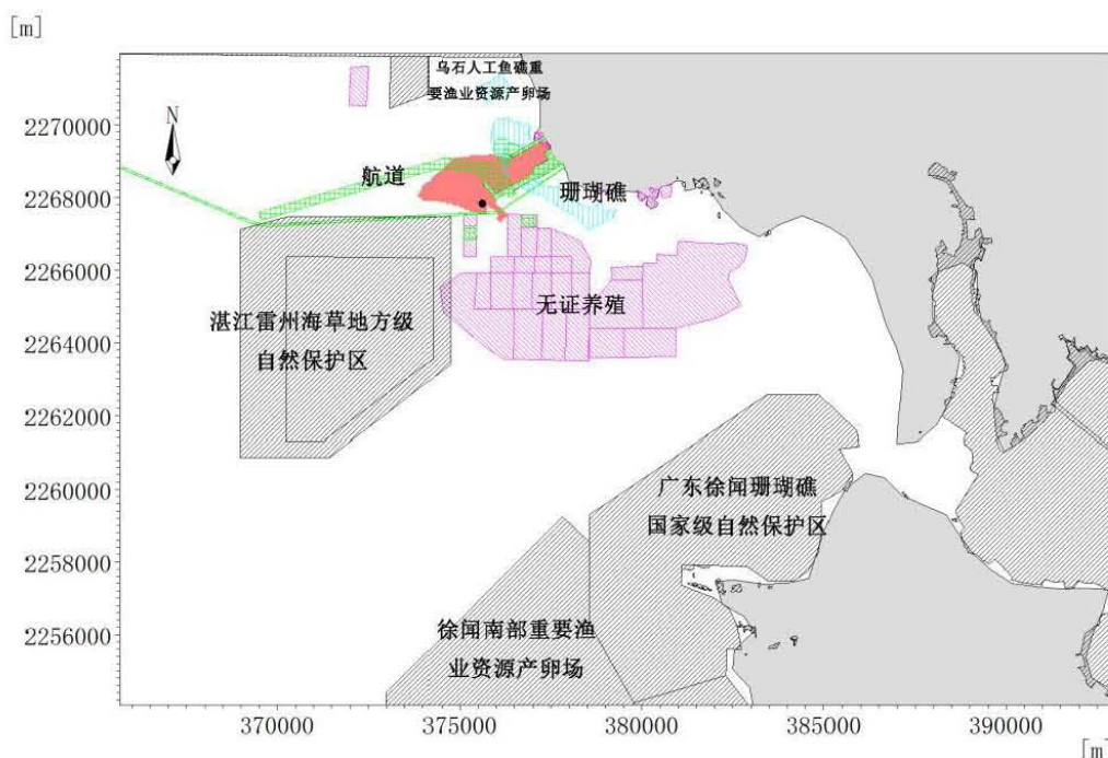
图 8.6.3-1 夏季主导风涨潮 48 小时油膜扩散范围 (SW, 4.68m/s) (黑点为溢油点)
