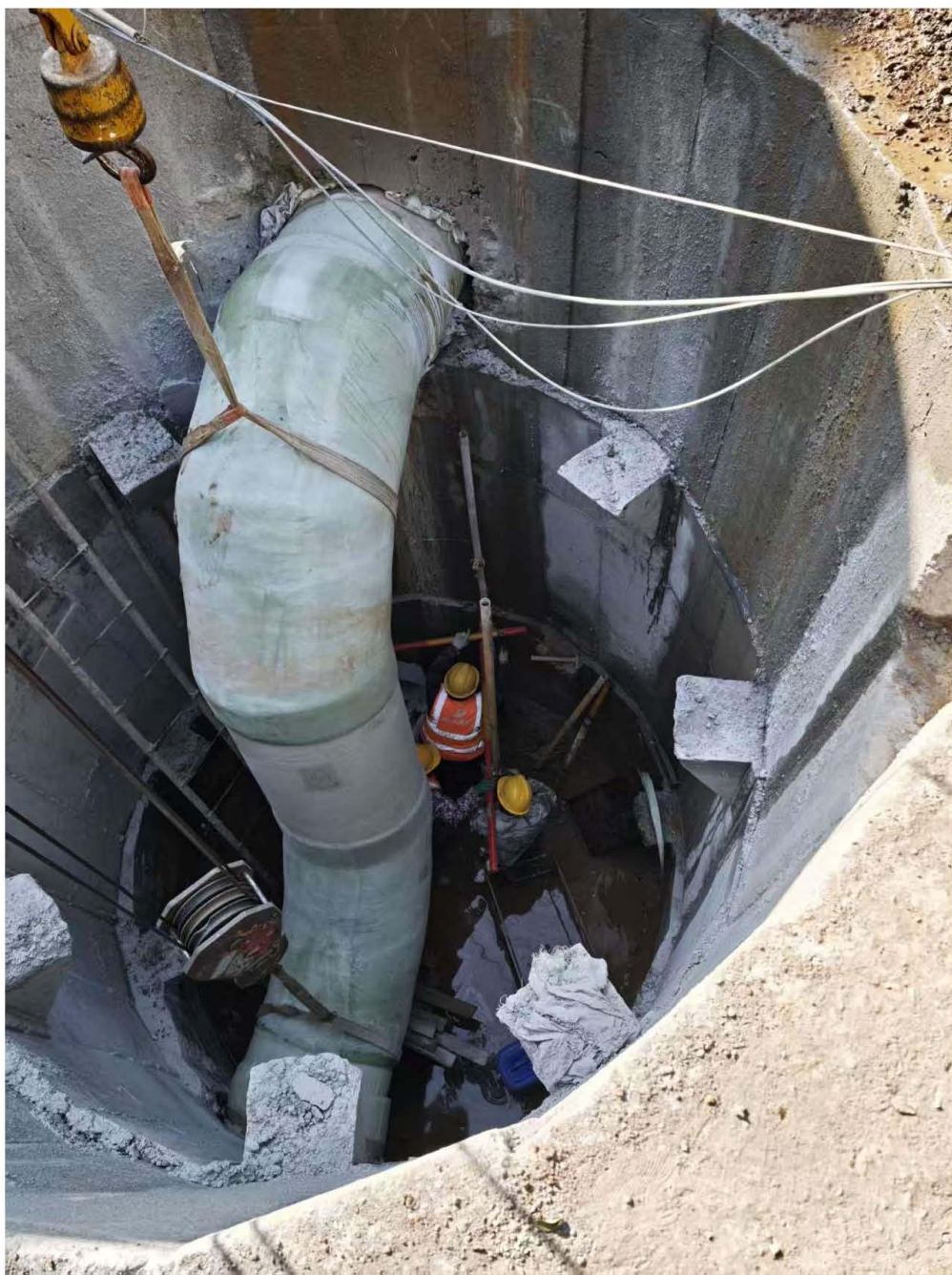
图 3.8.2-5 工作井内弯头衔接实景图
