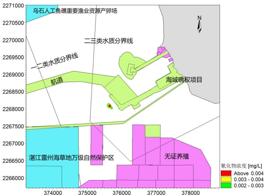
图 7.3.2-25 排污口中层氰化物扩散范围图
