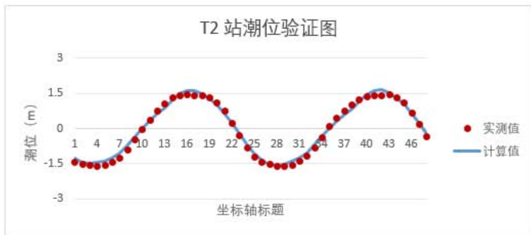
图 7.1.1-3 夏季潮位验证曲线
