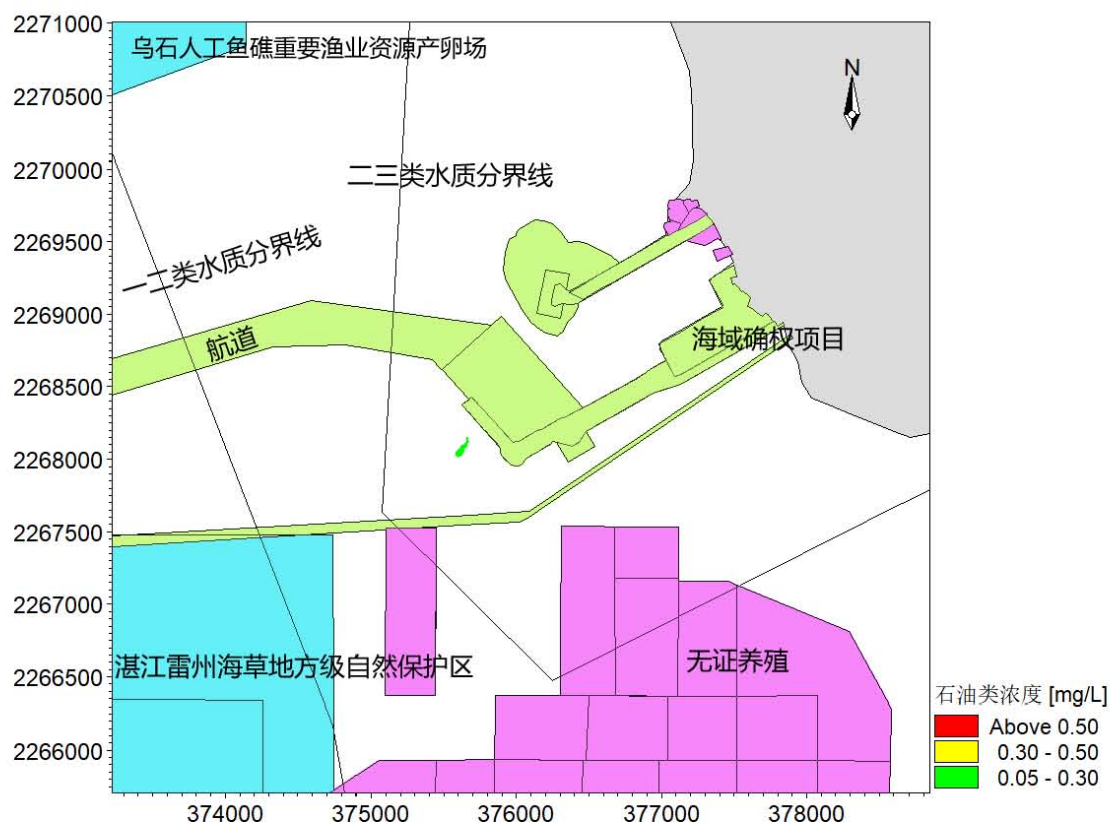
图 7.3.2-7 排污口表层石油类扩散范围图
