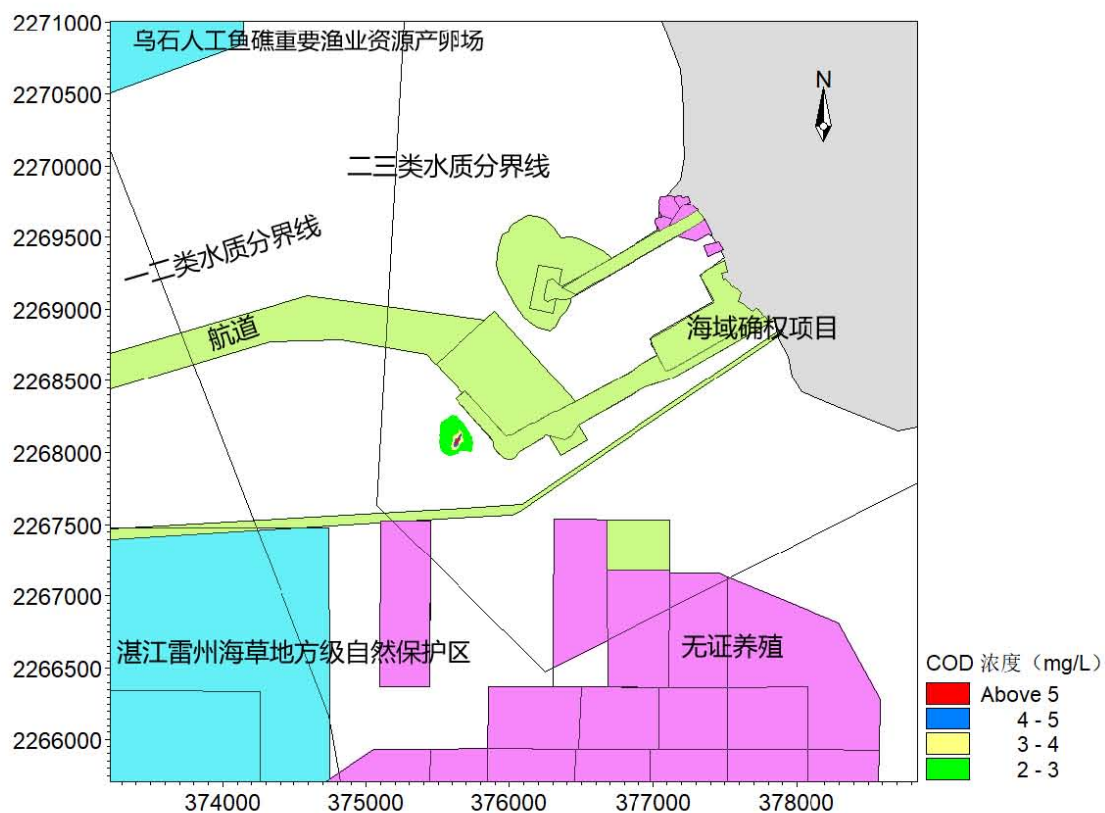
图 7.3.2-3 排污口中层 COD 扩散范围图
