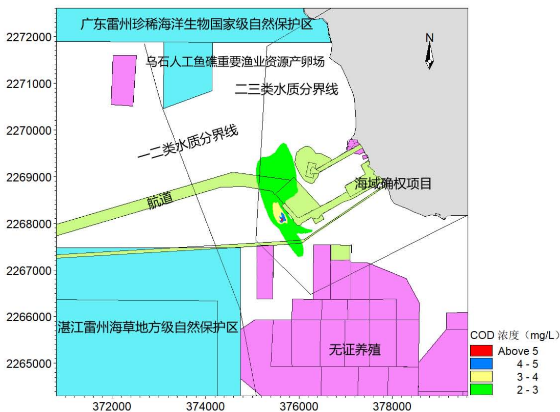
图 7.3.2-28 排污口事故工况底层 COD 扩散范围图
