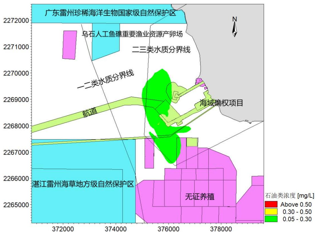
图 7.3.2-32 排污口事故工况表层石油类扩散范围图
