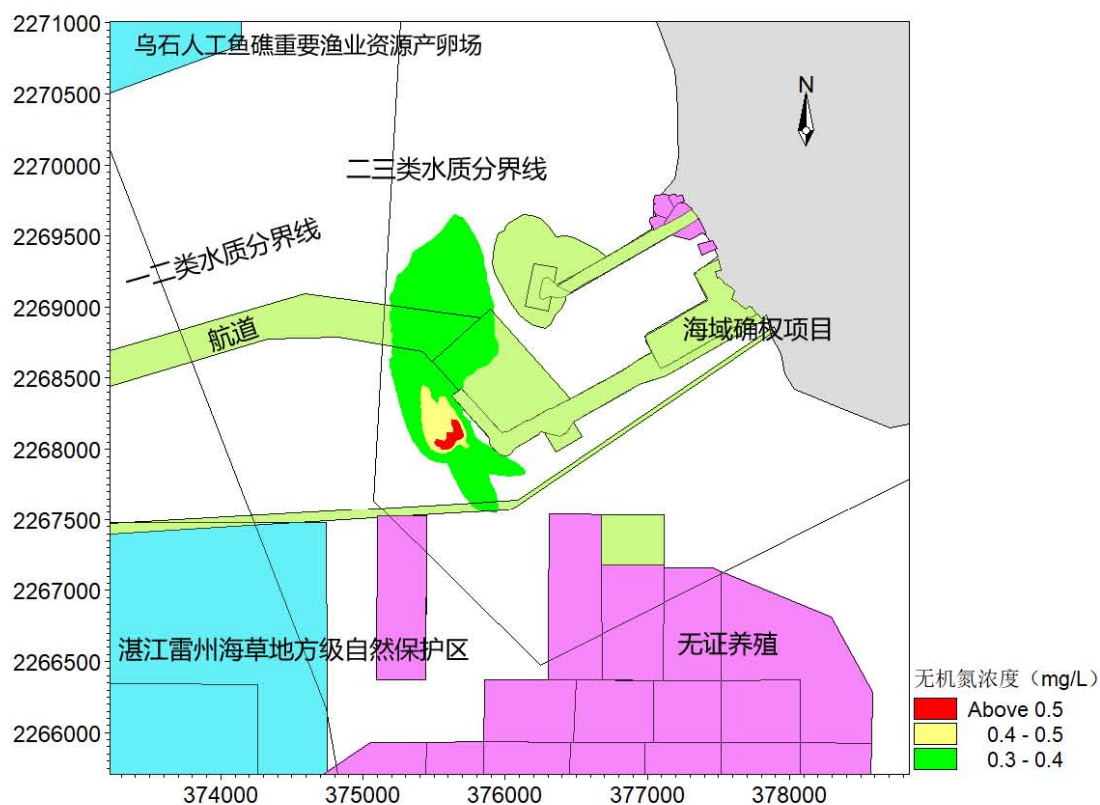
图 7.3.2-4 排污口表层无机氮扩散范围图
