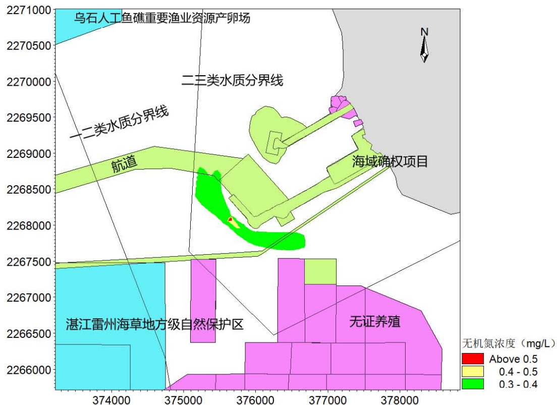
图 7.3.2-17 排污口表层无机氮扩散范围图
