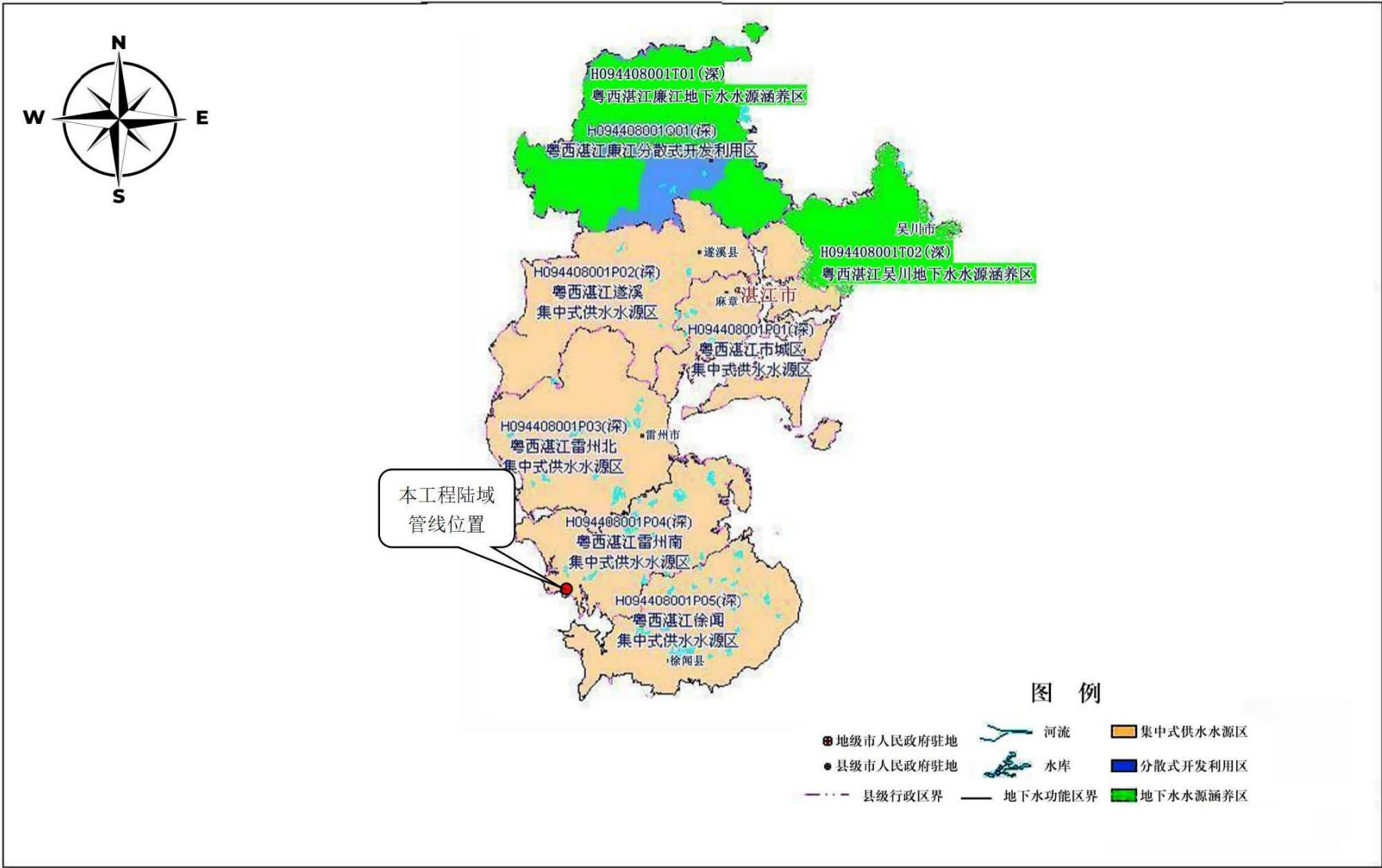
图 2.2-10 本工程陆域管线与湛江市深层地下水功能区相对位置示意图
