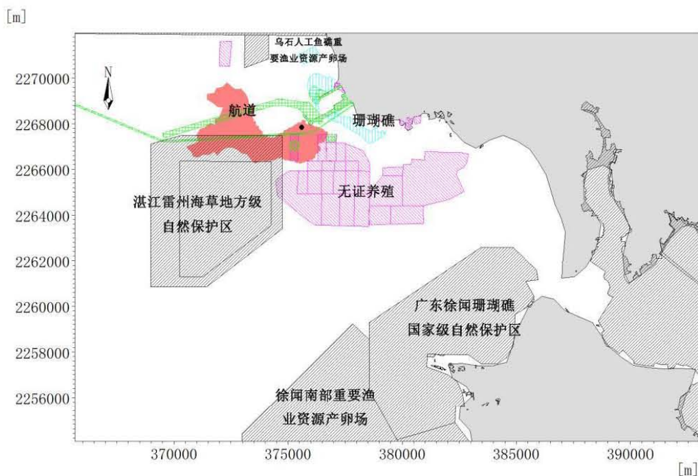
图 8.6.3-4 冬季主导风落潮 48 小时油膜扩散范围 (NE, 5.03m/s)
