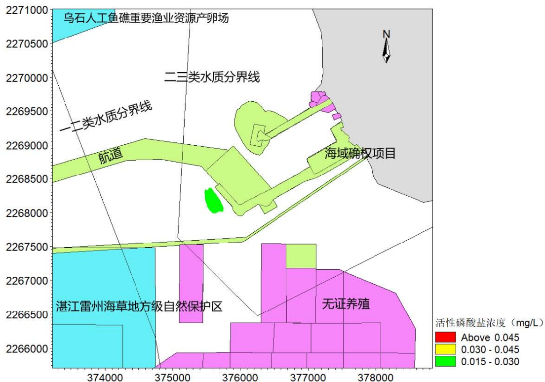
图 7.3.2-10 排污口底层活性磷酸盐扩散范围图
