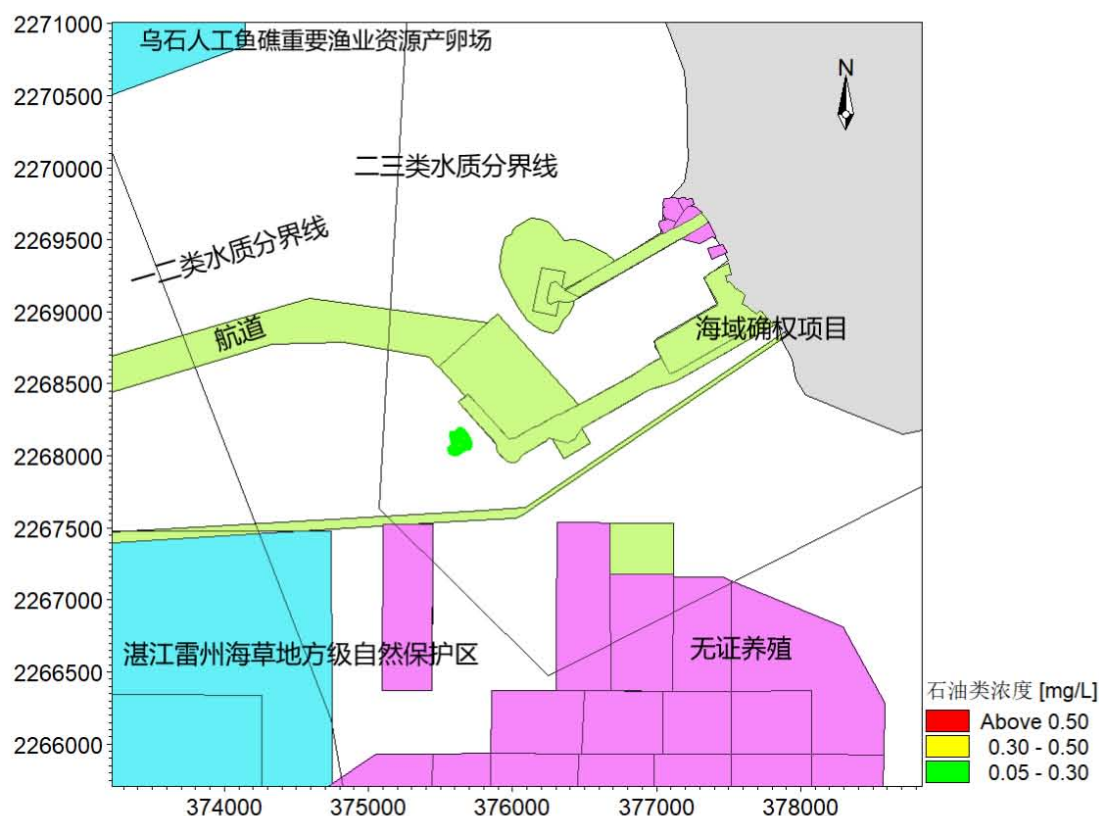
图 7.3.2-8 排污口中层石油类扩散范围图
