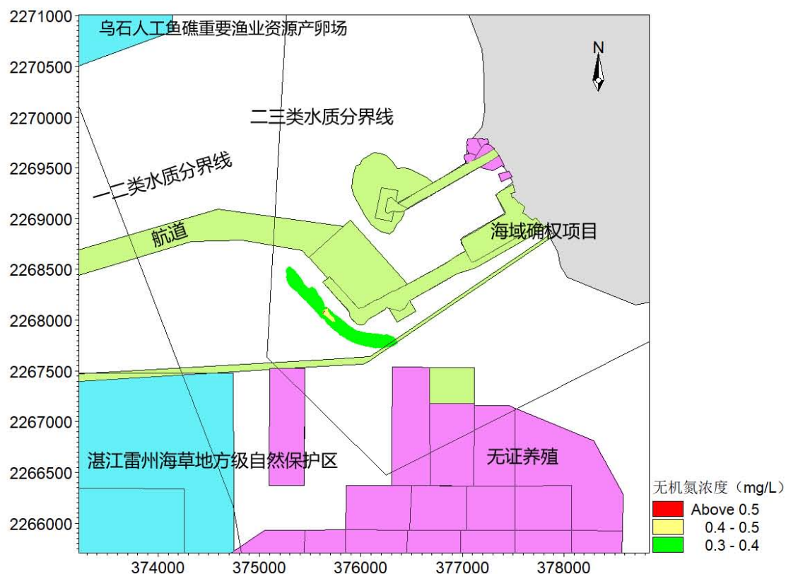
图 7.3.2-19 排污口底层无机氮扩散范围图
