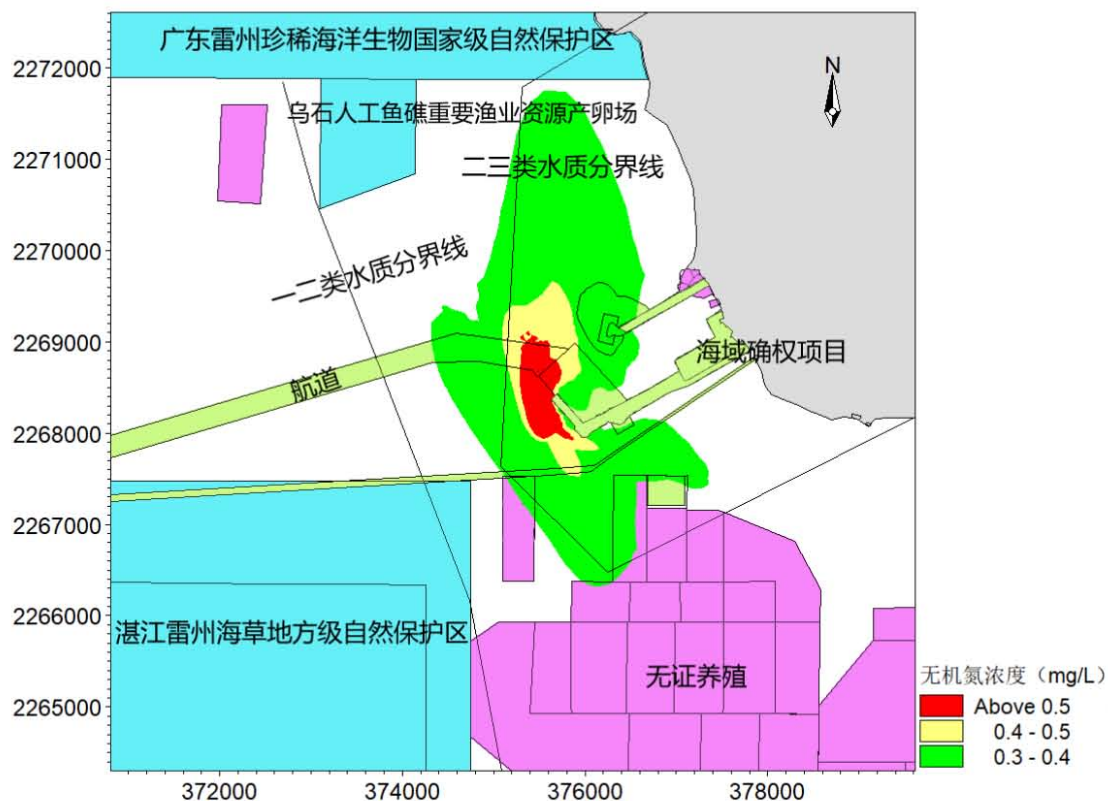
图 7.3.2-29 排污口事故工况表层无机氮扩散范围图
