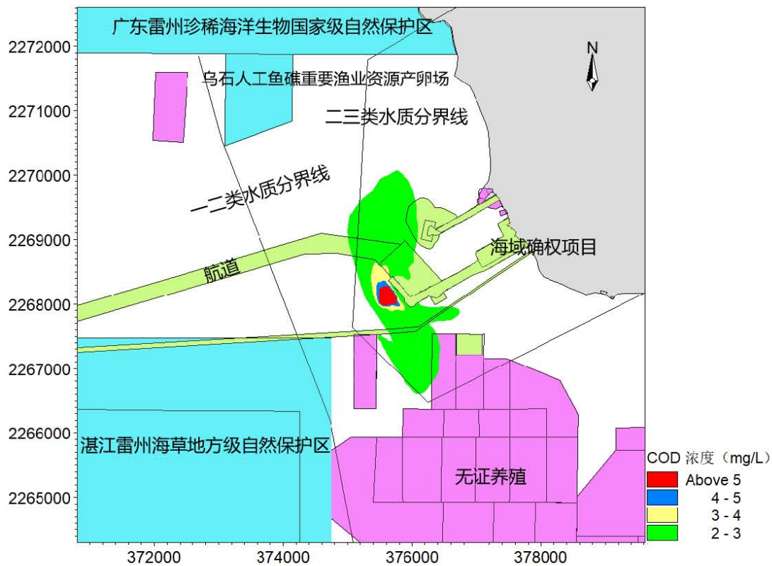
图 7.3.2-27 排污口事故工况中层 COD 扩散范围图
