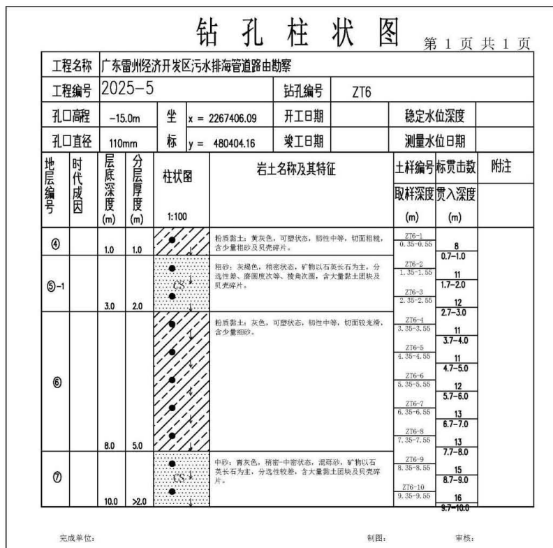
图 5.1.3-6 ZT5 与 ZT6 钻孔柱状图
