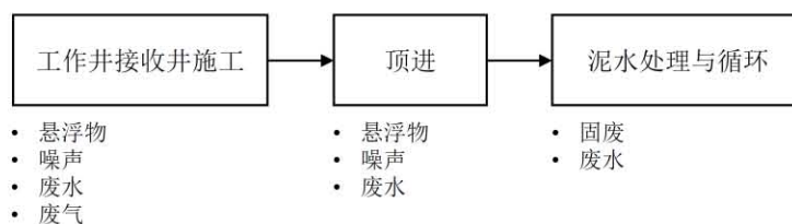
图 4.1.1-2 本项目污水管道顶管法主要施工工序及产污环节
