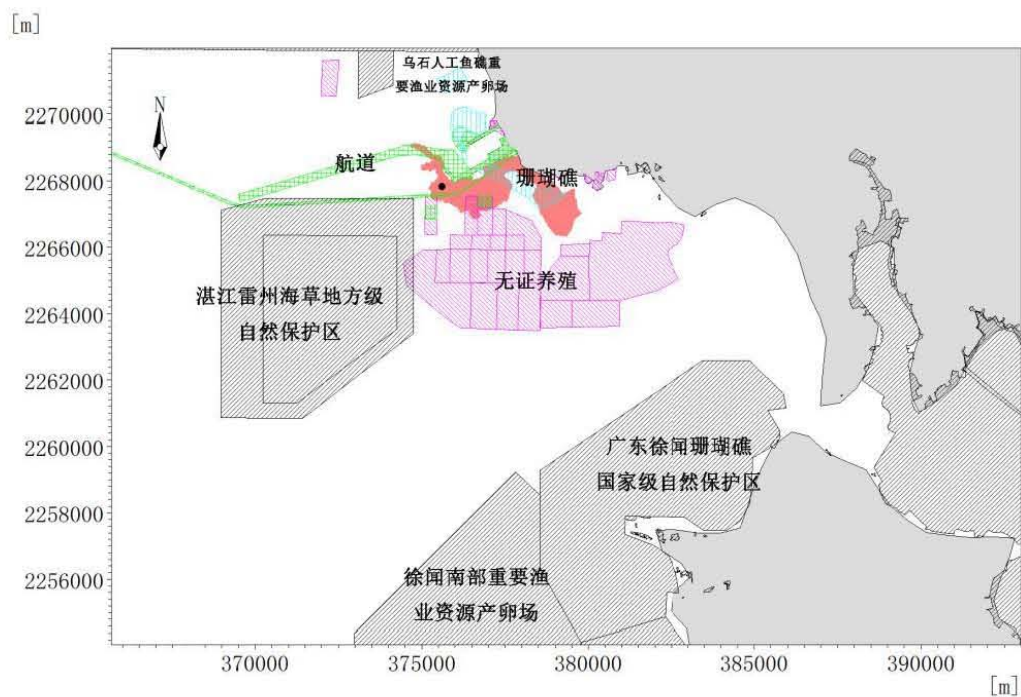
图 8.6.3-2 夏季主导风落潮 48 小时油膜扩散范围 (SW, 4.68m/s)
