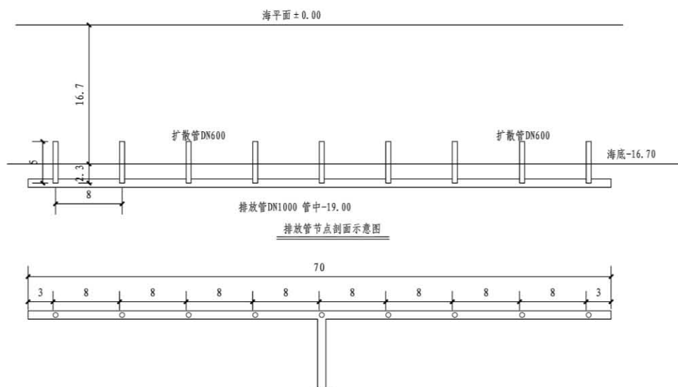
图 3.7.2-1 本项目扩散器结构断面图
