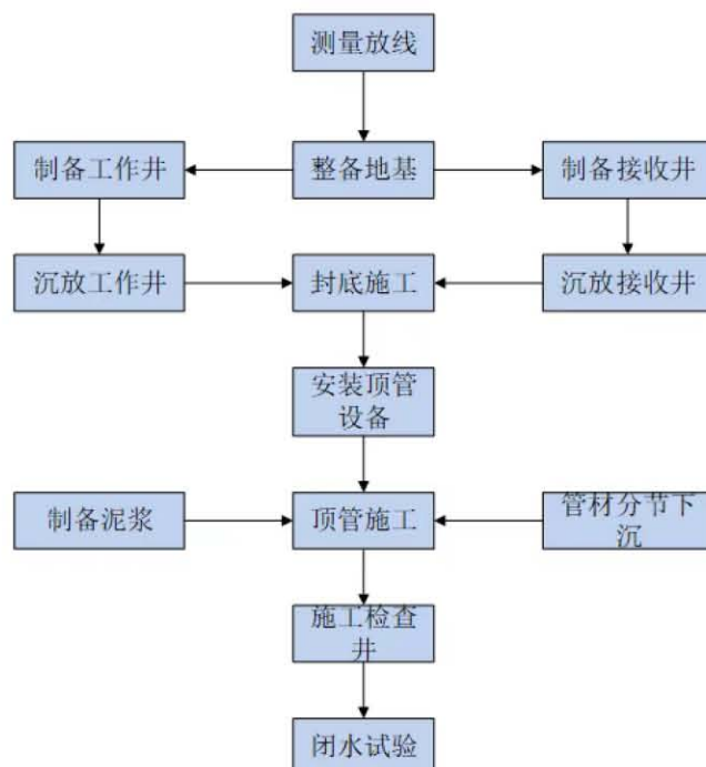
图 3.8.1-1 陆域管线顶管施工主要工艺流程图
