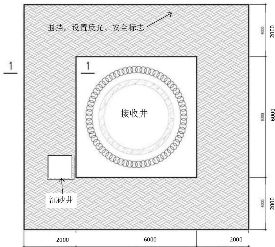
图 3.8.1-4 陆域顶管施工接收井施工场地平面布置图
