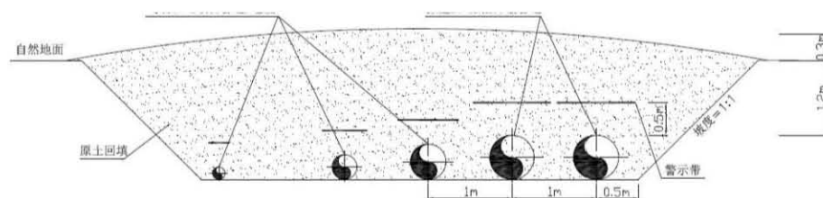
图 5.3.1-2 乌石油田群 5 条海缆同沟铺设断面图
