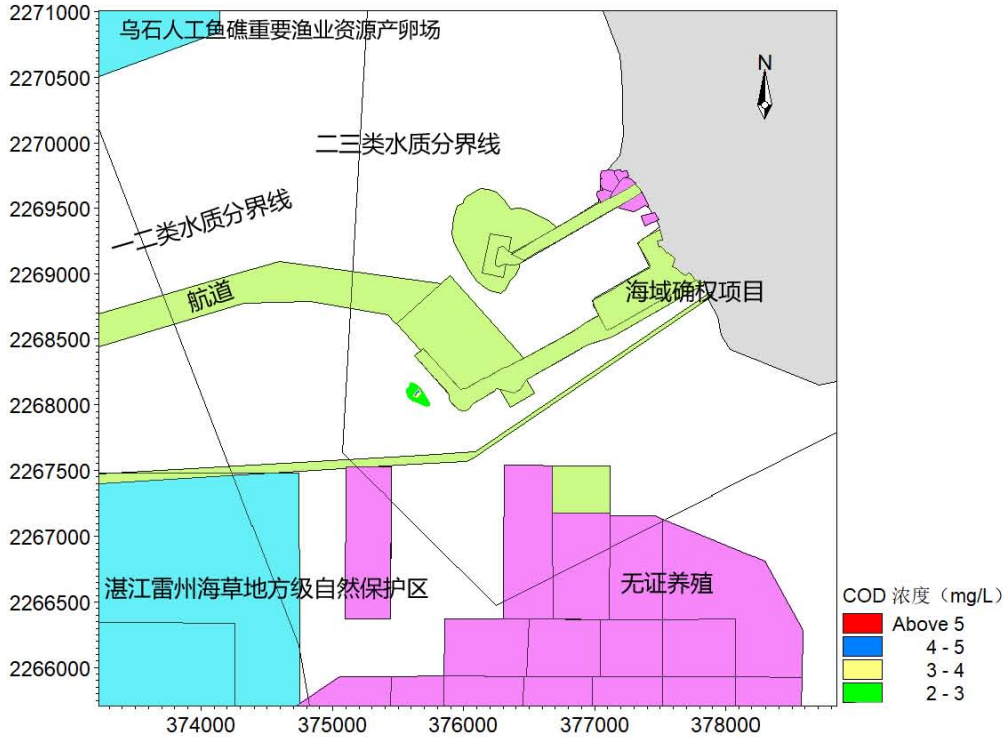
图 7.3.2-16 排污口中层 COD 扩散图
