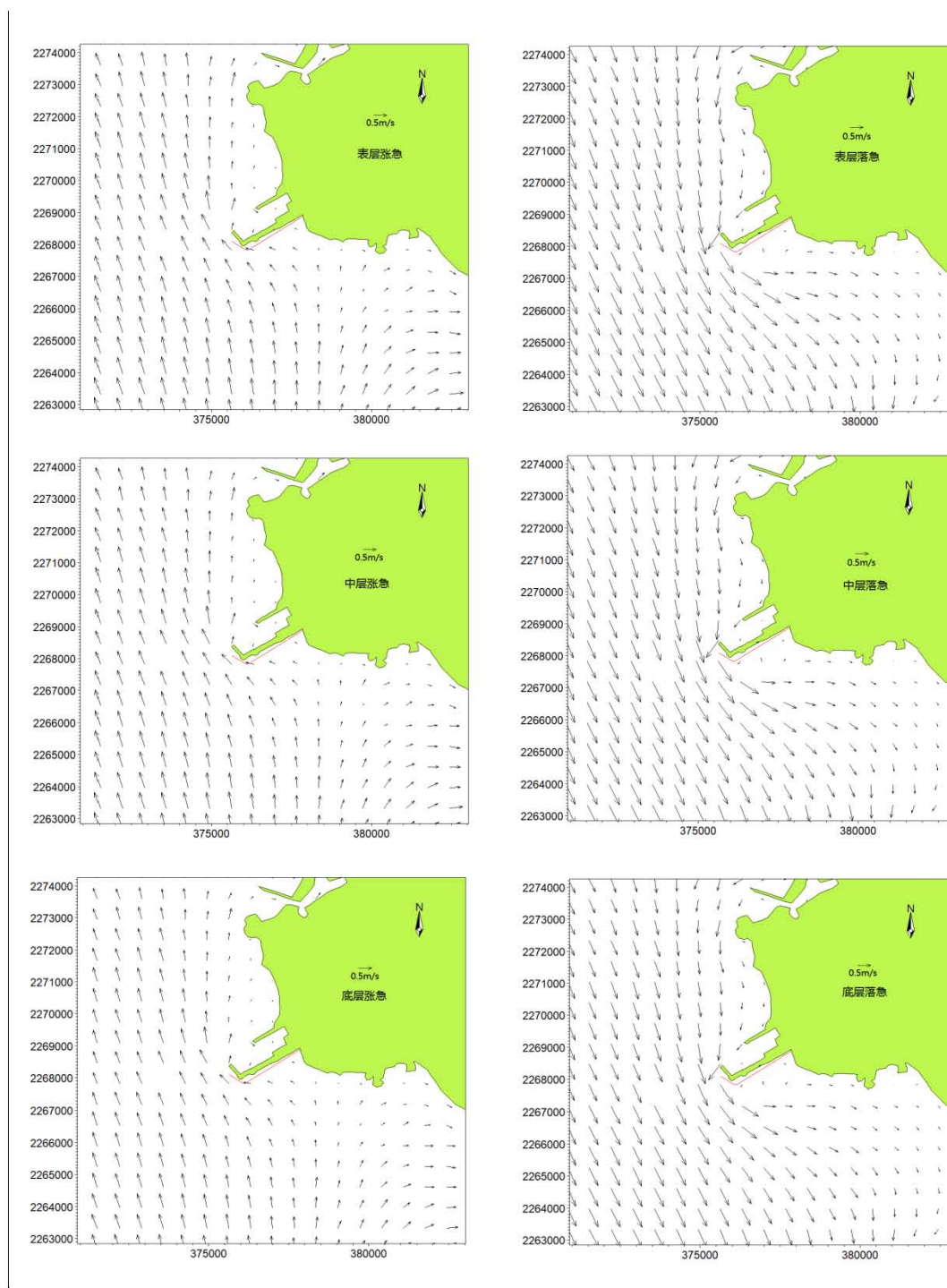
图 7.1.2-2 冬季表中底层涨落潮流场图（红线为管线）
