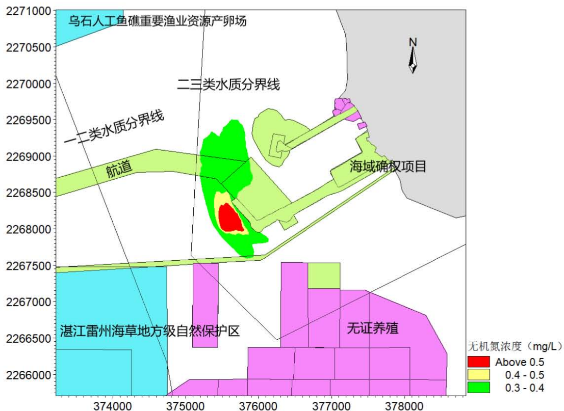
图 7.3.2-5 排污口中层无机氮扩散范围图
