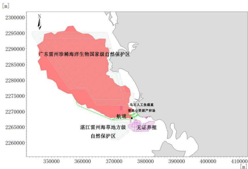
图 8.6.3-5 针对西北部敏感目标涨潮 48 小时油膜扩散范围 (SE, 13.8m/s)
