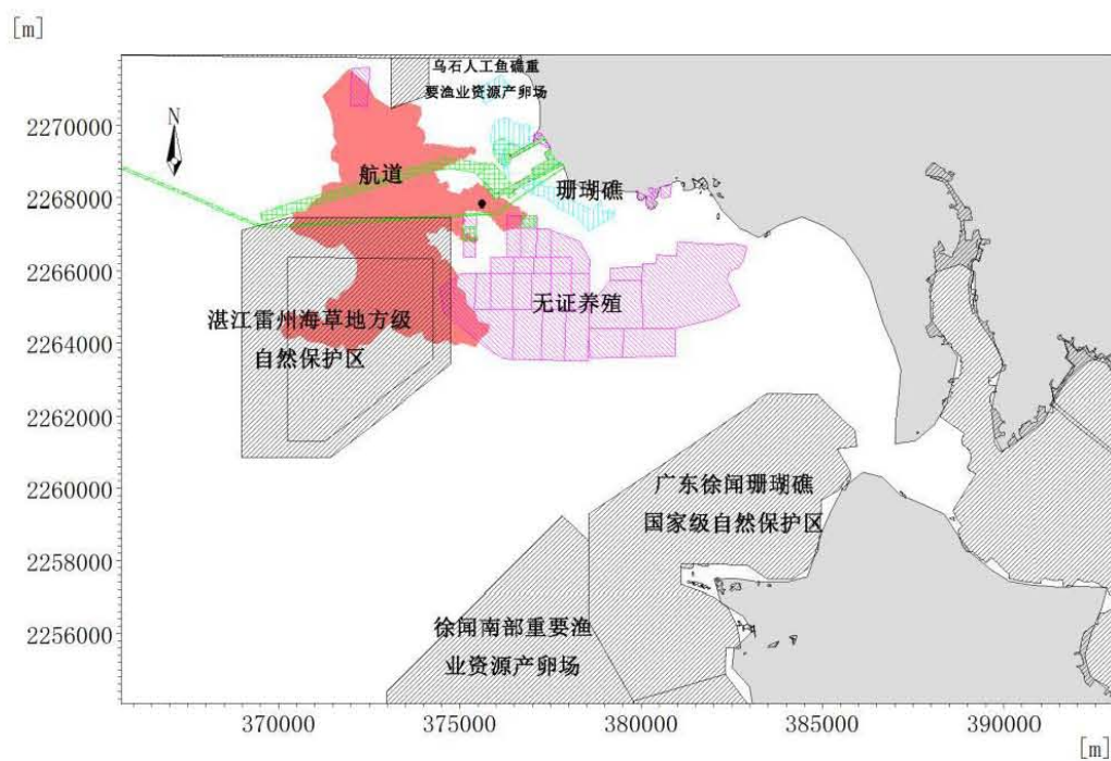
图 8.6.3-3 冬季主导风涨潮 48 小时油膜扩散范围 (NE, 5.03m/s)
