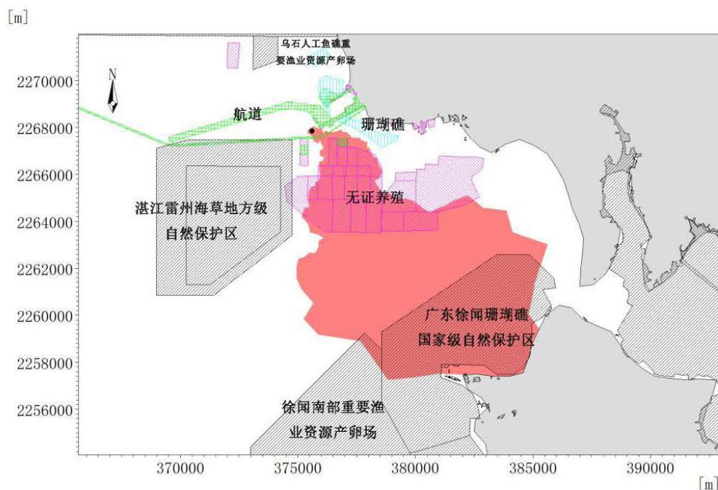
图 8.6.3-6 针对东南部敏感目标落潮 48 小时油膜扩散范围 (NW, 13.8m/s)
