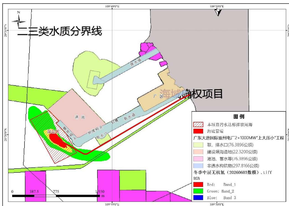
图 7.3.2-26a 排污混合区范围图
