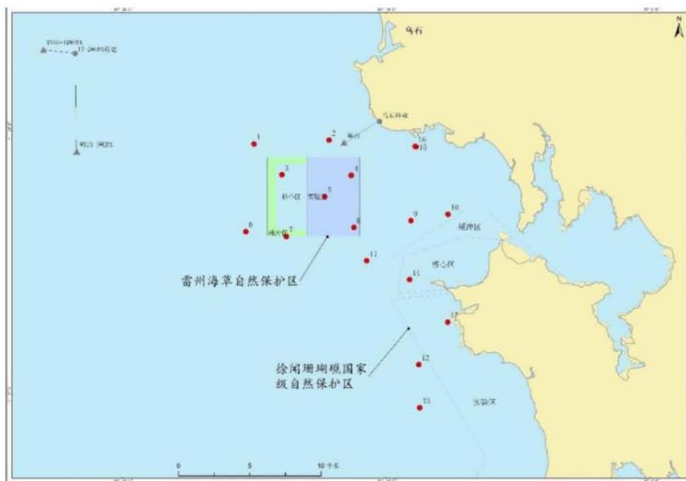
图 6.8.3-2 雷州海草自然保护区海草床保护生物监测站位图（2020 年）
