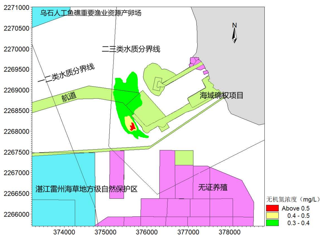
图 11.1.1-4 排污口底层无机氮扩散范围与生态保护红线叠置图
