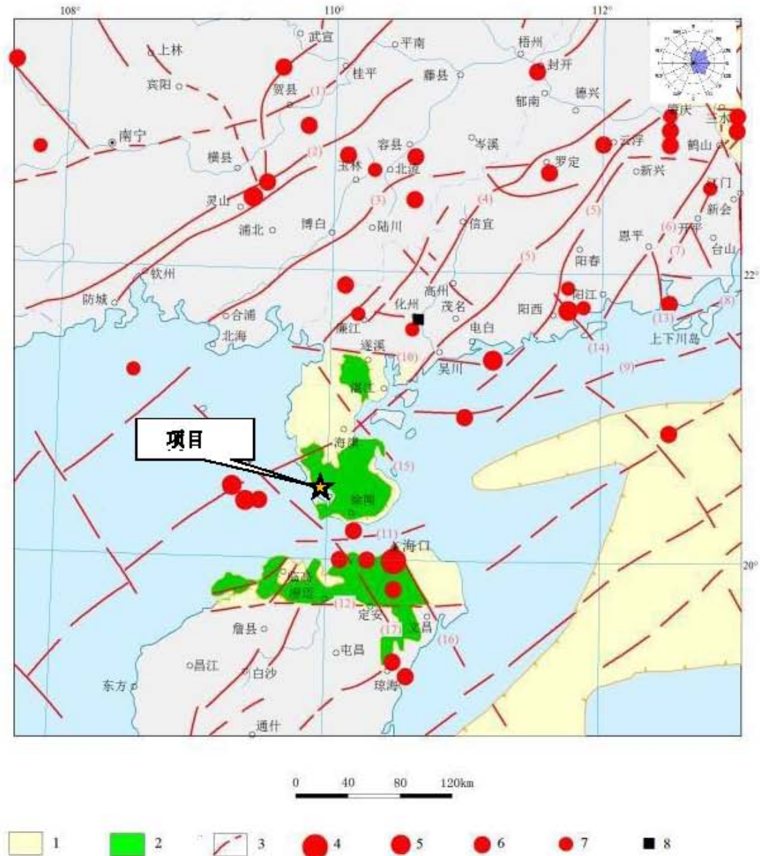
图 5.13-1 区域主要断裂构造与地震分布
