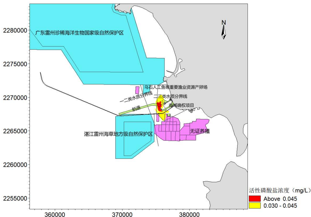
图 7.3.2-34 排污口事故工况表层活性磷酸盐扩散范围图
