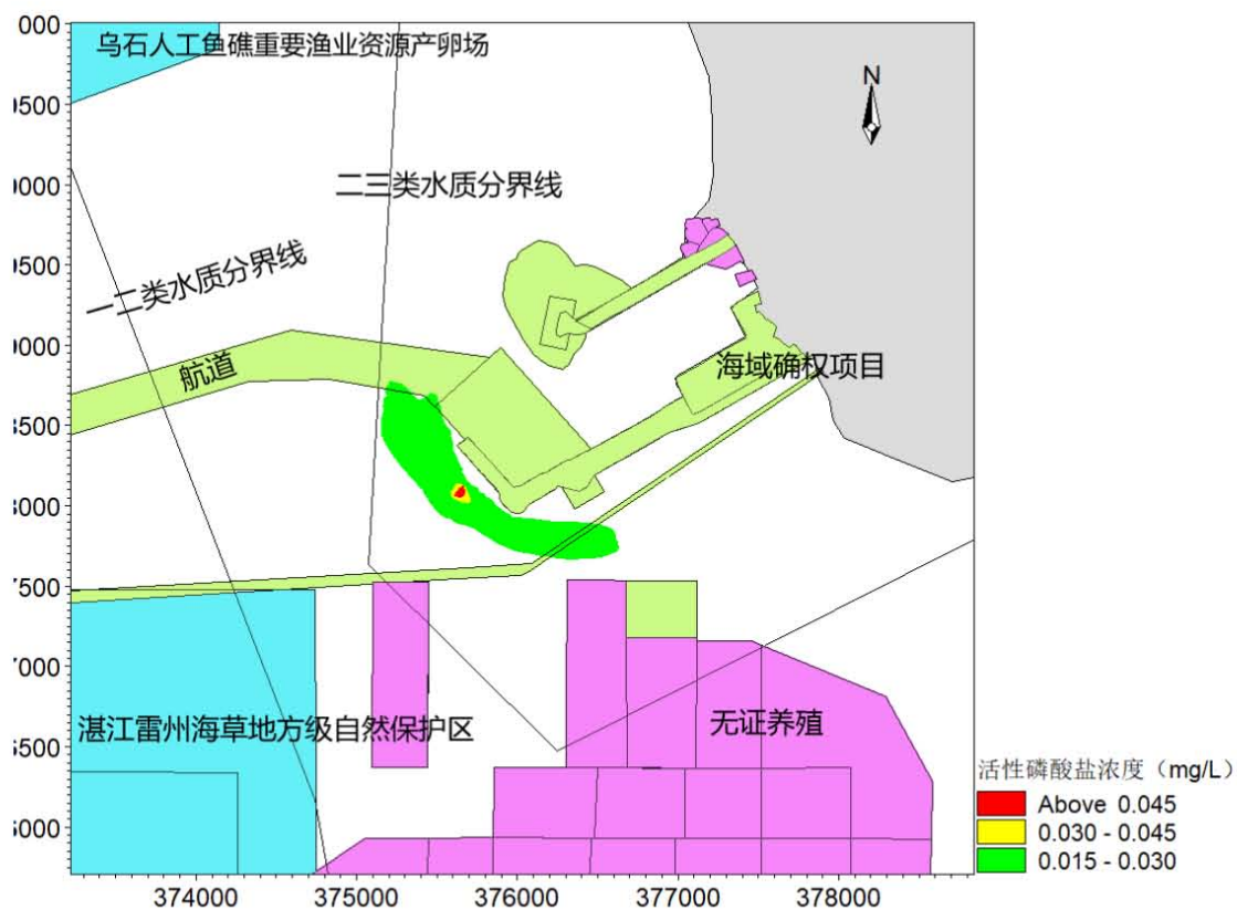
图 7.3.2-21 排污口中层活性磷酸盐扩散范围图
