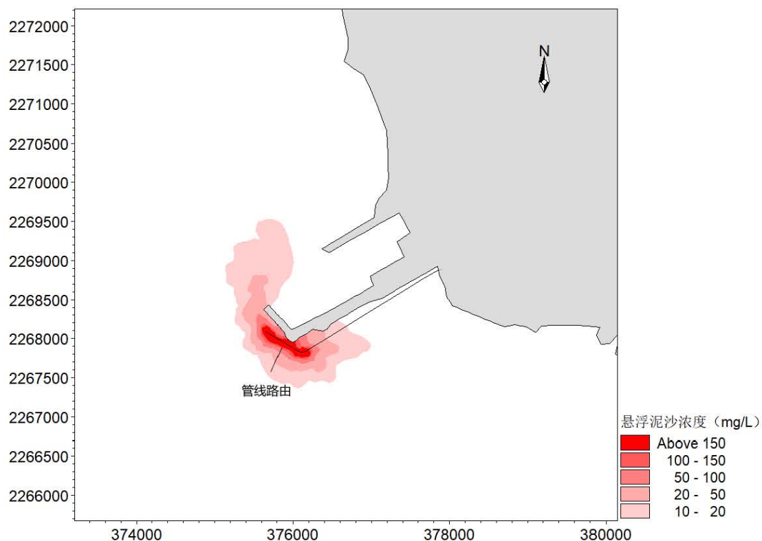
图 7.3.1-2 工程施工造成的底层悬沙增量浓度
