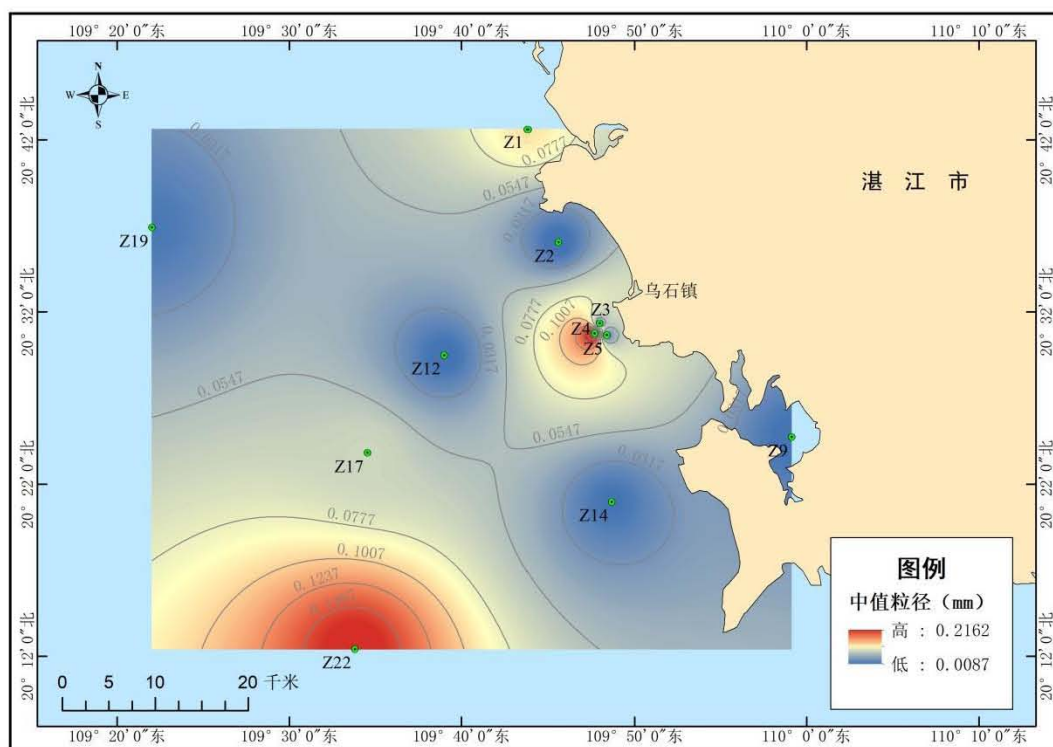
图 6.2-3 湛江乌石海域表层沉积物中值粒径平面分布（2023 年春季）
