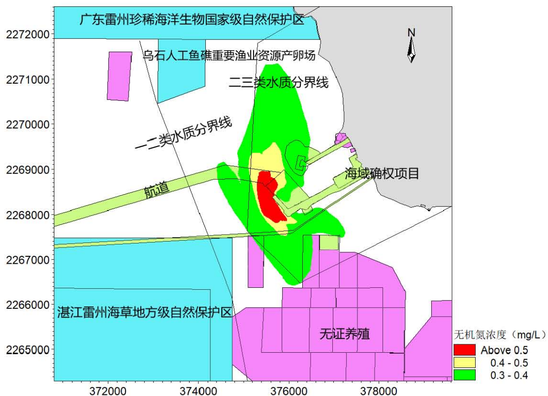
图 7.3.2-30 排污口事故工况中层无机氮扩散范围图
