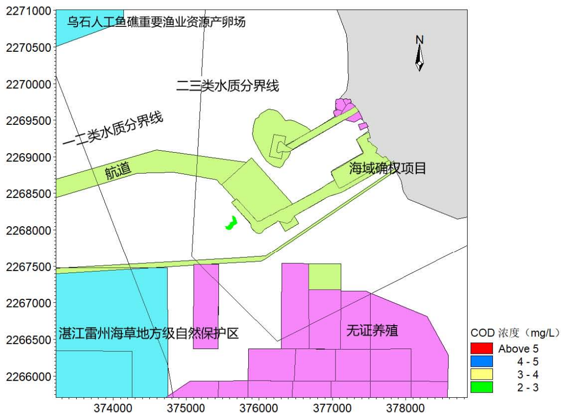
图 7.3.2-2 排污口表层 COD 扩散范围图
