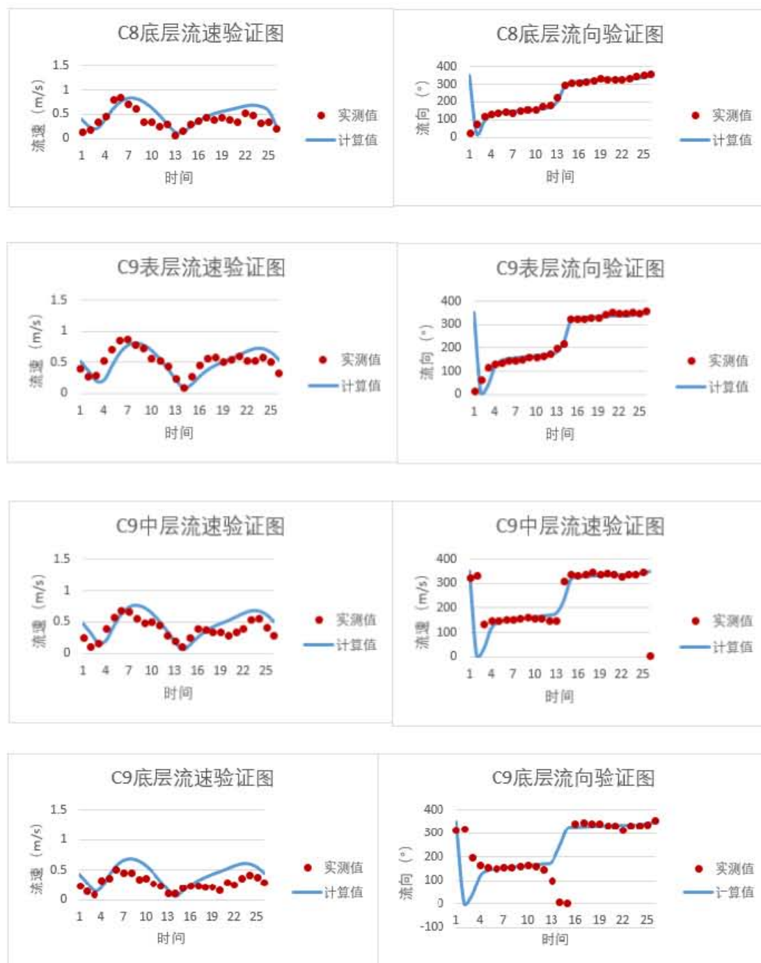
图 7.1.1-4 夏季大潮各层流速流向验证图
