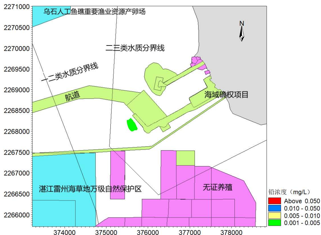
图 7.3.2-14 排污口底层铅扩散范围图
