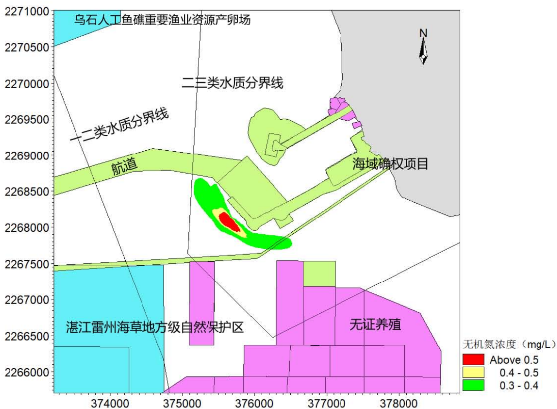
图 7.3.2-18 排污口中层无机氮扩散范围图
