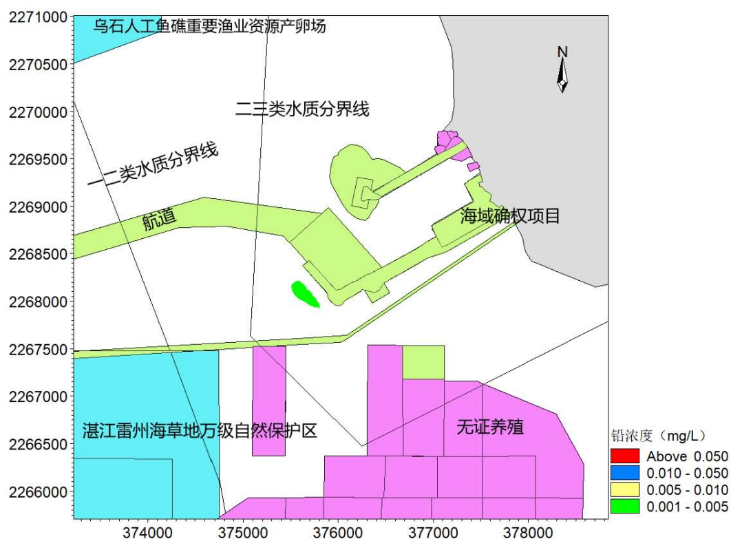
图 7.3.2-23 排污口中层铅扩散范围图
