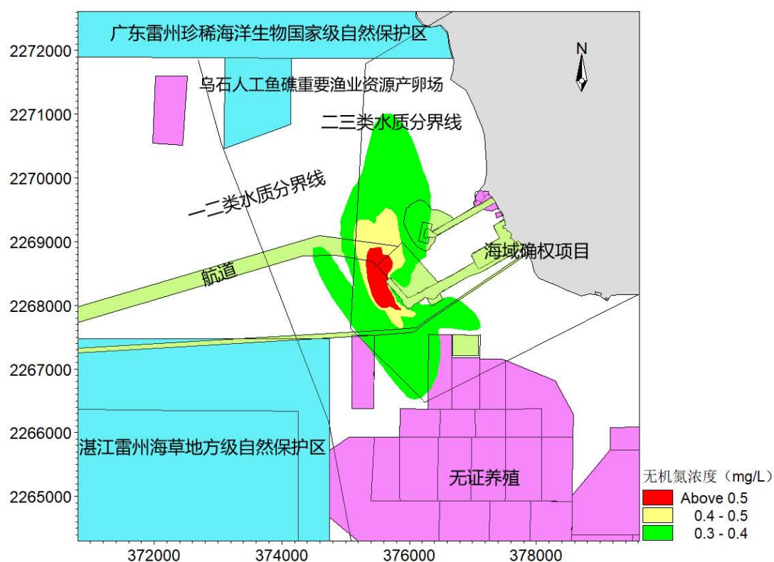
图 7.3.2-31 排污口事故工况底层无机氮扩散范围图
