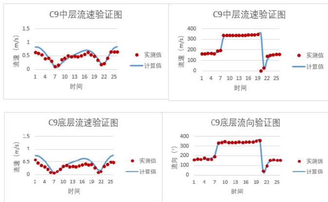
图 7.1.1-6 冬季大潮各层流速流向验证图
