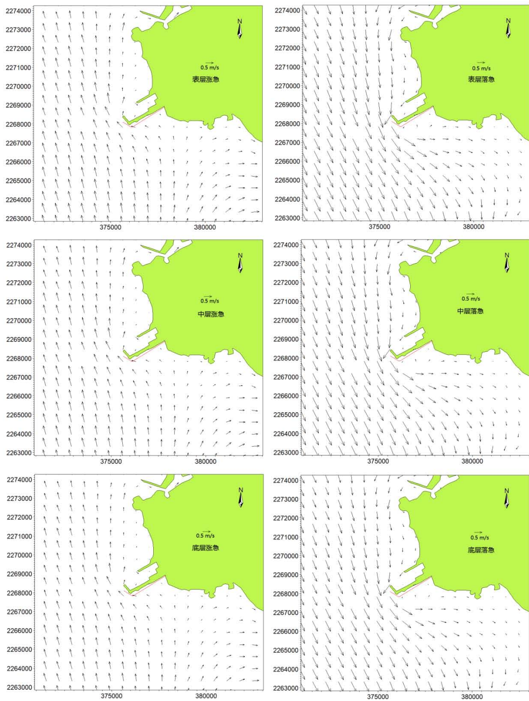
图 7.1.2-1 夏季表中底层涨落潮流场图（左边为涨潮，右边为落潮，红线为管线）
