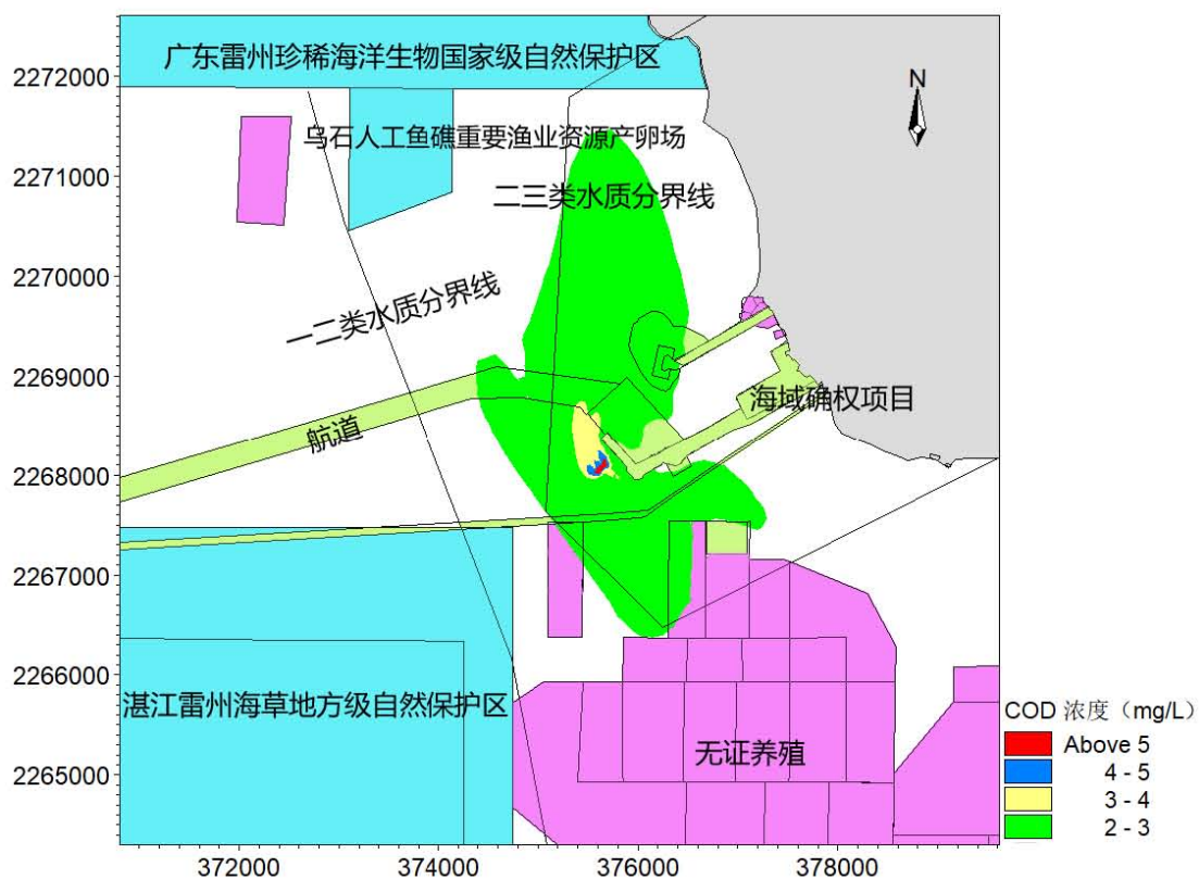
图 7.3.2-26 排污口事故工况表层 COD 扩散范围图
