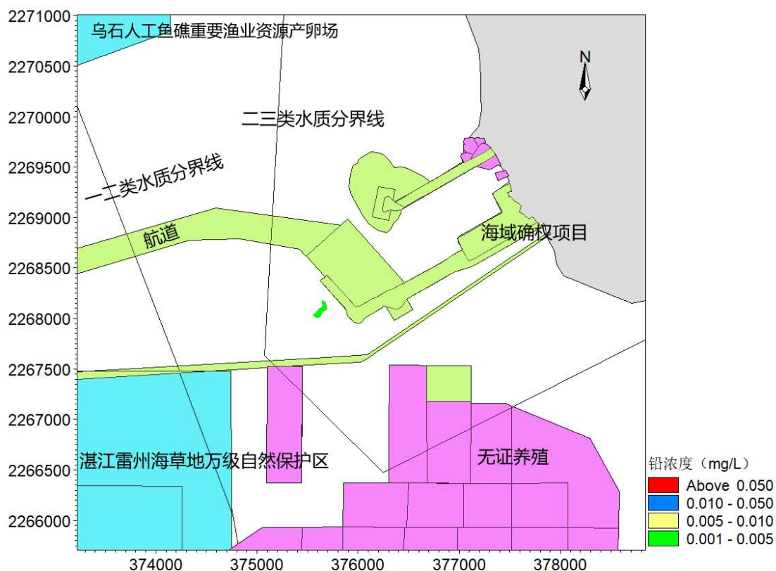
图 7.3.2-12 排污口表层铅扩散范围图
