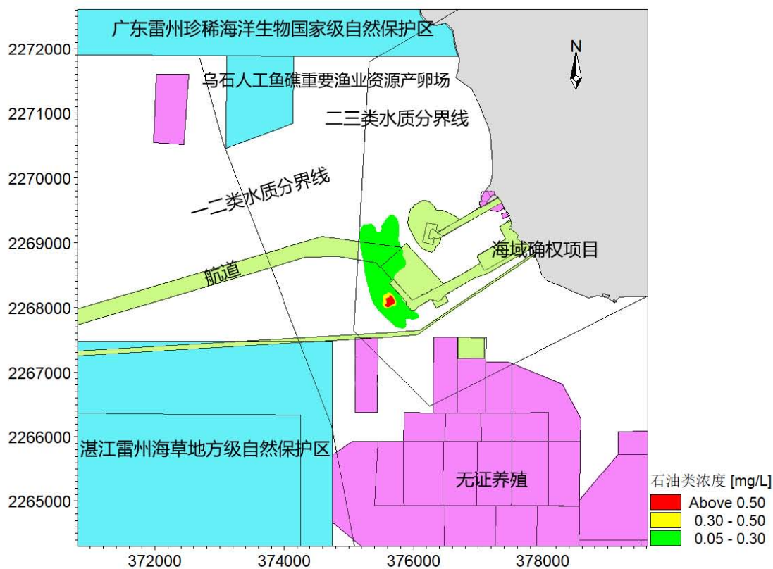
图 7.3.2-33 排污口事故工况中层石油类扩散范围图
