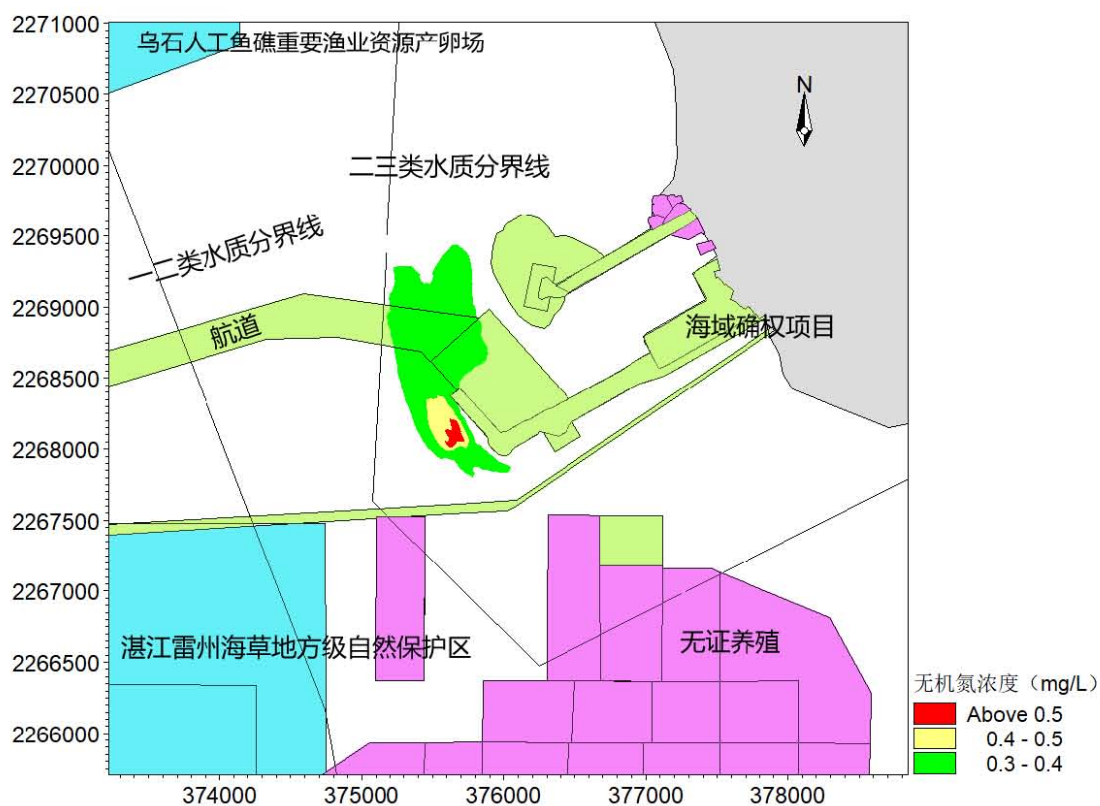
图 7.3.2-6 排污口底层无机氮扩散范围图
