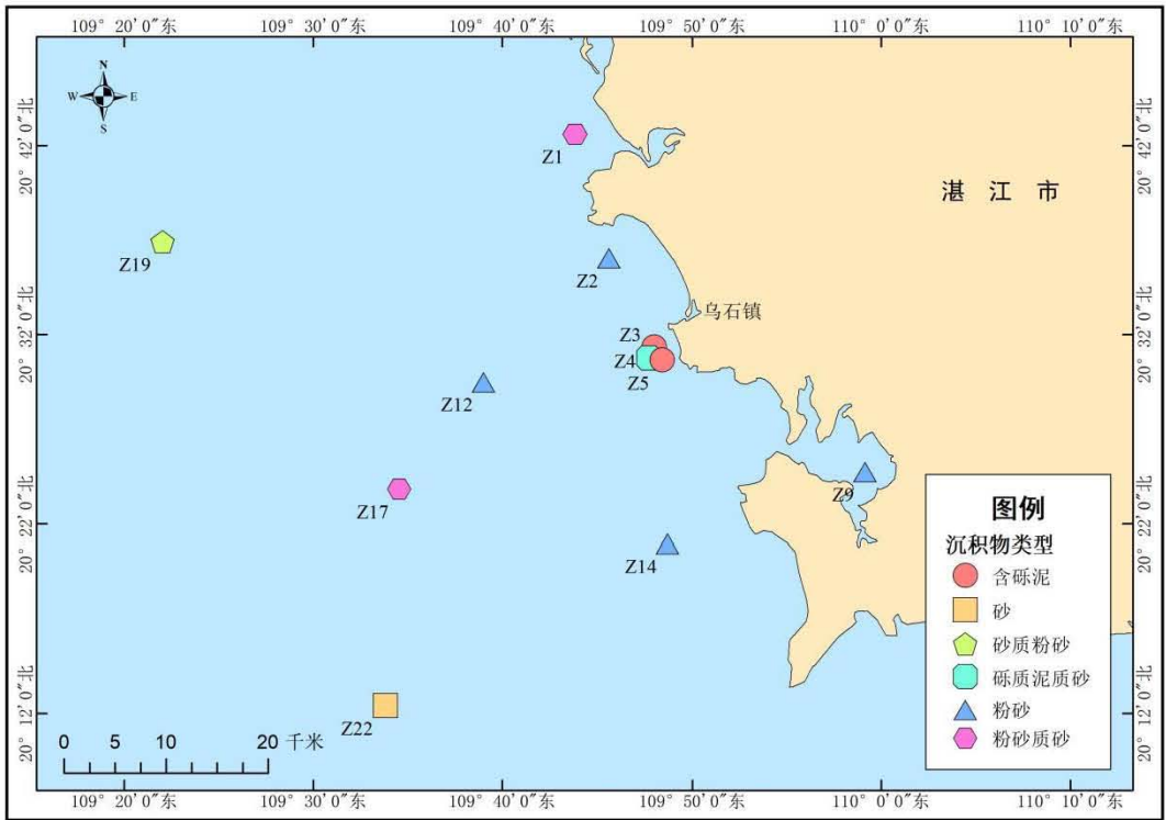
图 6.2-2 湛江乌石海域表层沉积物类型平面分布（2023 年春季）
