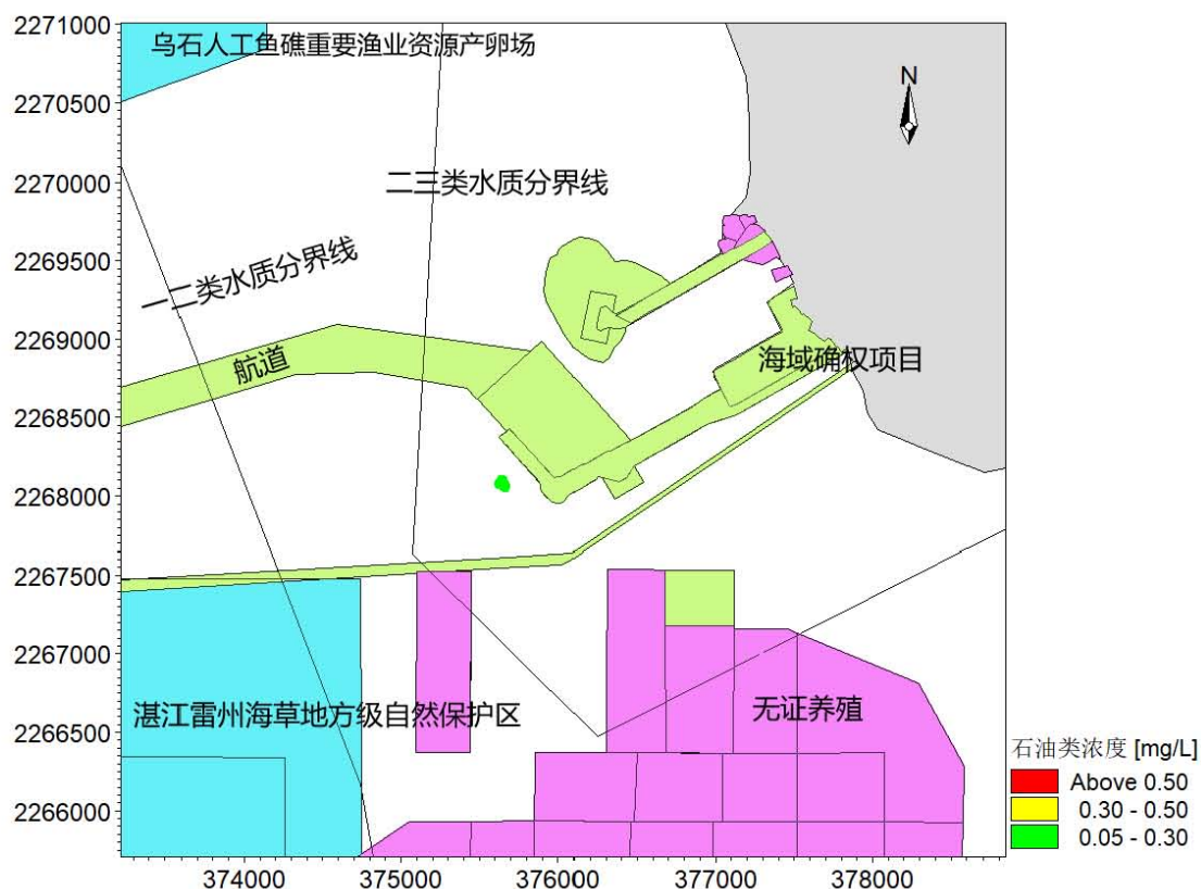
图 7.3.2-20 排污口中层石油类扩散范围图
