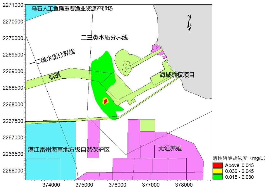
图 7.3.2-9 排污口中层活性磷酸盐扩散范围图
