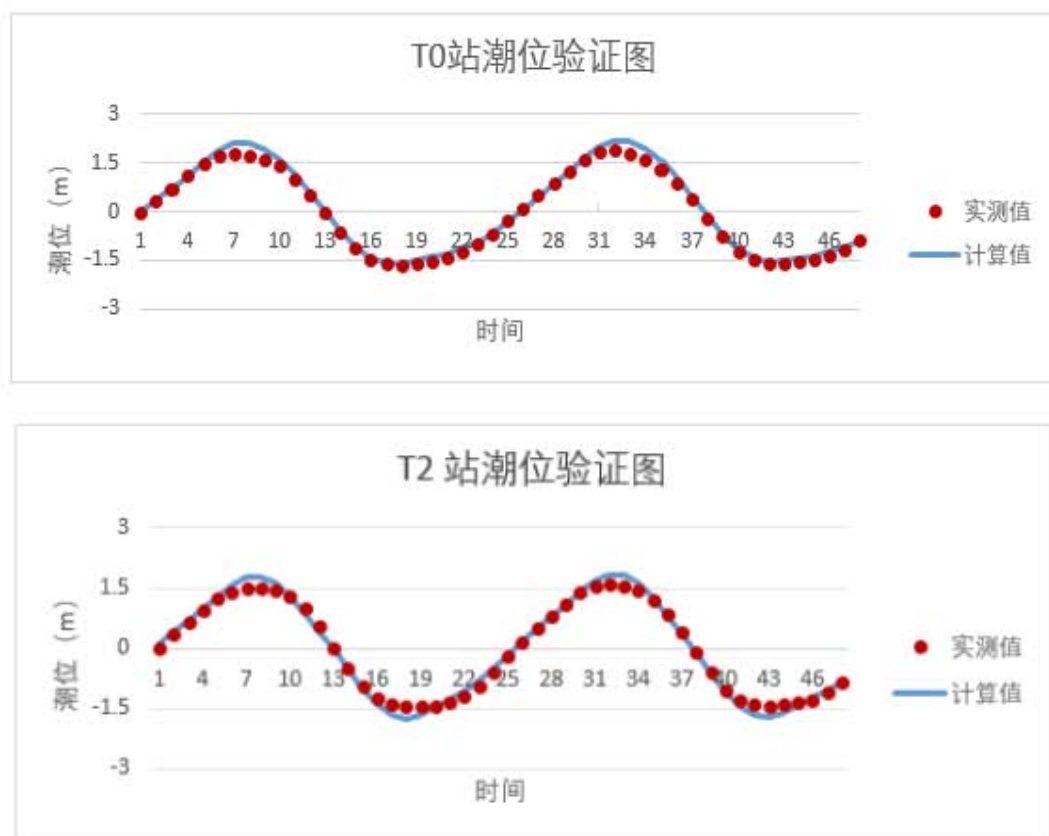
图 7.1.1-5 冬季潮位验证图
