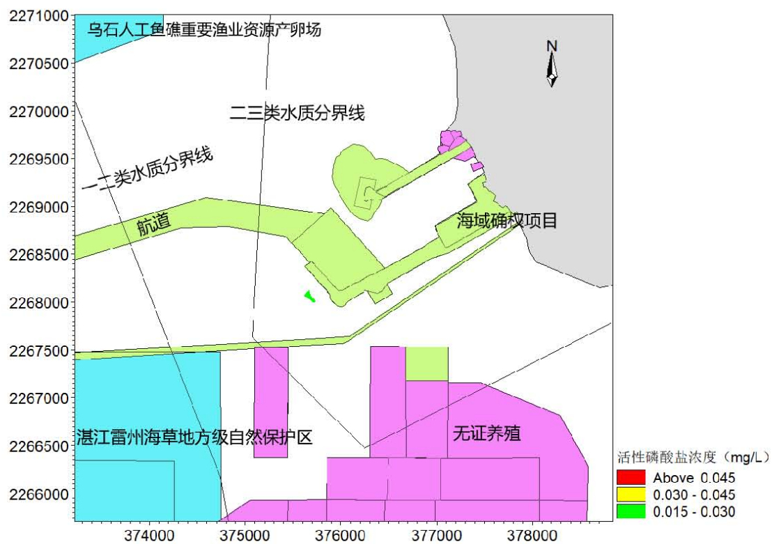
图 7.3.2-22 排污口底层活性磷酸盐扩散范围图
