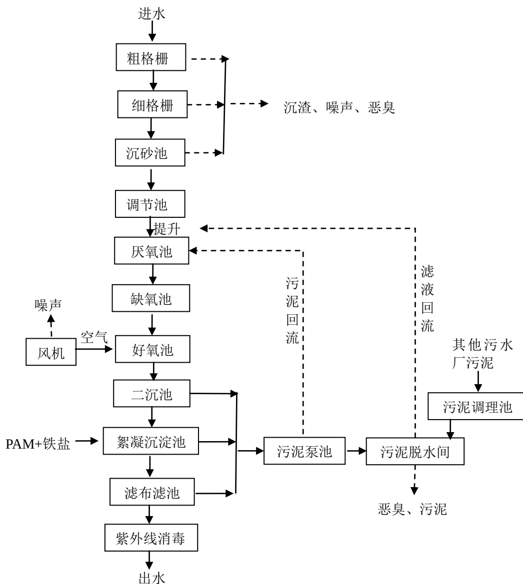
图 4 项目营运期污水处理工艺流程及产污节点示意图
