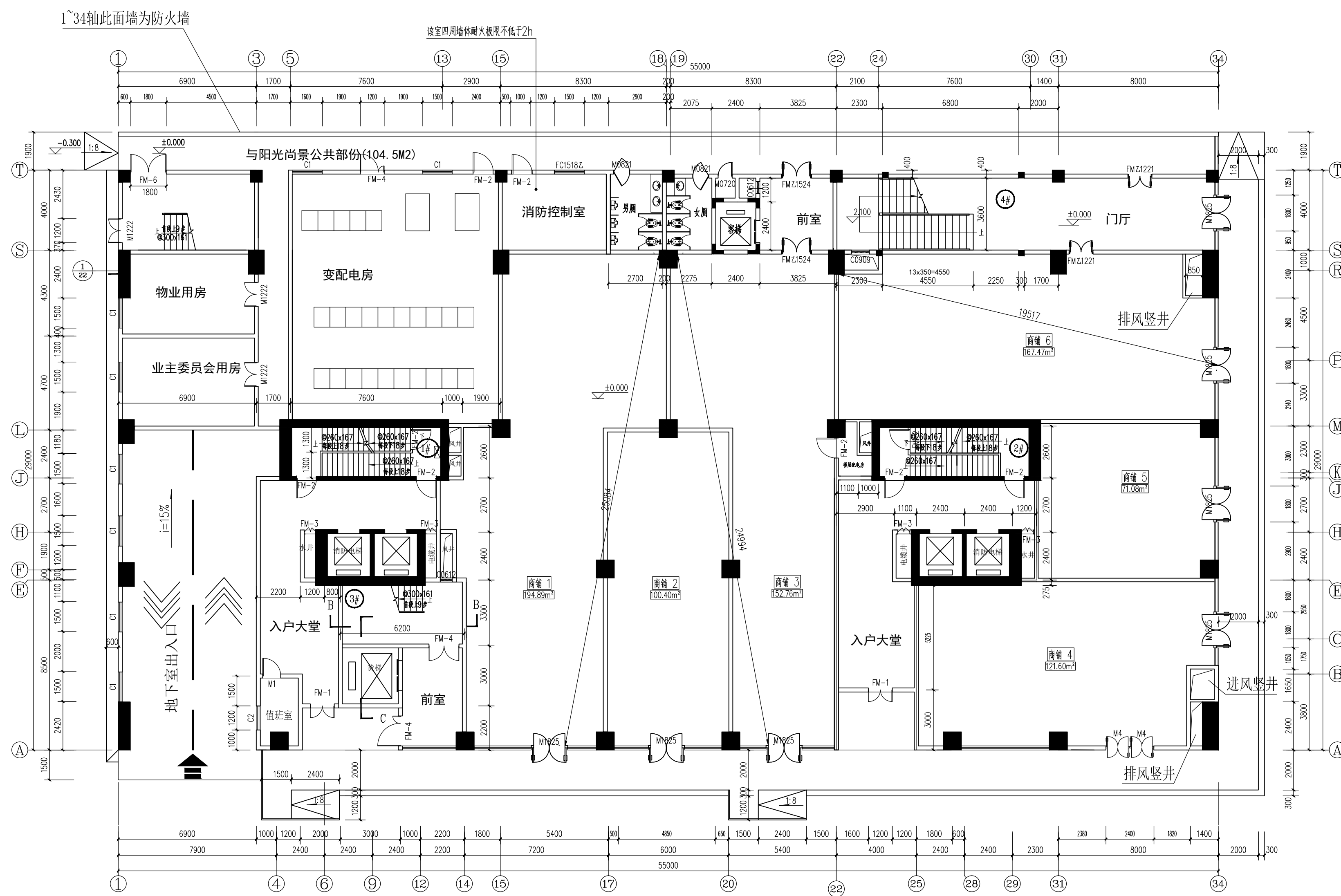
商场底层平面图 1:100
