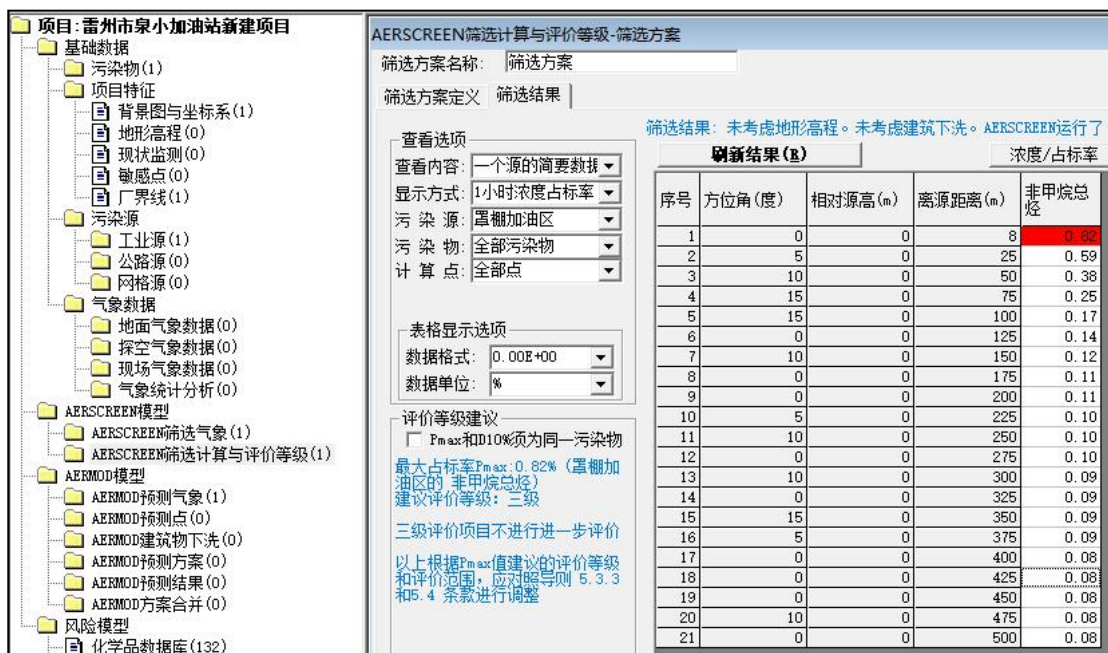
图8 罩棚加油区(多边形面源)最大占标率 P_{max} 估算结果
