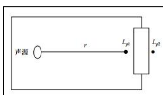
图 9 室内声源等效为室外声源图
