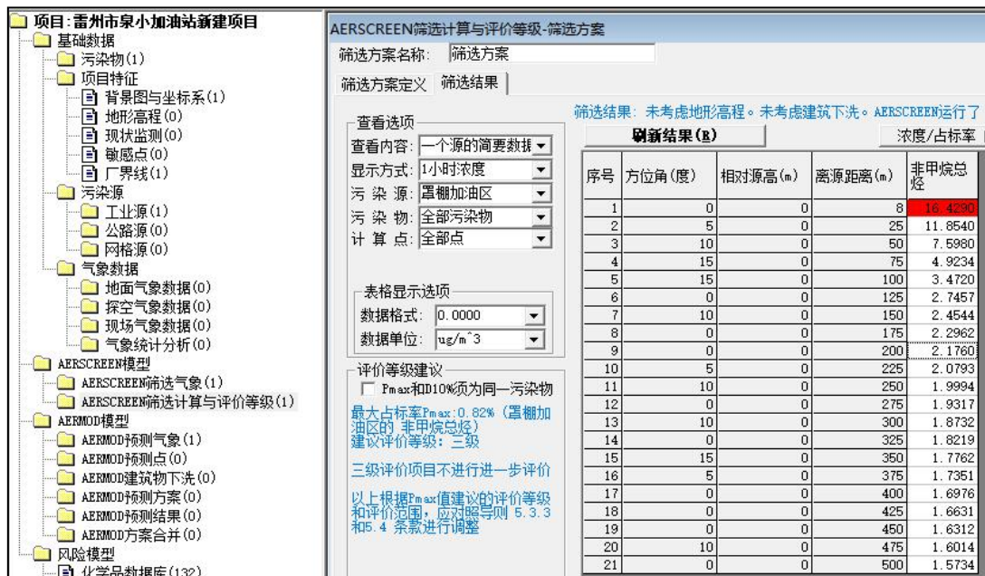
图7 罩棚加油区(多边形面源)最大地面空气质量浓度 C_{max} 估算结果
