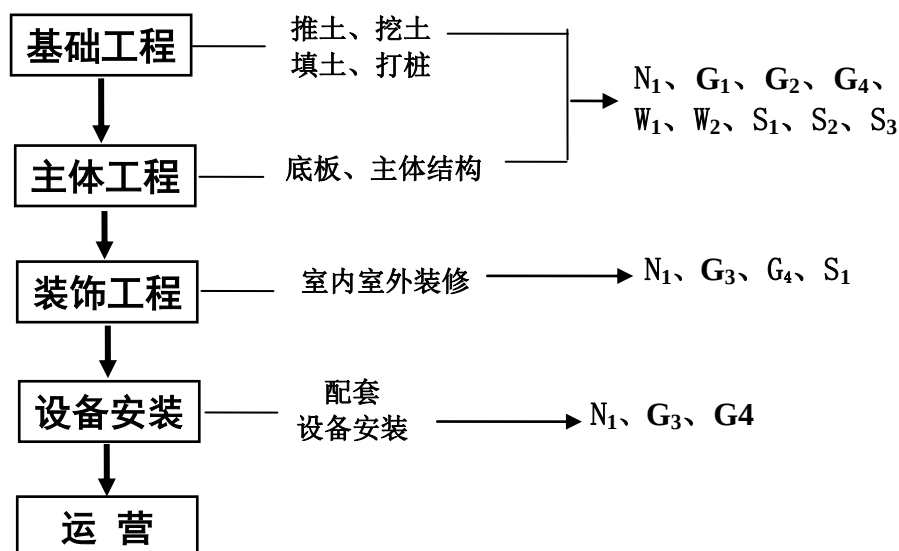
图 5-1 施工阶段生产工艺流程及产污示意图
