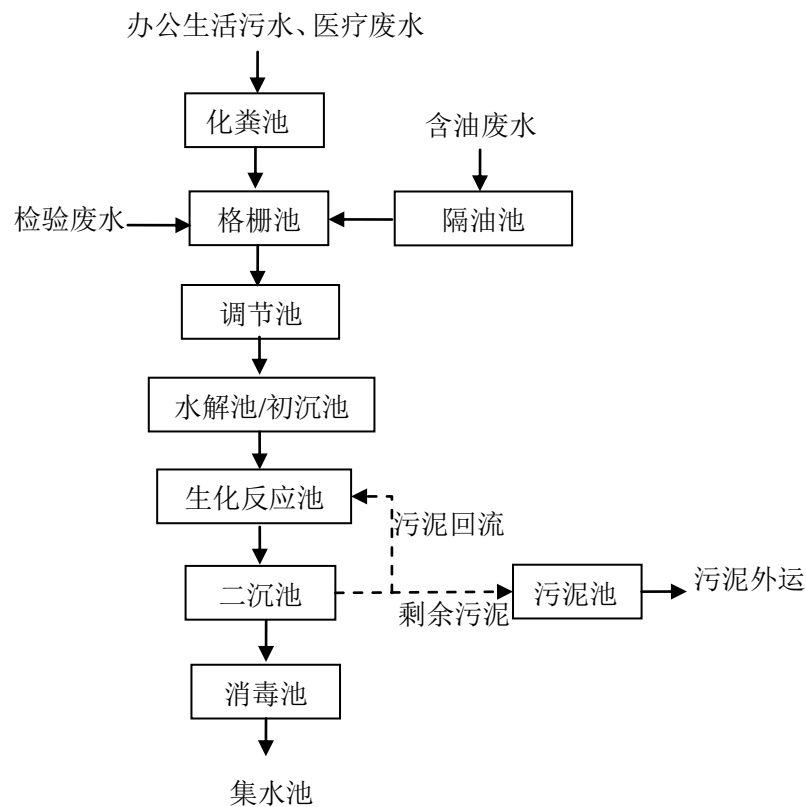
图 6-1 院内自建污水处理工艺流程图
