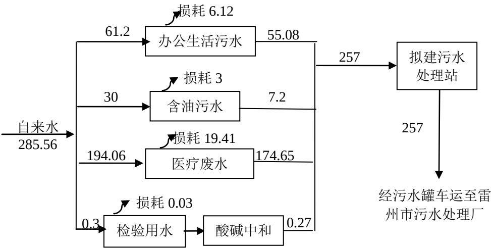
图 5-3 项目日水平衡图（单位：t/d）
