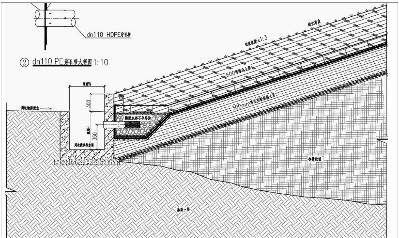
图1 方案剖面图
