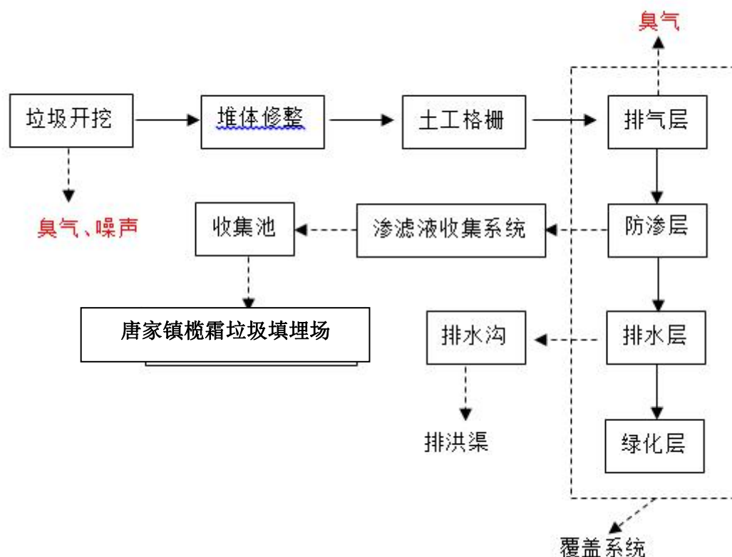
图 5-1 封场施工期工艺流程图及产污环节图
