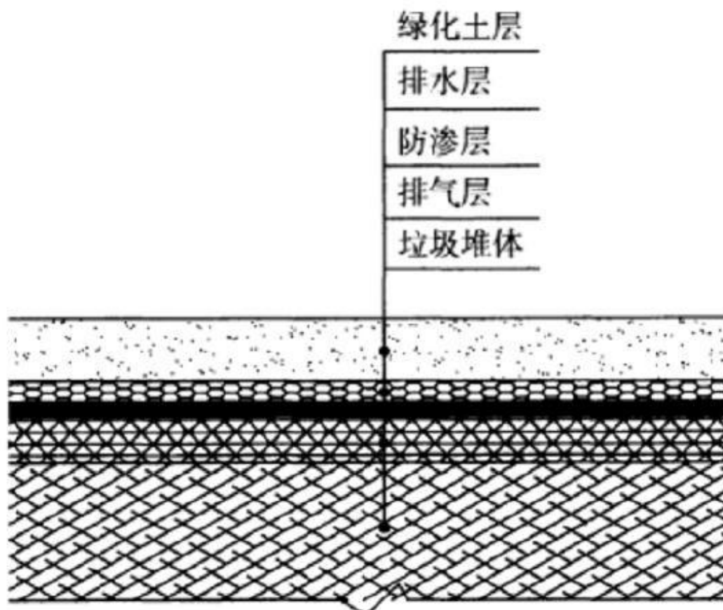
图 2 覆盖系统结构图
