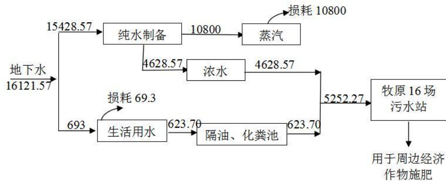
图 2-2 项目运营期给排水年平衡图 (t/a)
