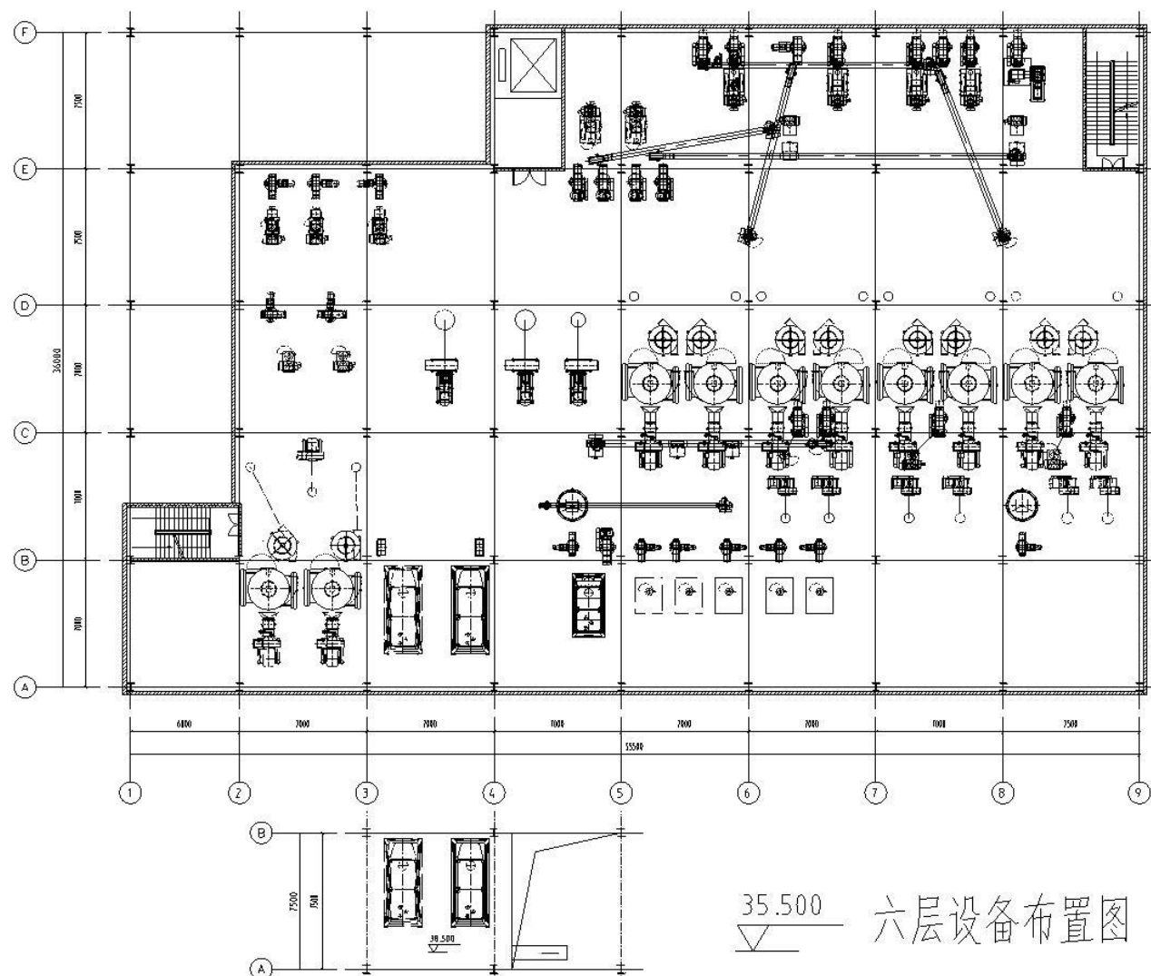
附图5 生产车间（生产区）平面布置图
