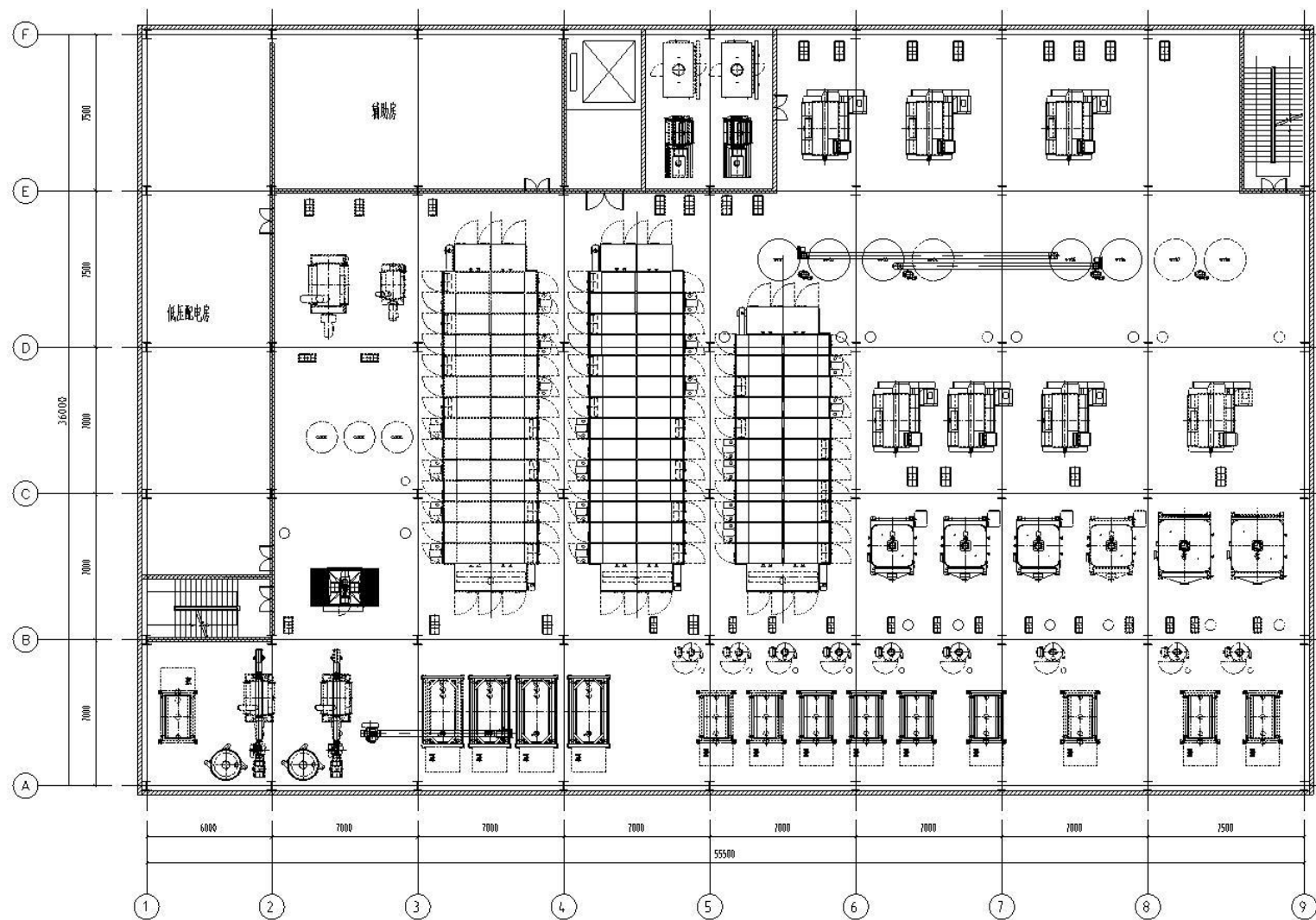
7.000 二层设备布置图
