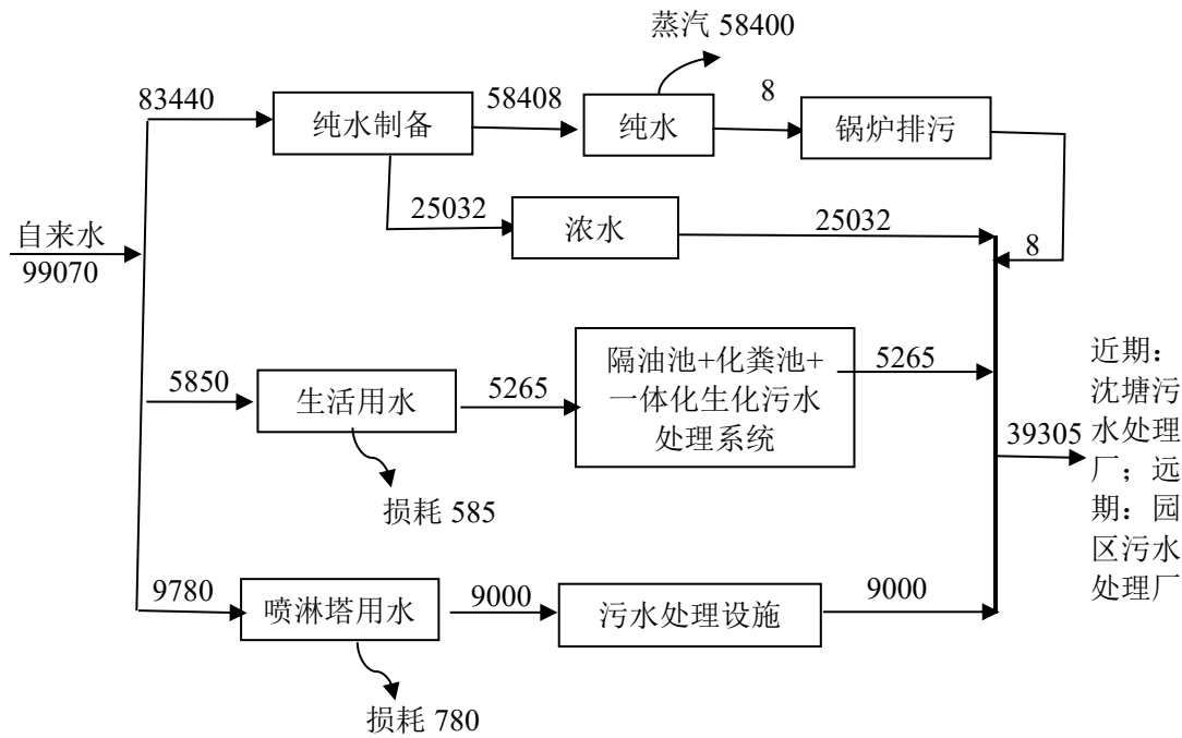
图 2-2 项目运营期给排水年平衡图（t/a）
