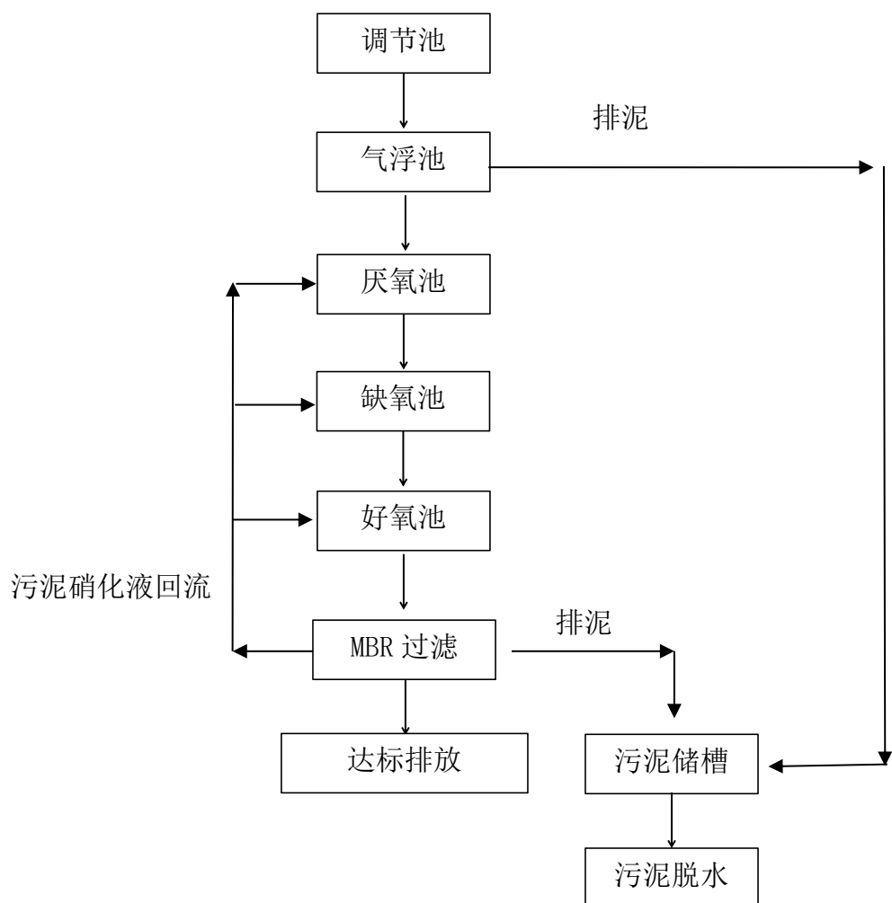
图 4-1 项目污水处理设施废水处理工艺流程图
