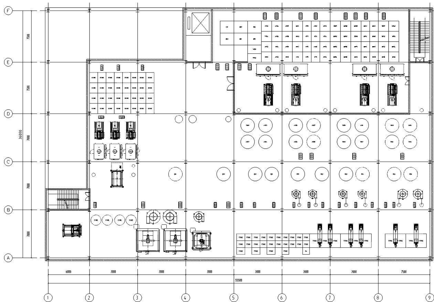
22.500 四層設備布置圖
