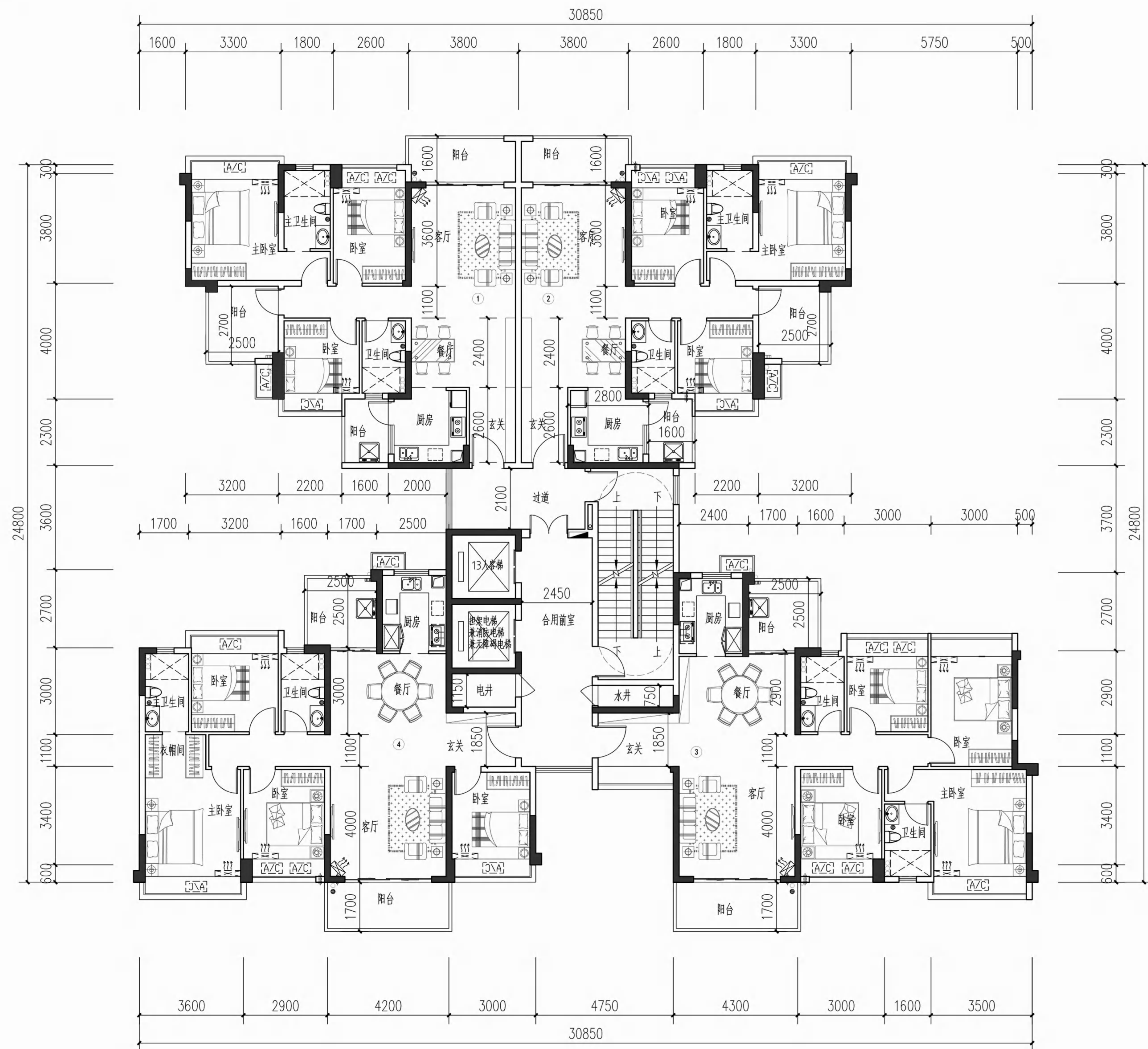
标准层平面图图
