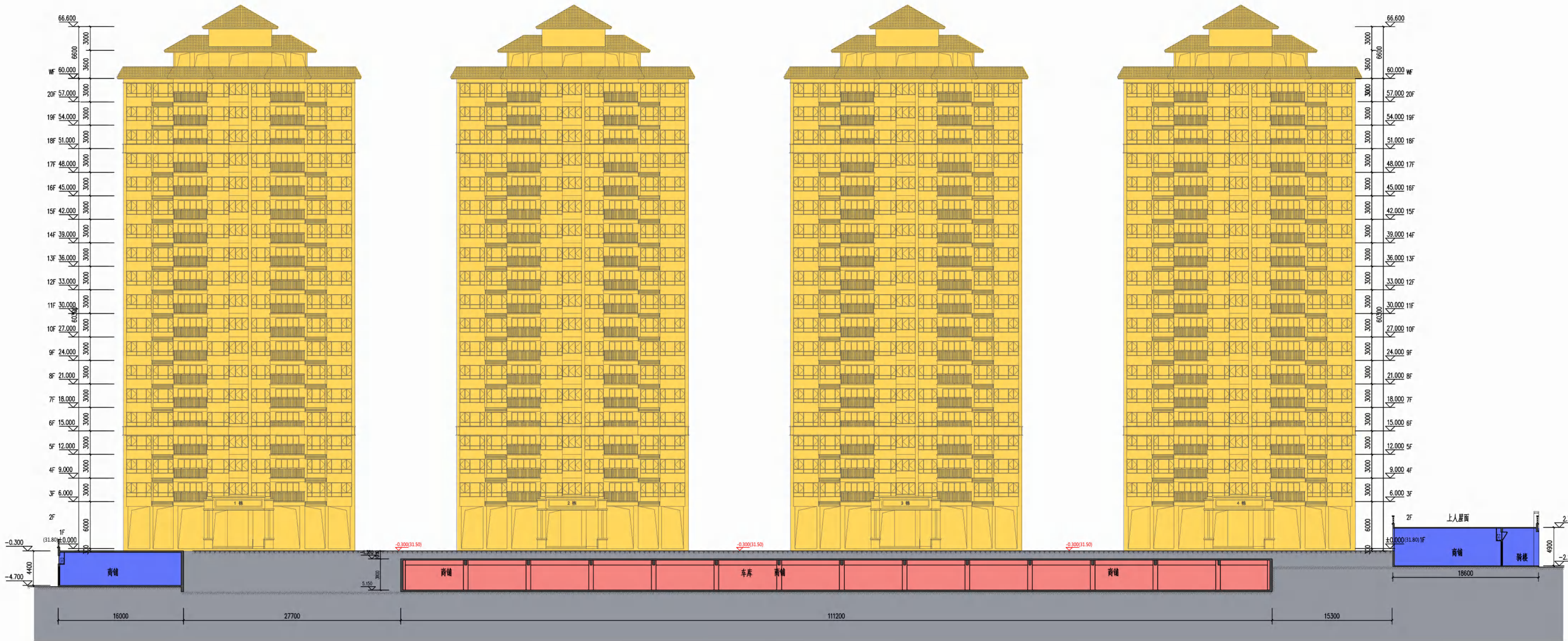
2-2剖面示意图
