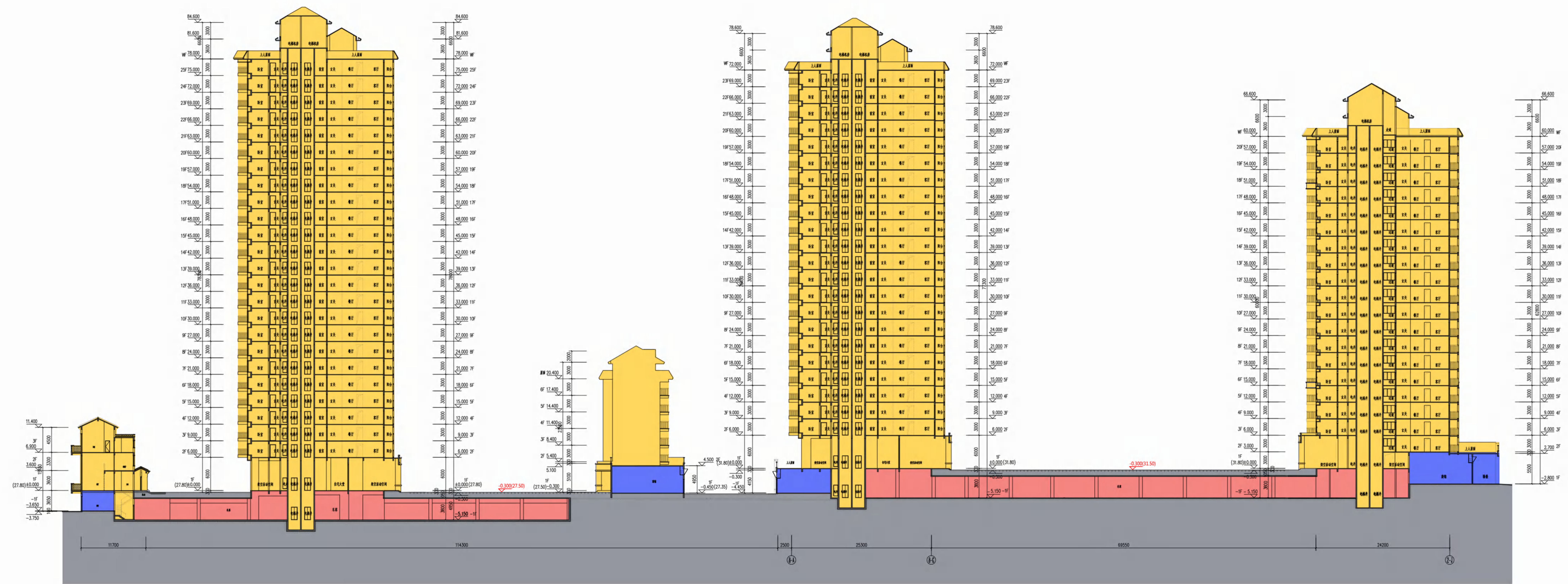
1-1剖面示意图
