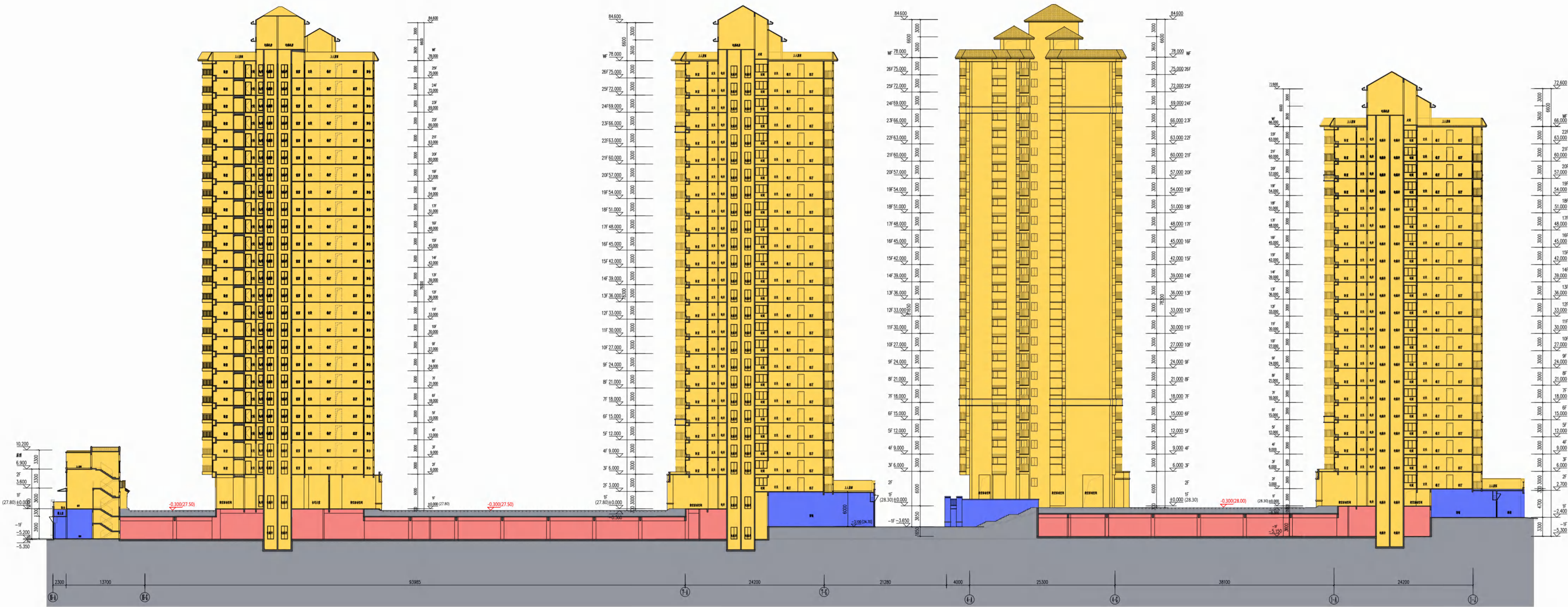
1-1剖面示意图
