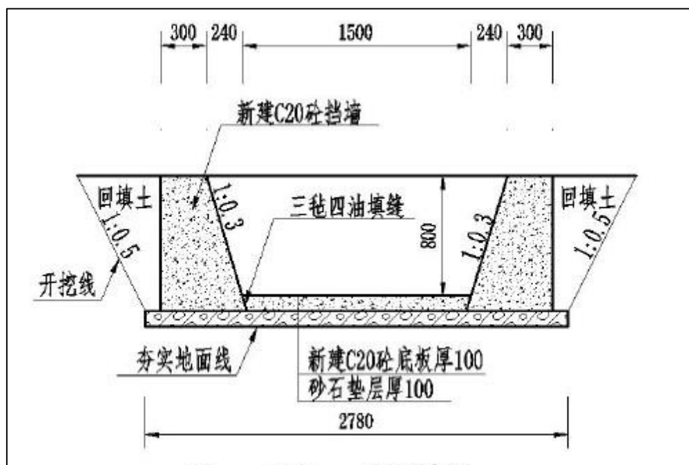
图 1 渠道横断面型式图
